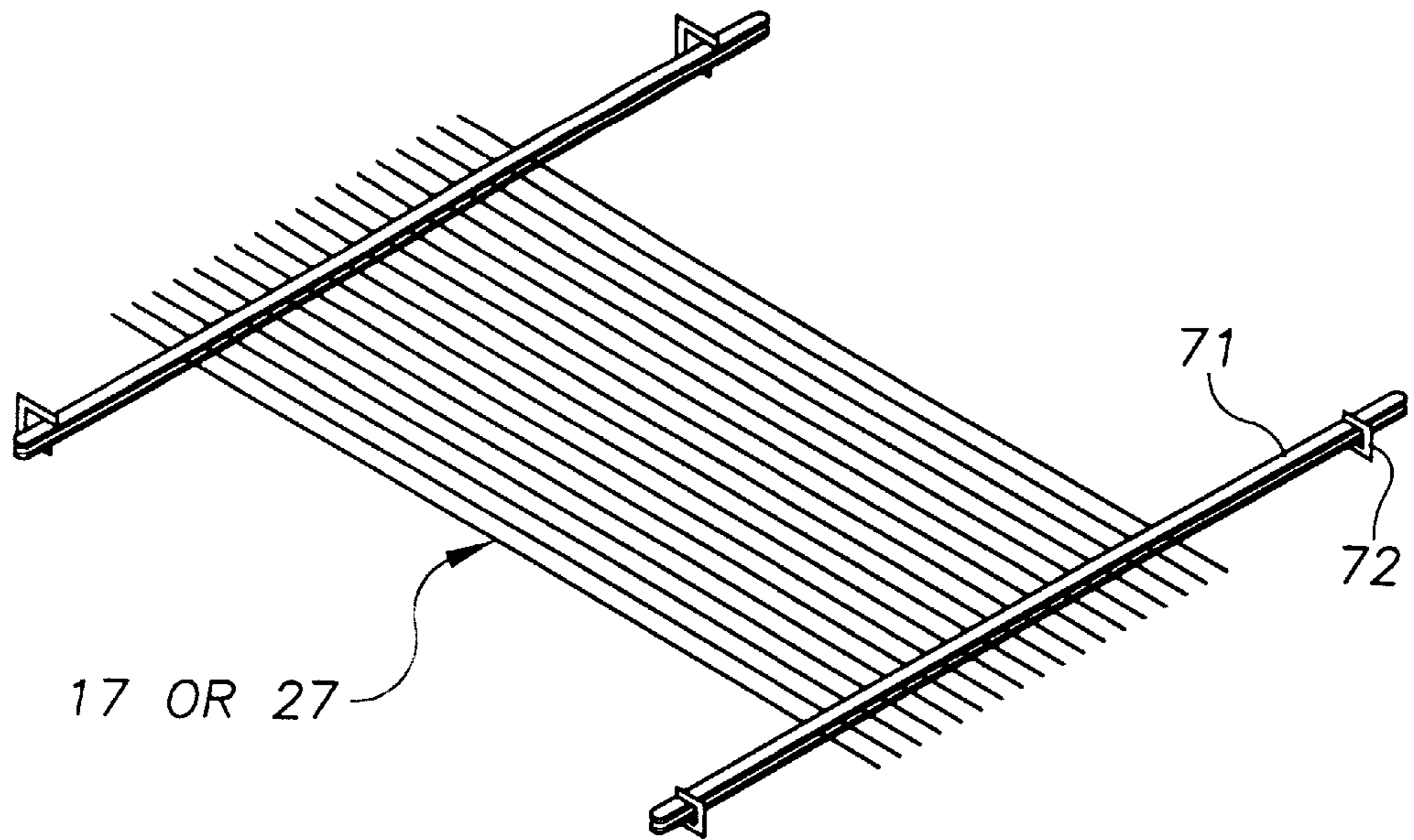
FIG. 26D
