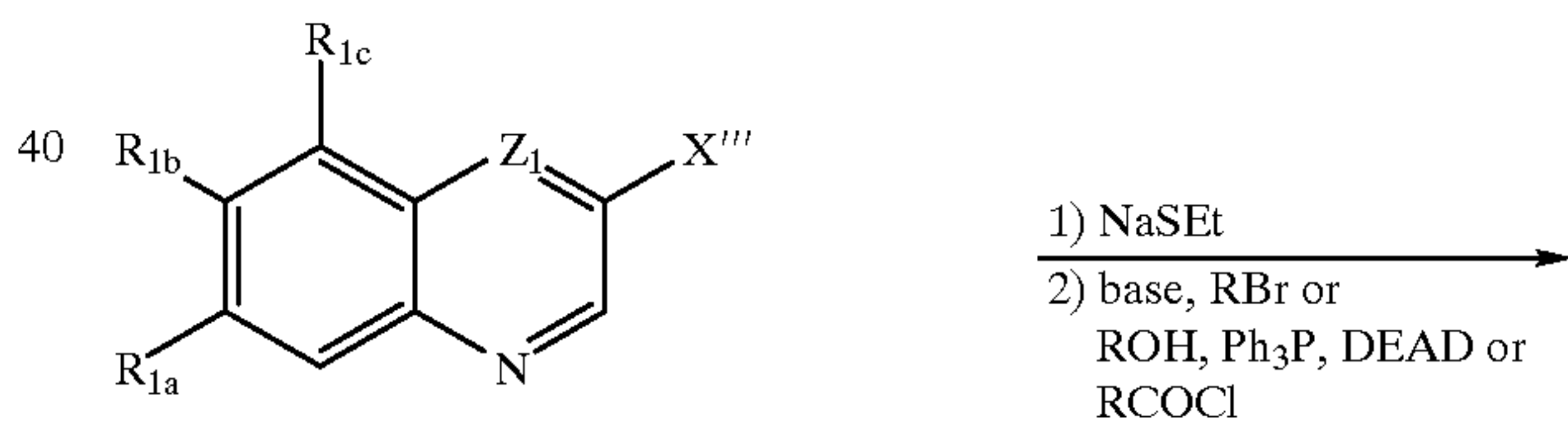
Scheme VI
