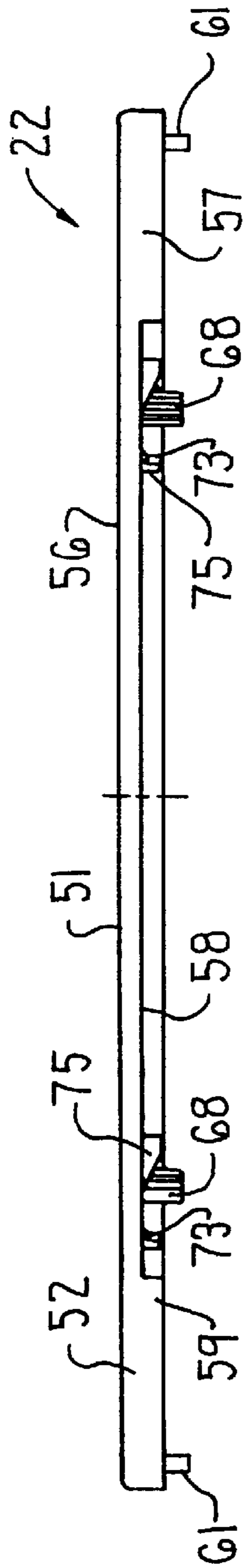
FIG. 7
