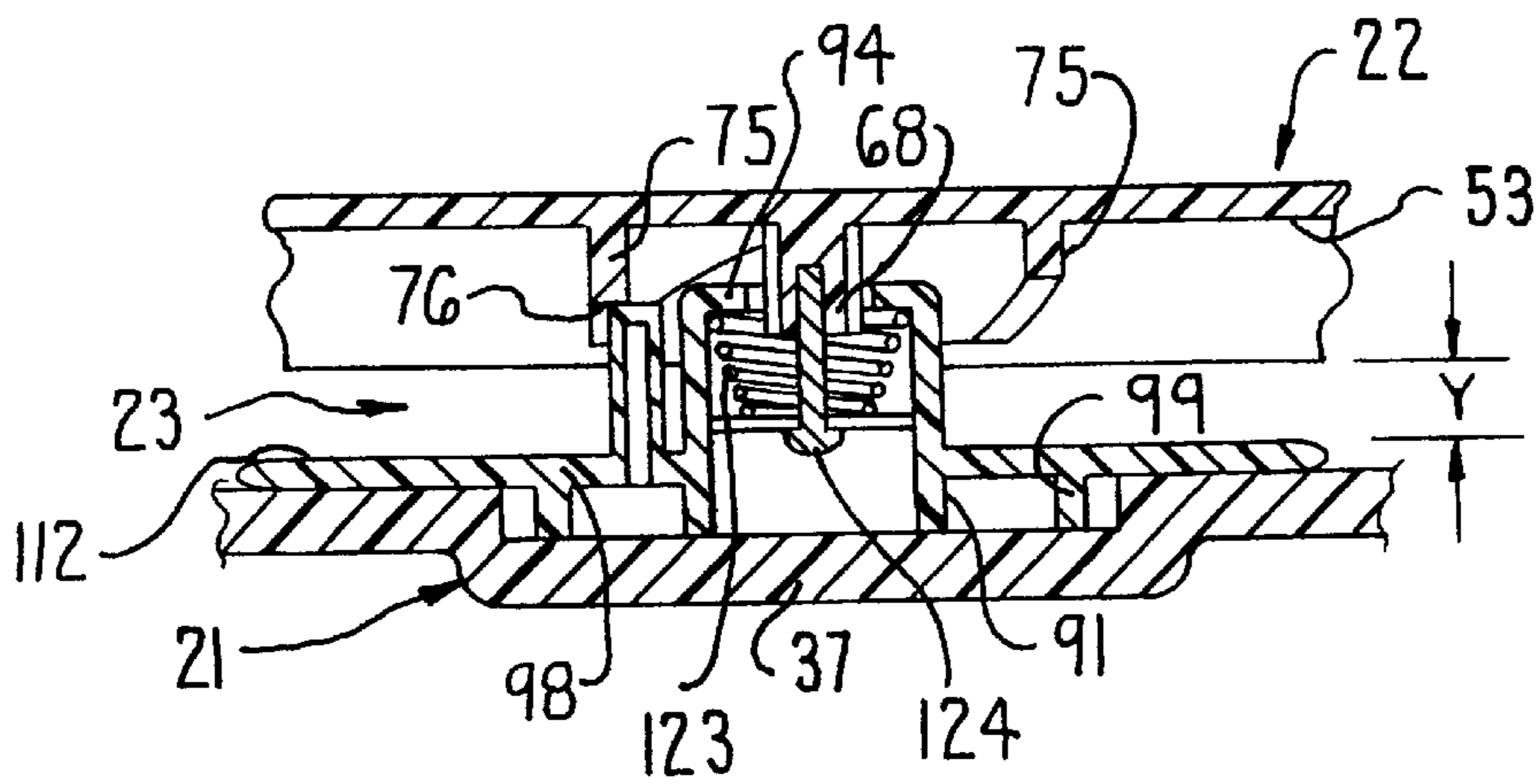
FIG. 17
