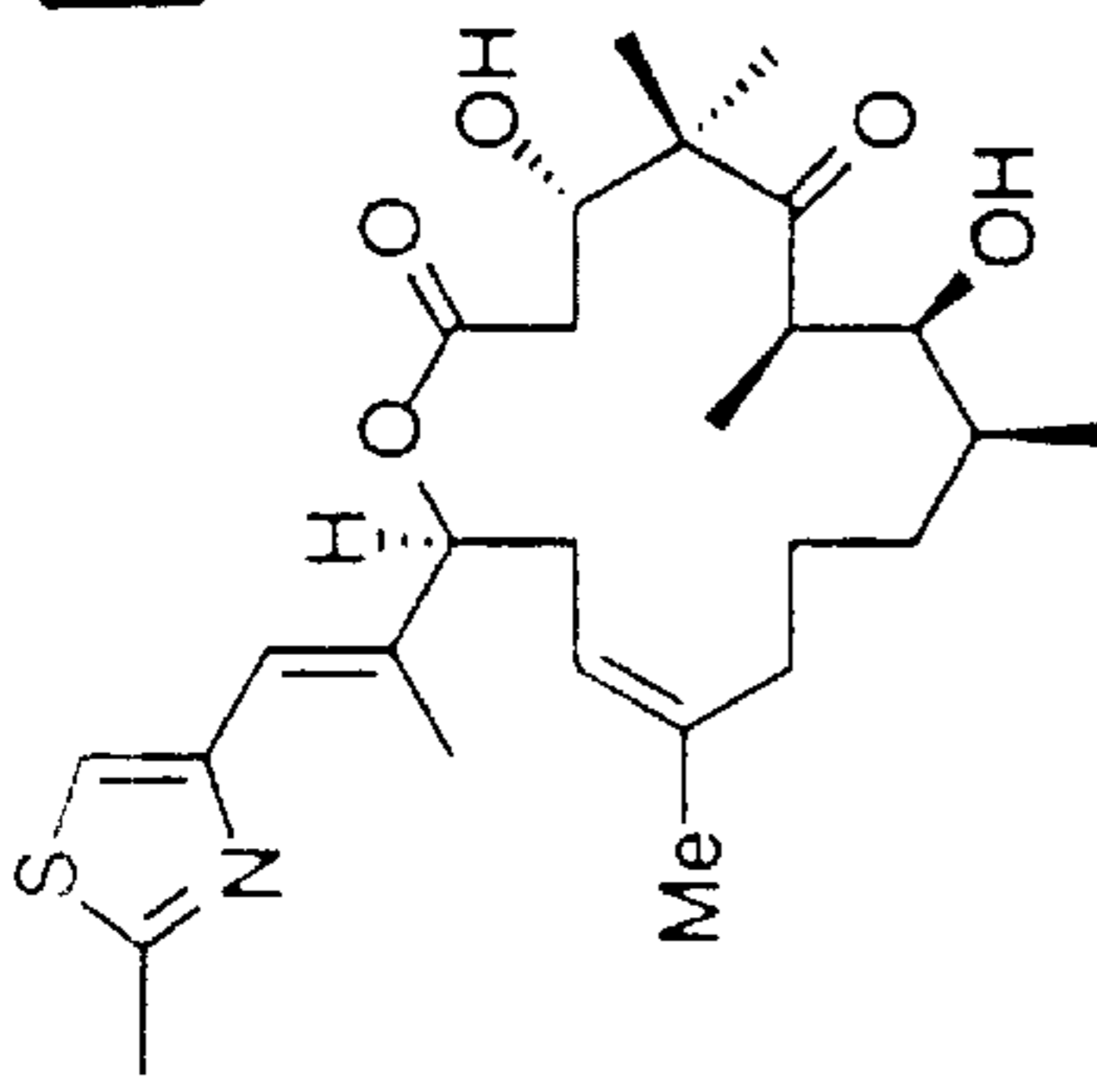
desoxyepothilone B
