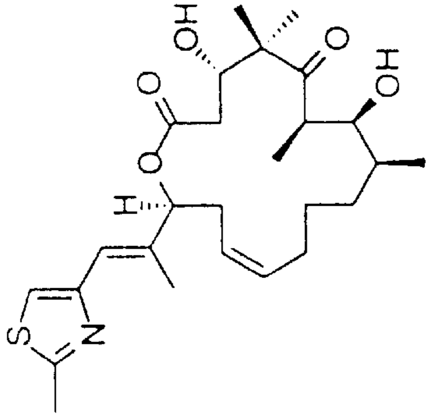
desoxyepothilone A
