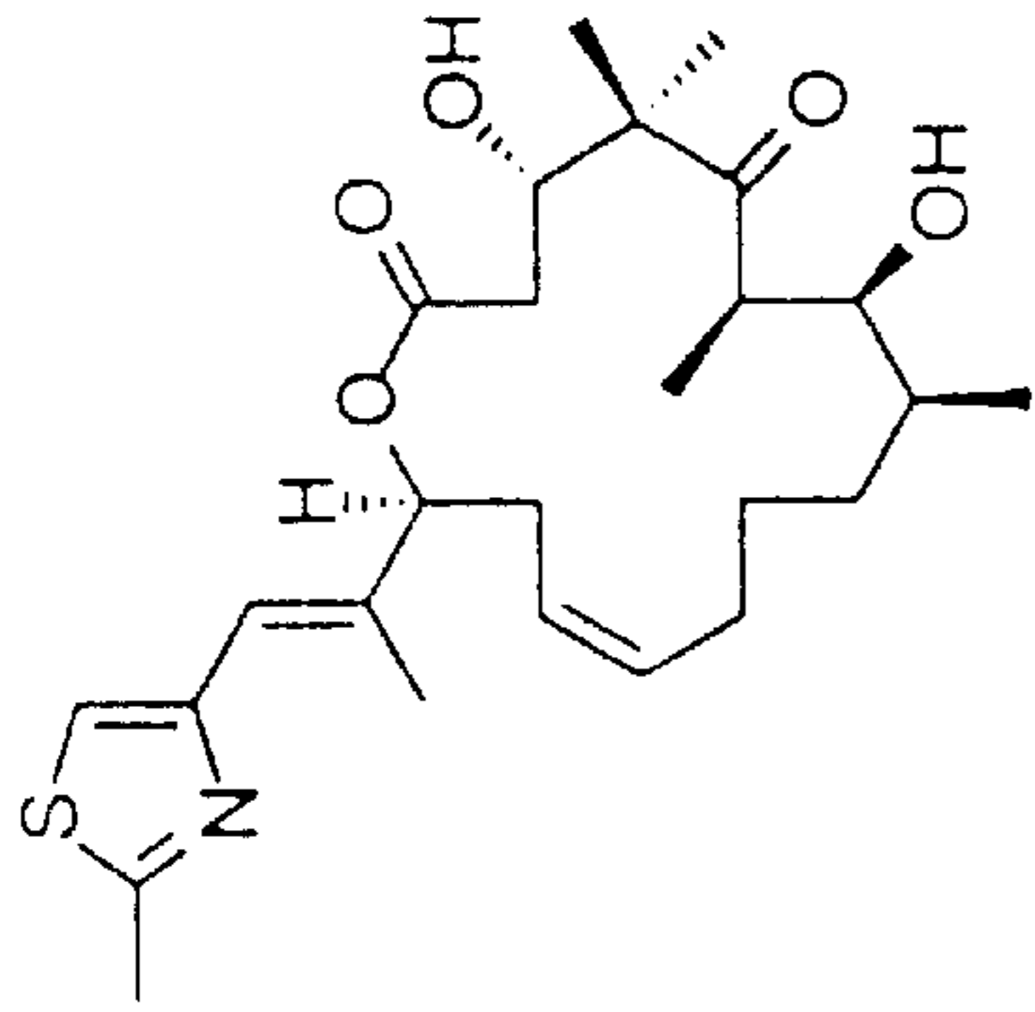
desoxyepothilone A
