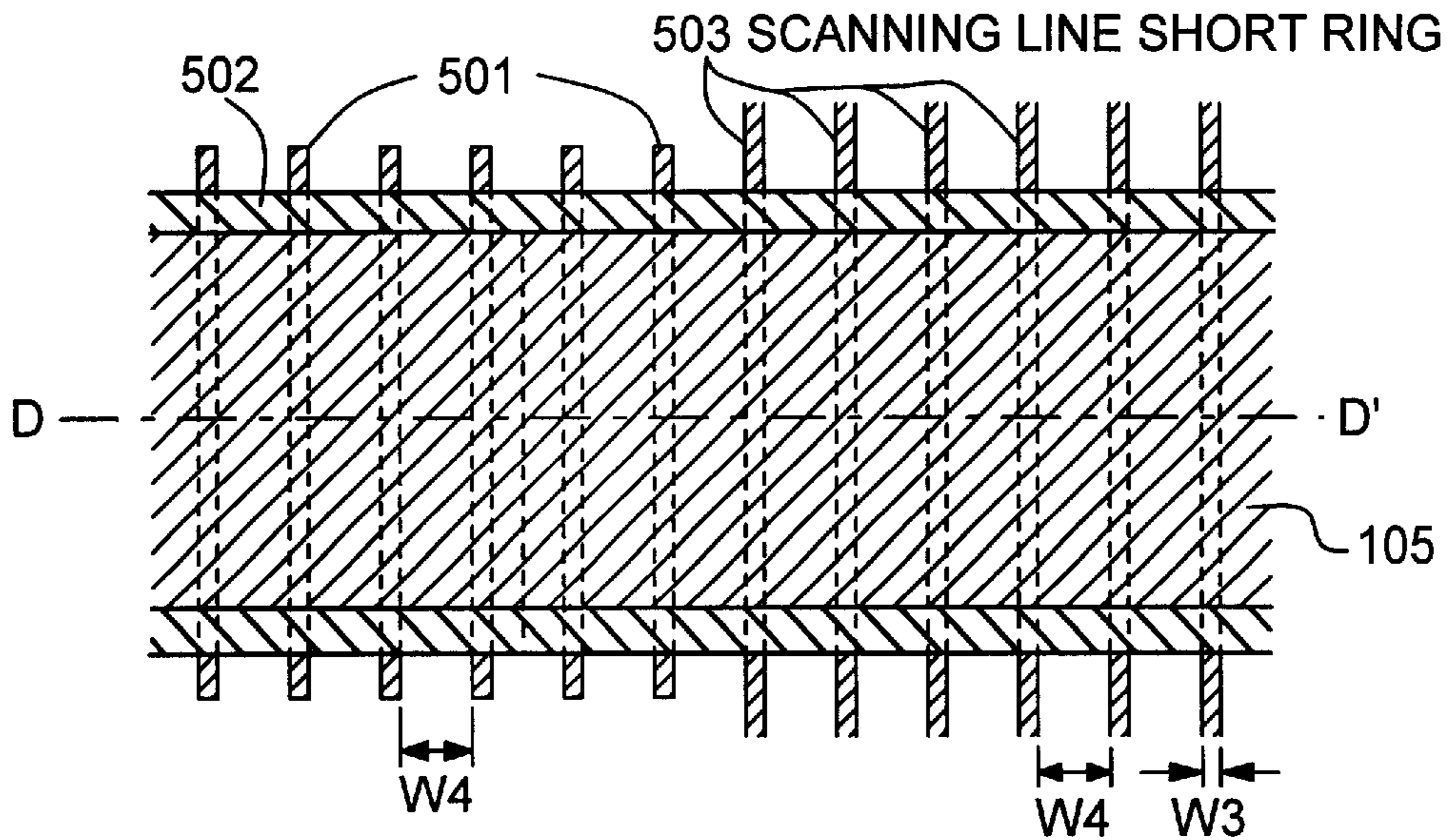
FIG. 8A
