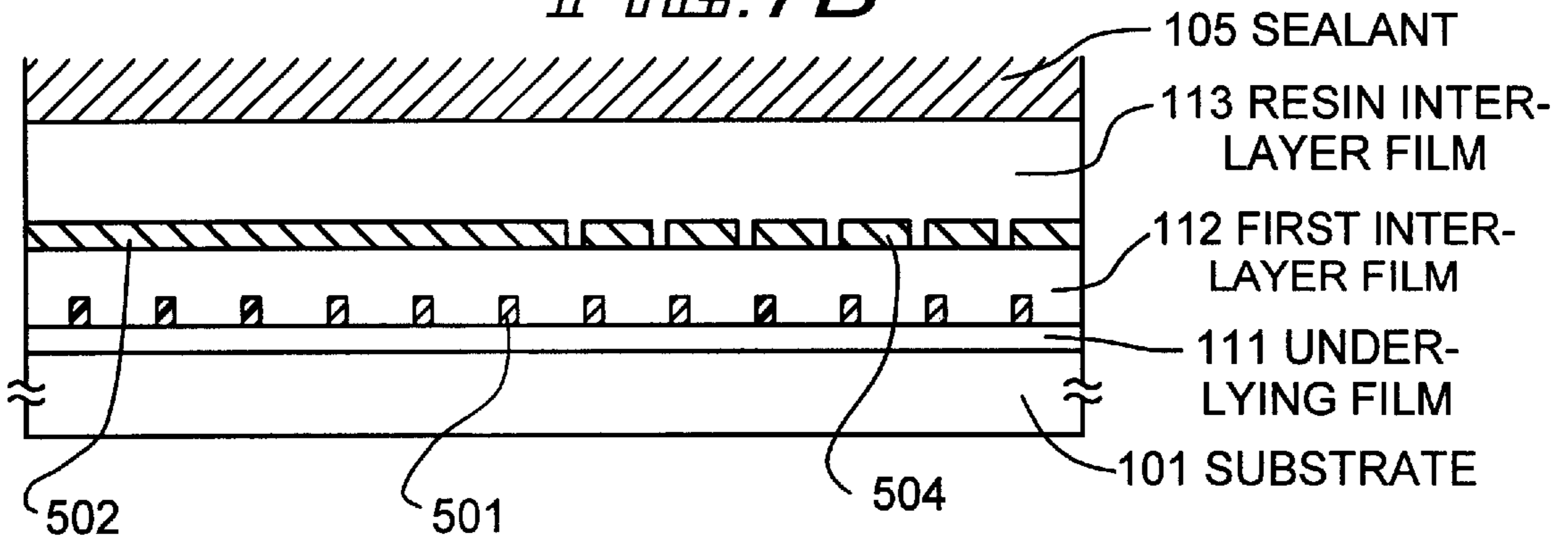
FIG. 7B
