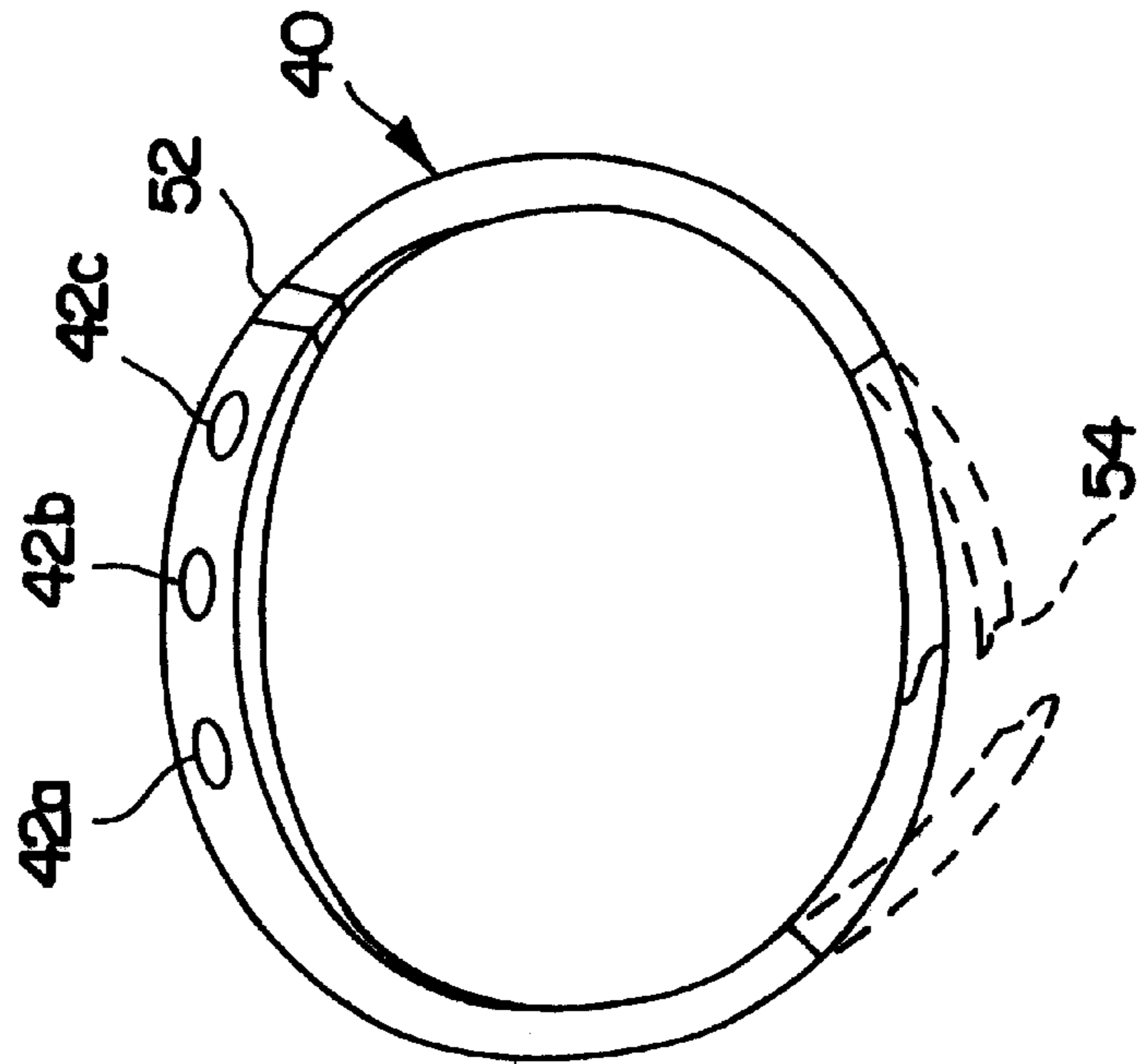
FIG. 3A
