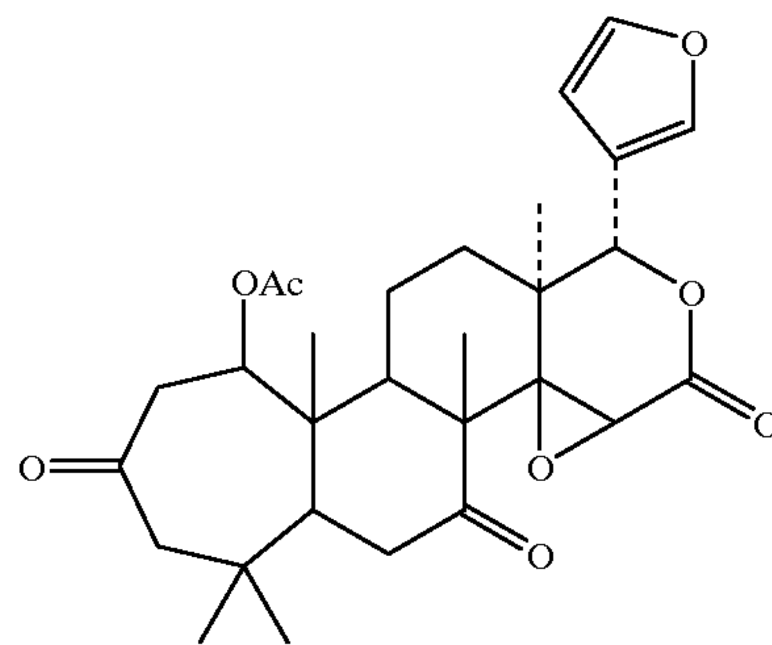
Nomillin
