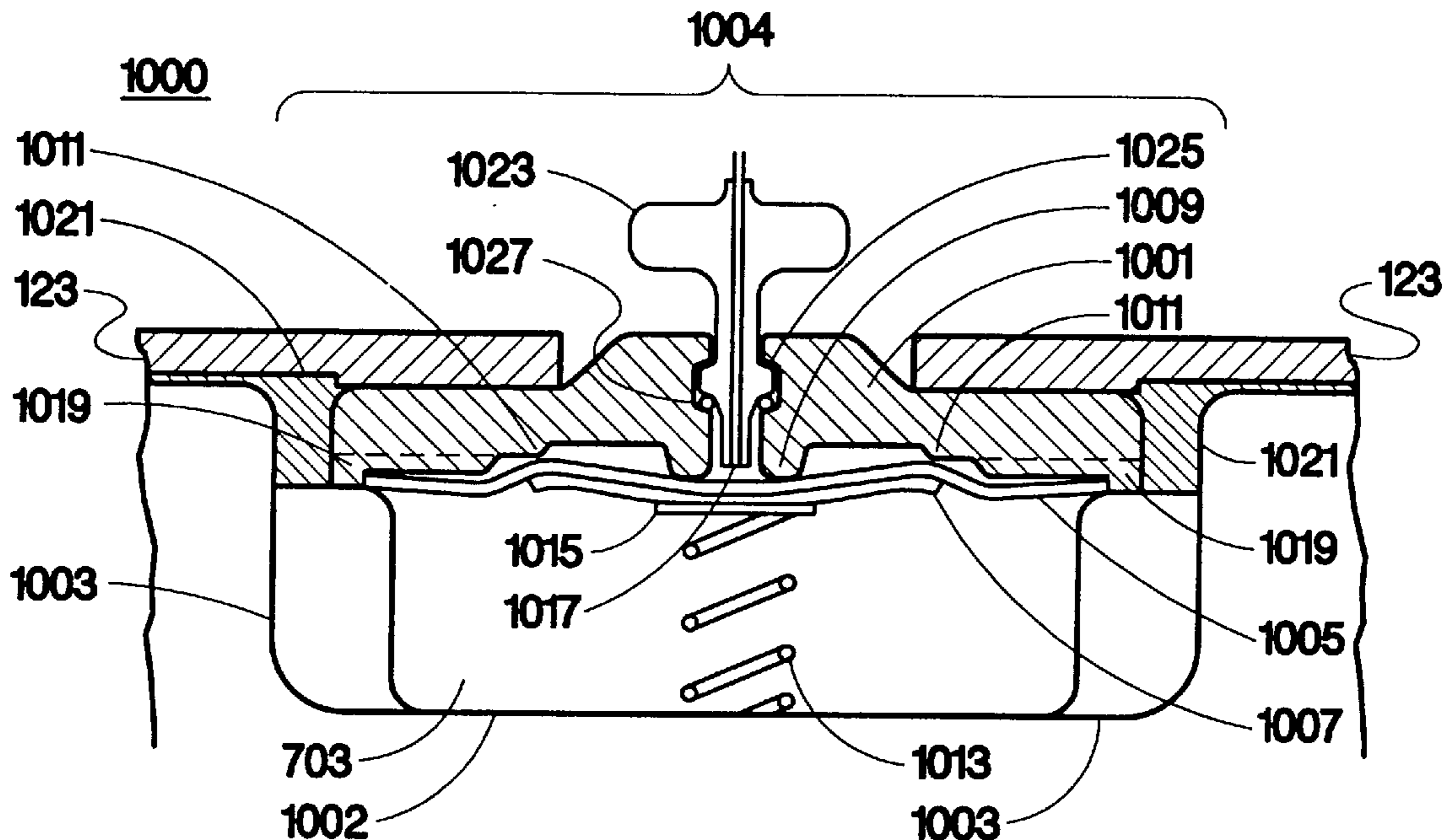
SECTION D-D
