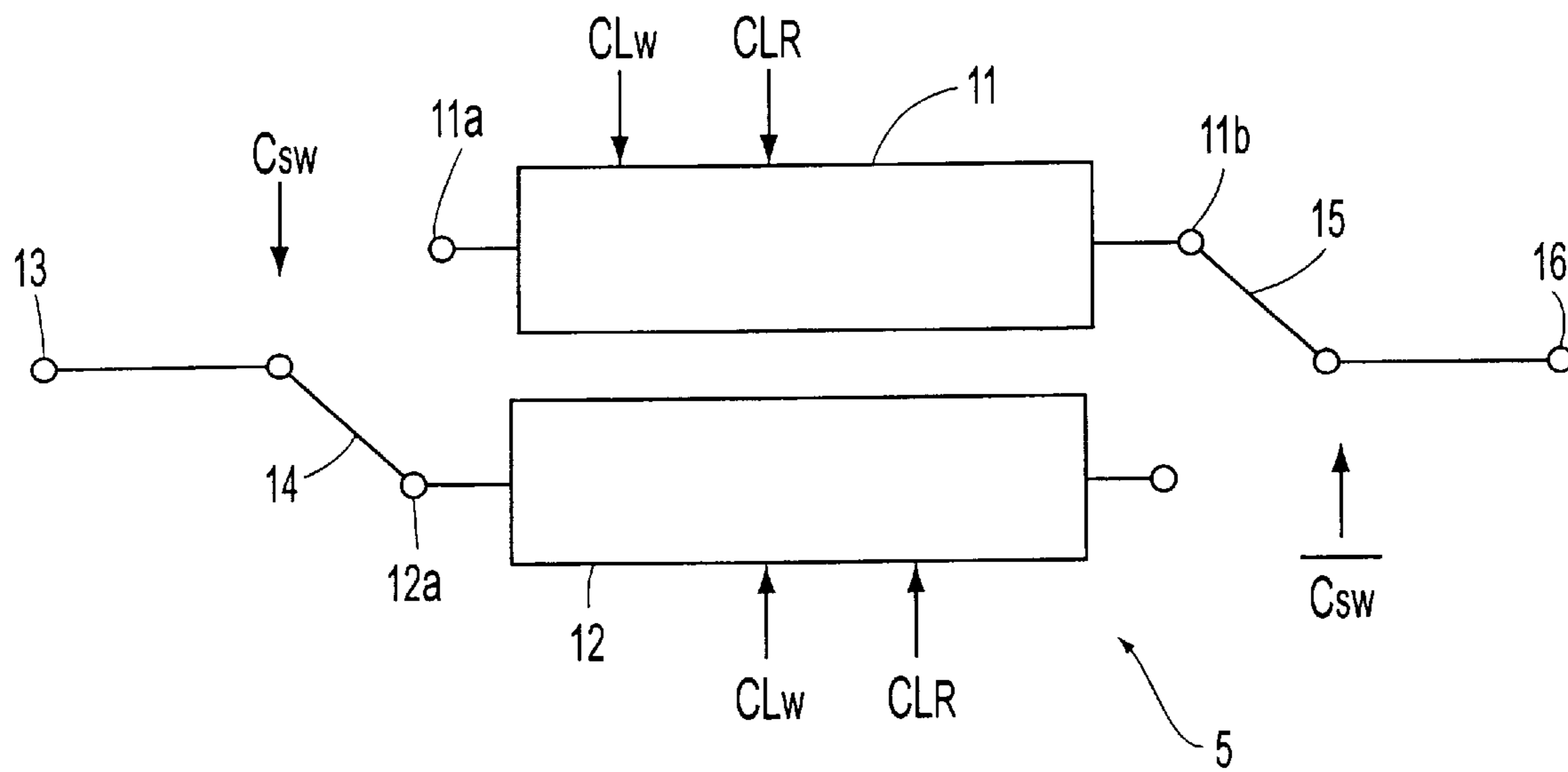
FIG.1(b)
