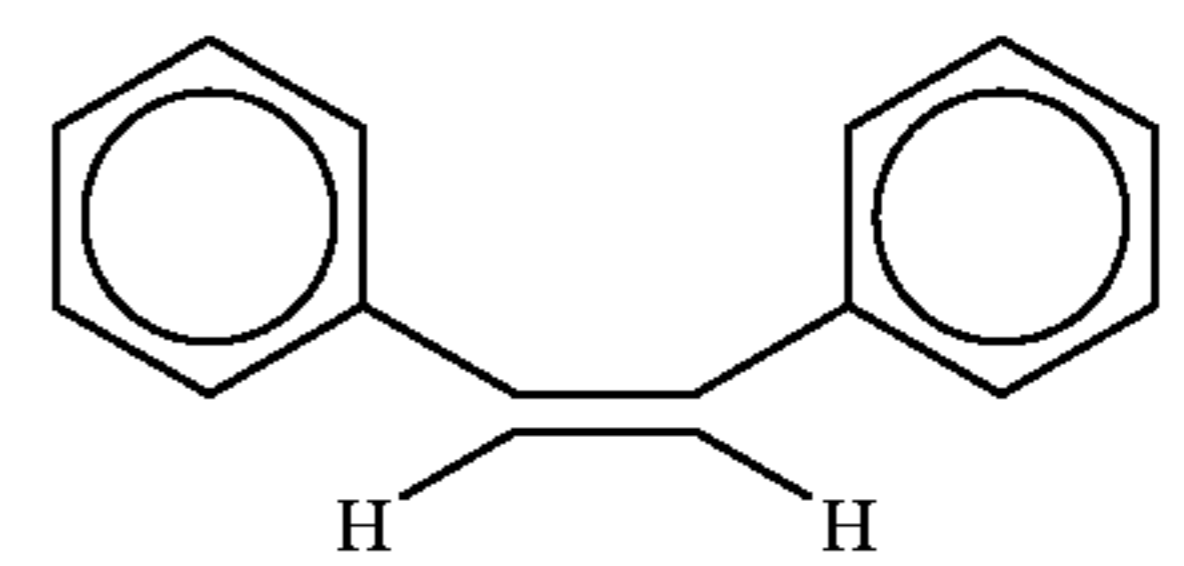
z-stilbene
