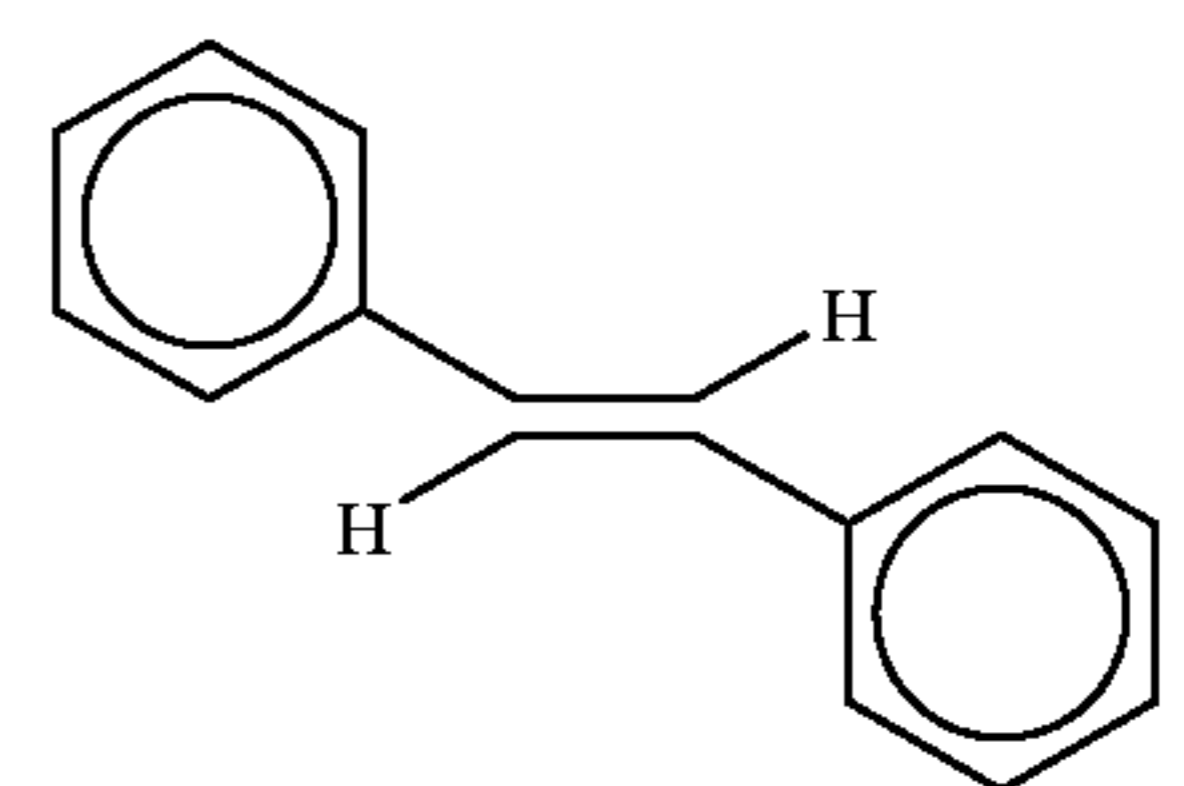
e-stilbene
