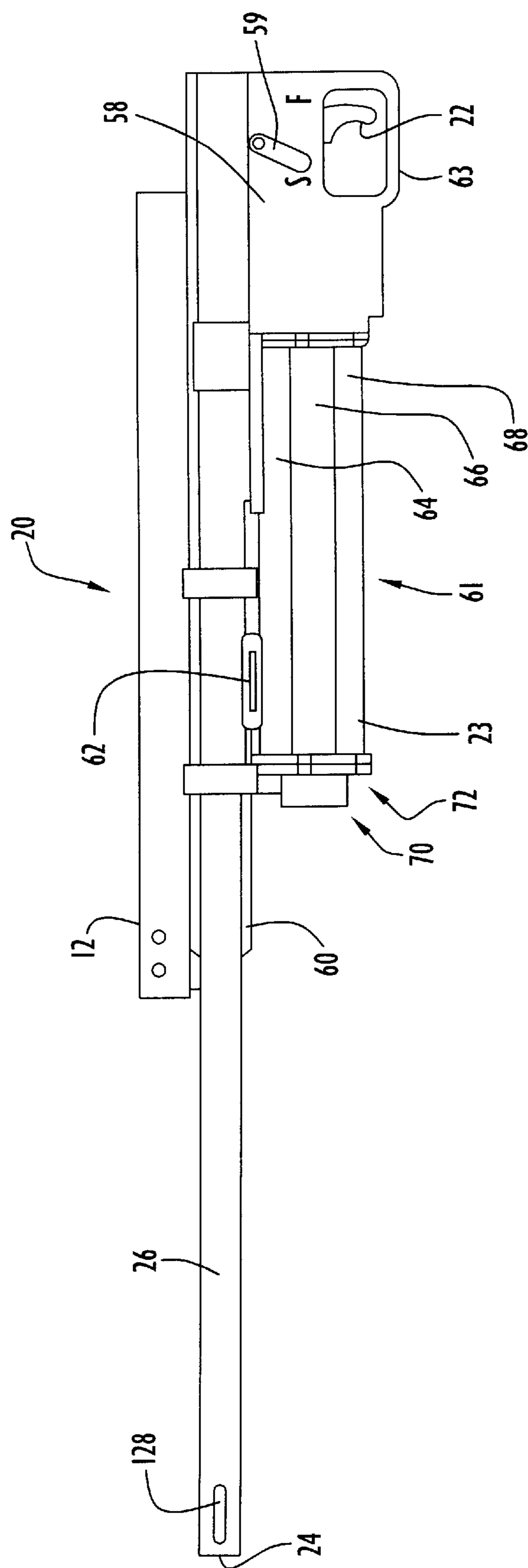
FIG.8
