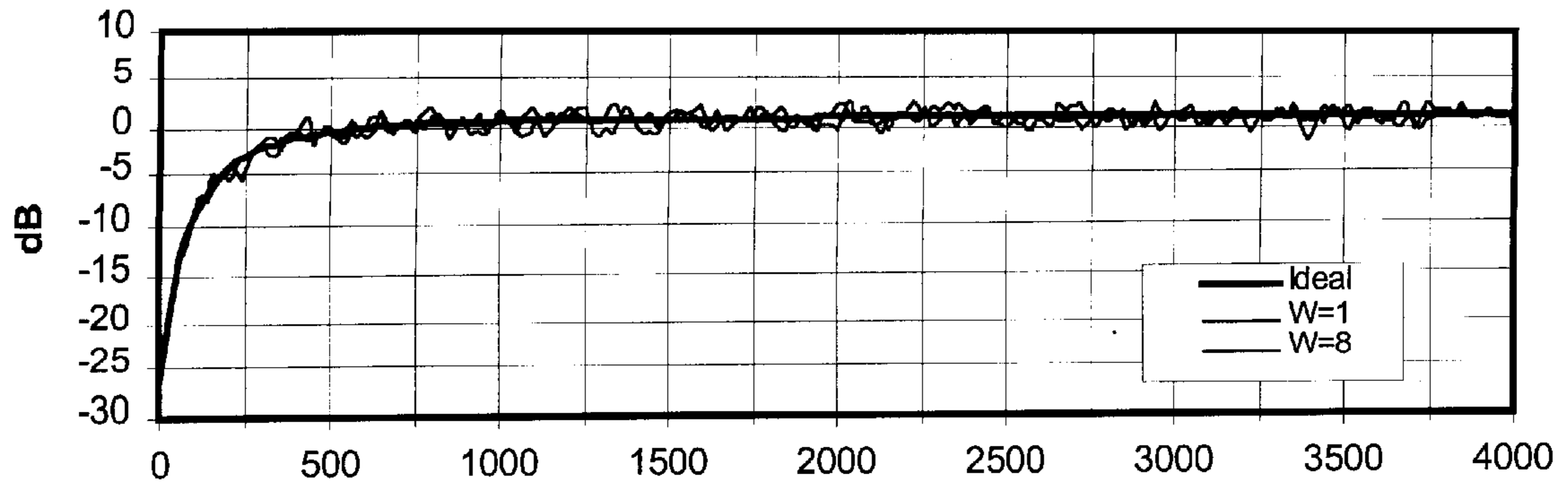
Figure 3a. Test A, HPF, Linear Values
