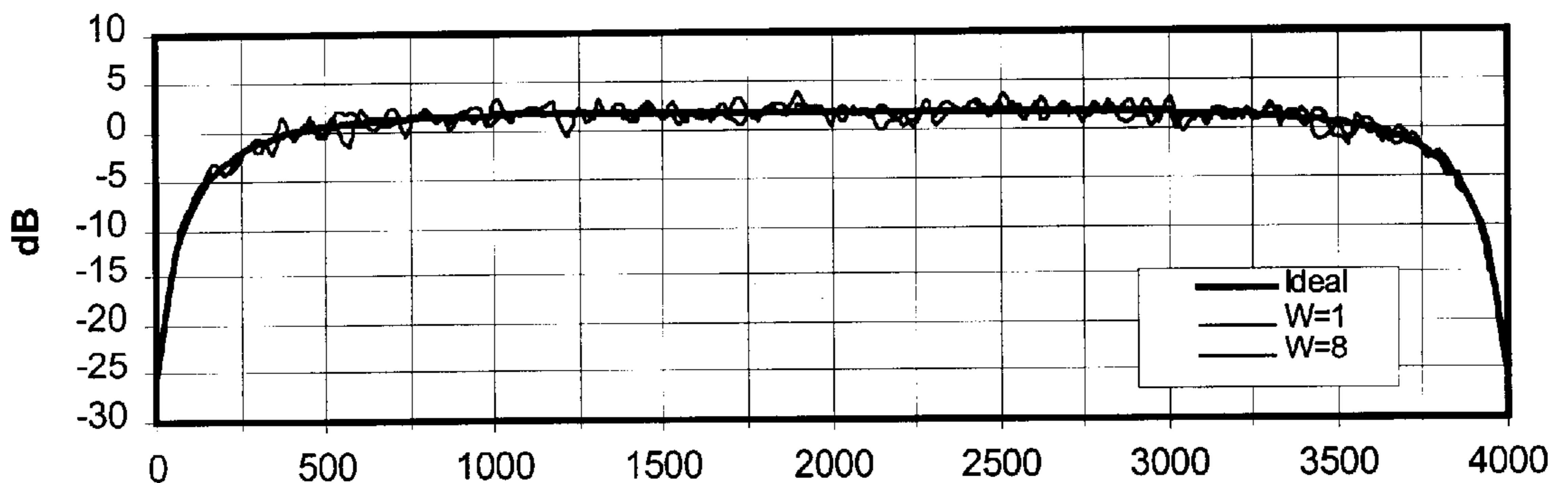
Figure 4c. Test C, BPF, PCM Values
