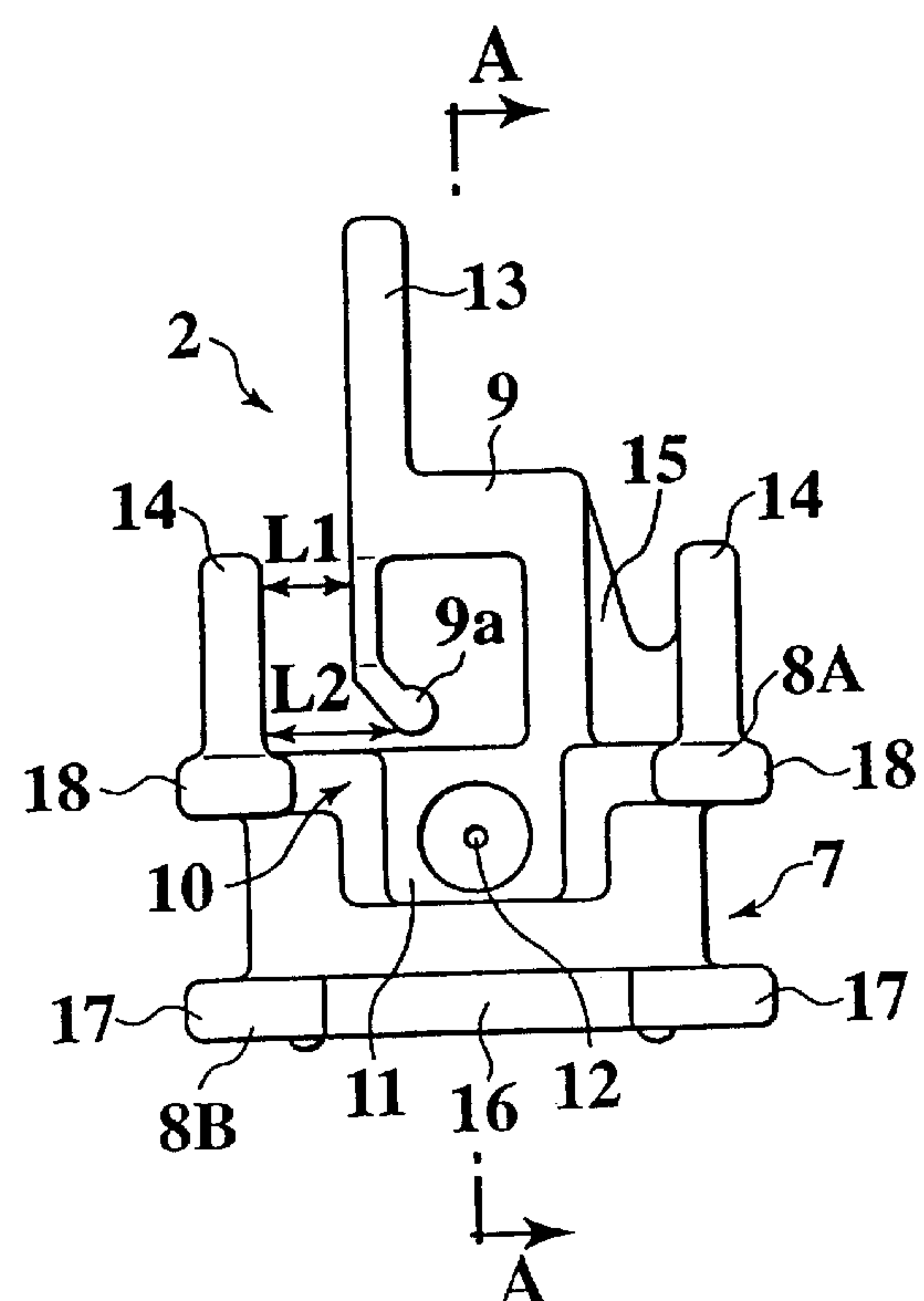
FIG.3A
