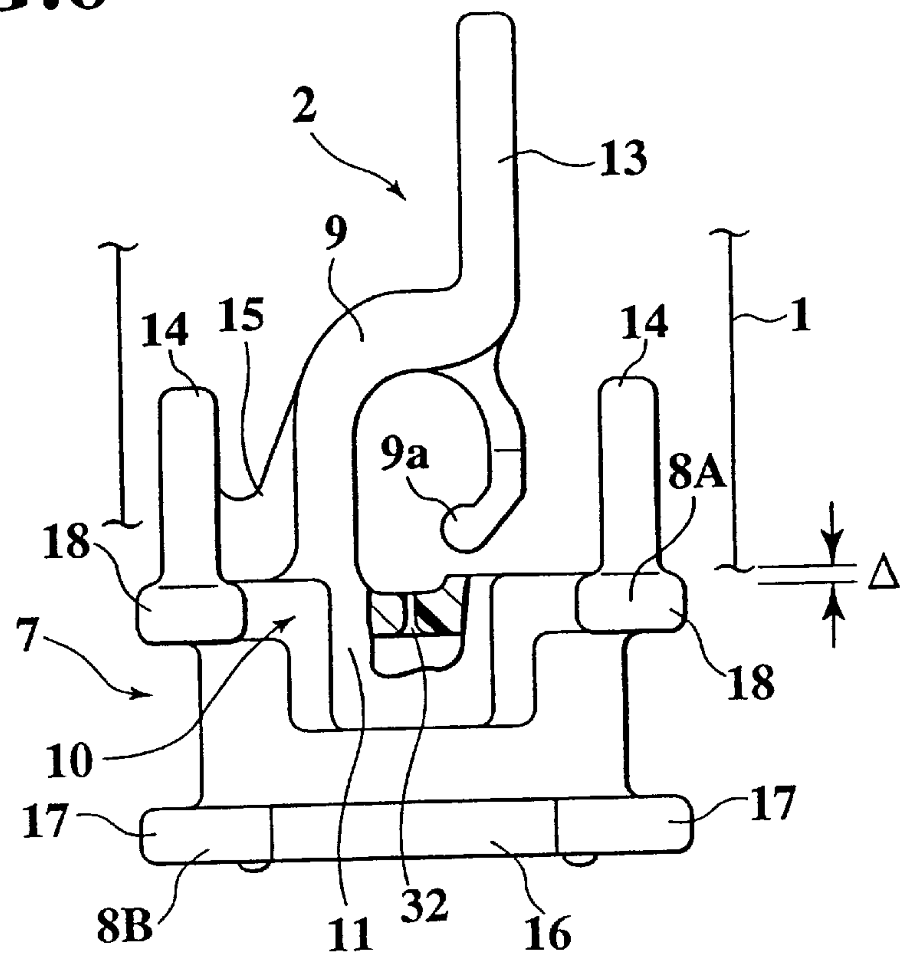
FIG.6
