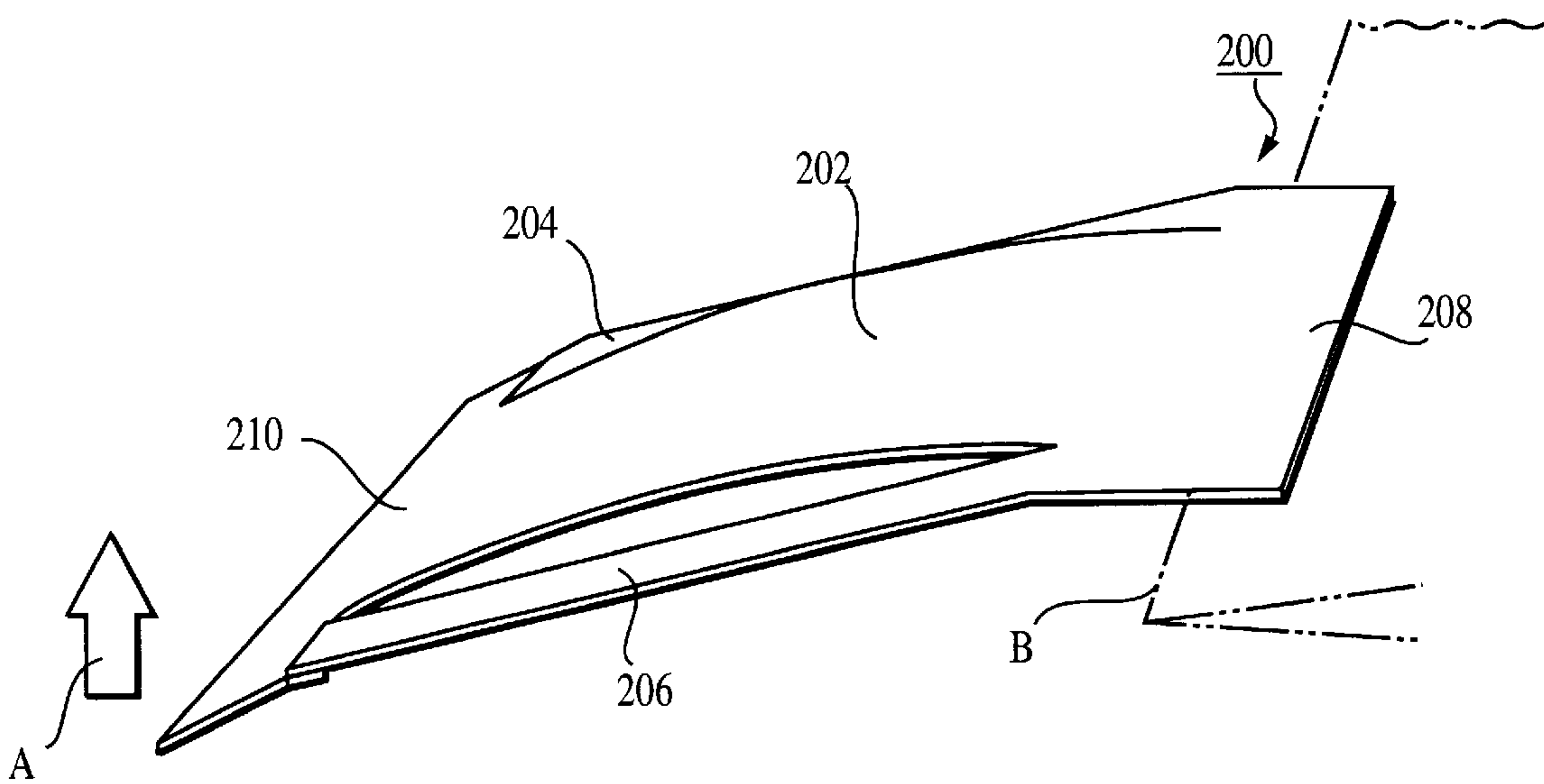
FIG. 5B
