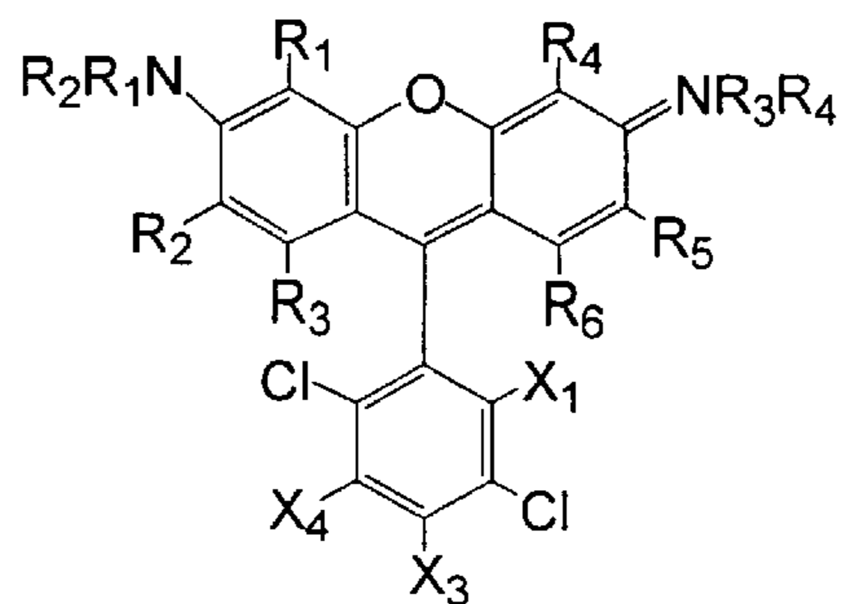
4,7-Dichlororhodamine
