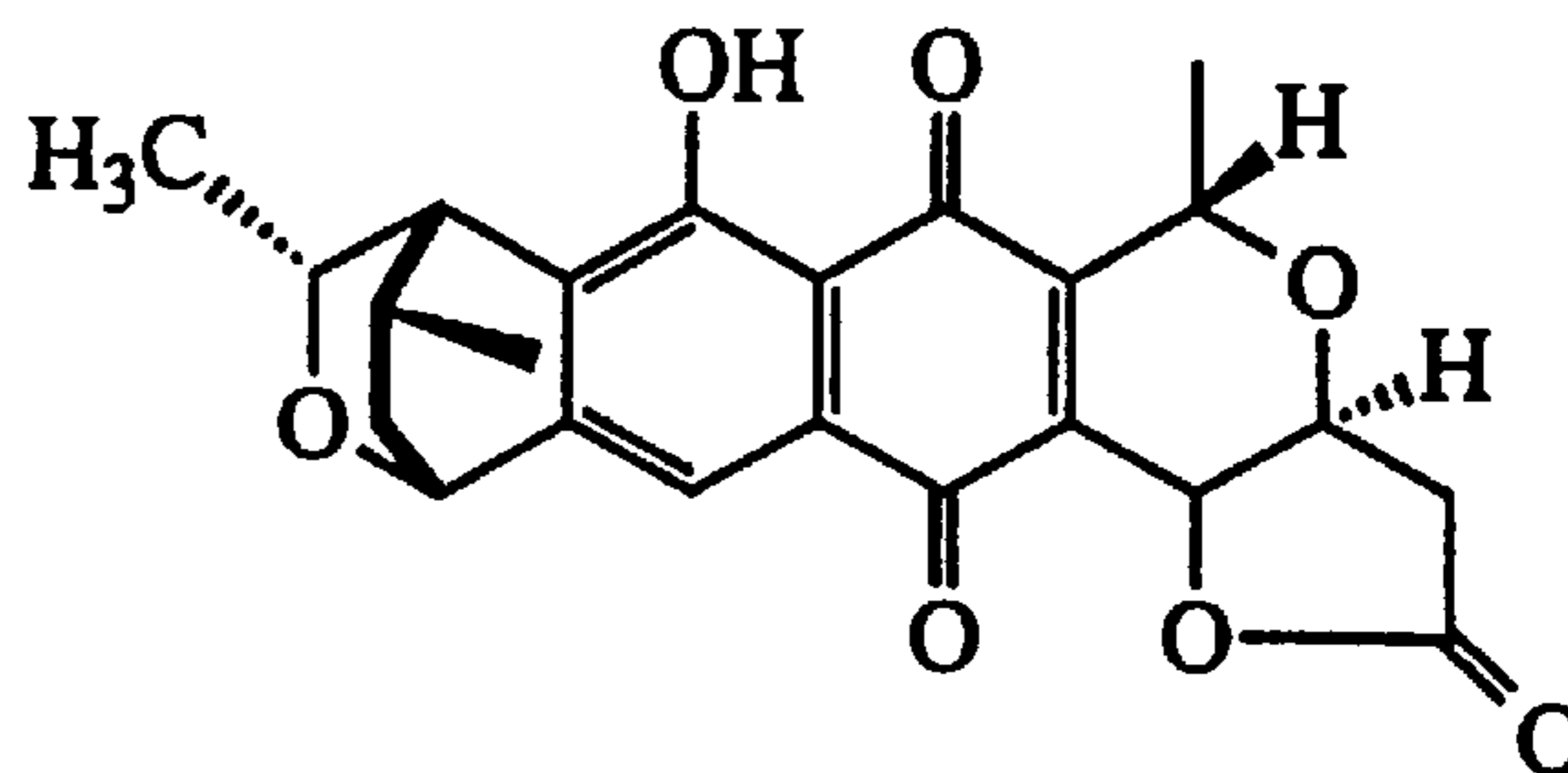
GRANATICIN (4)
