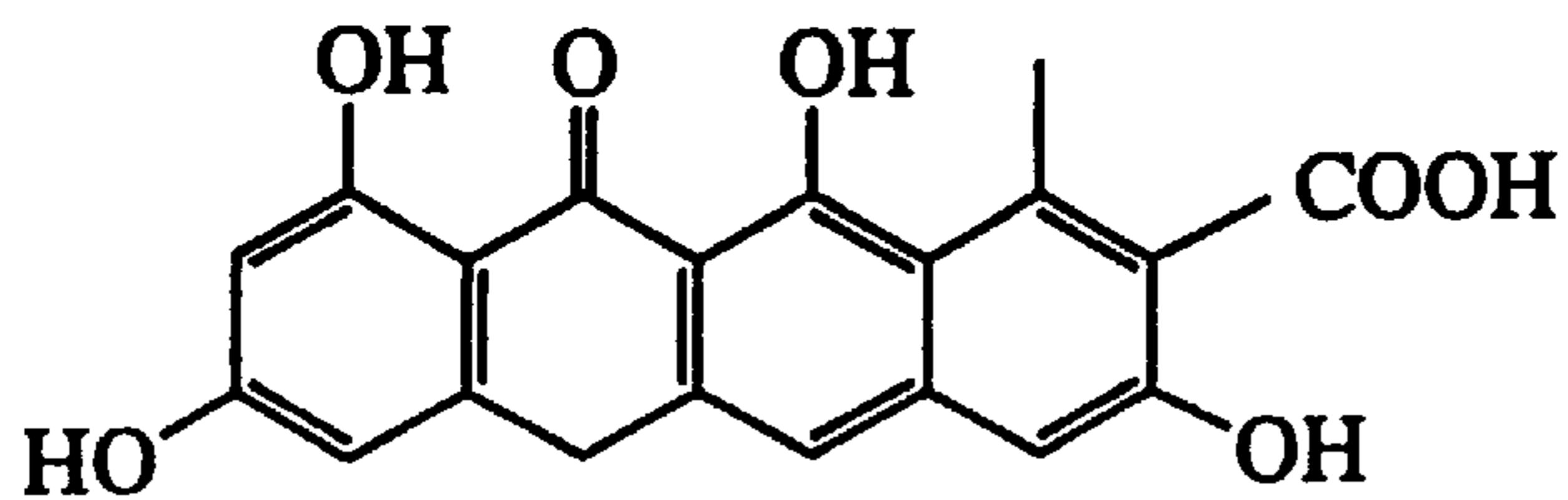
TETRACENOMYCIN F1 (5)
