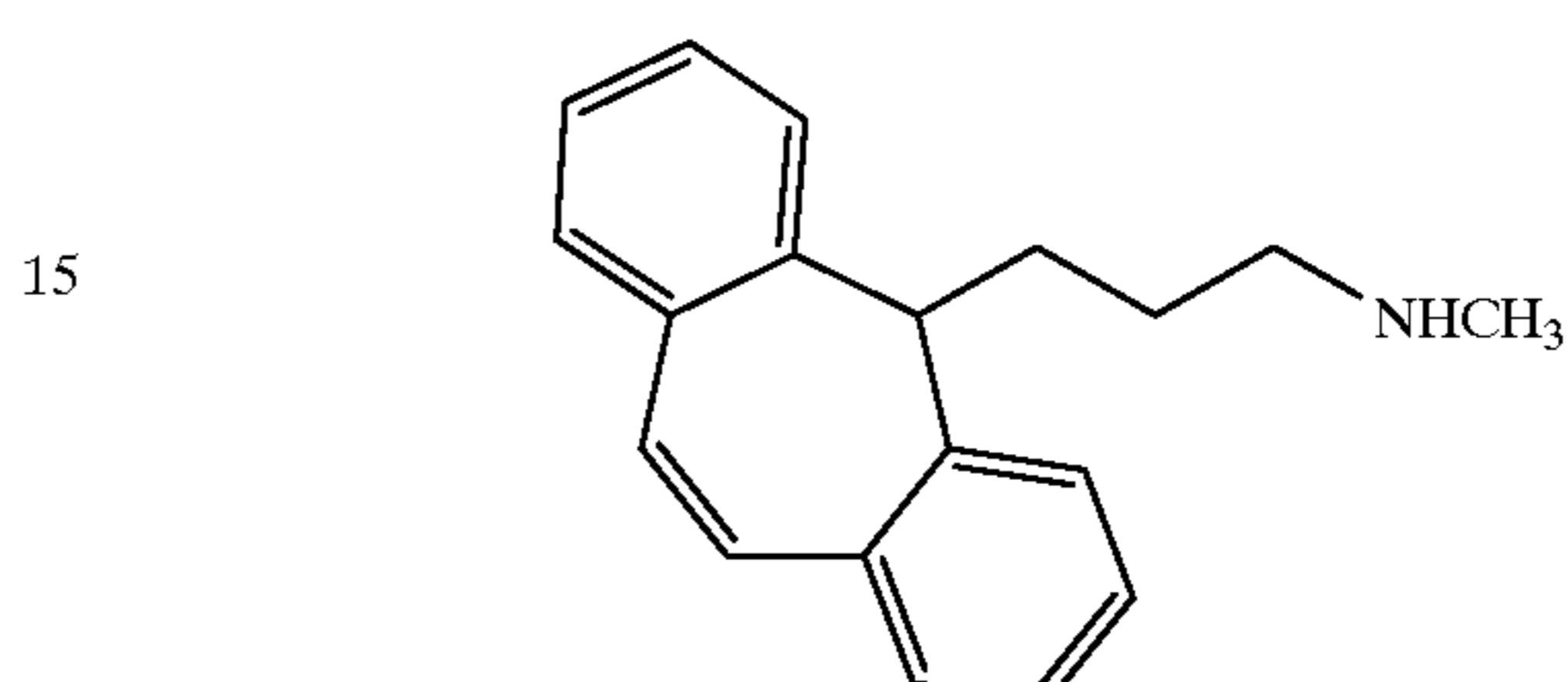
Protrylptyline
