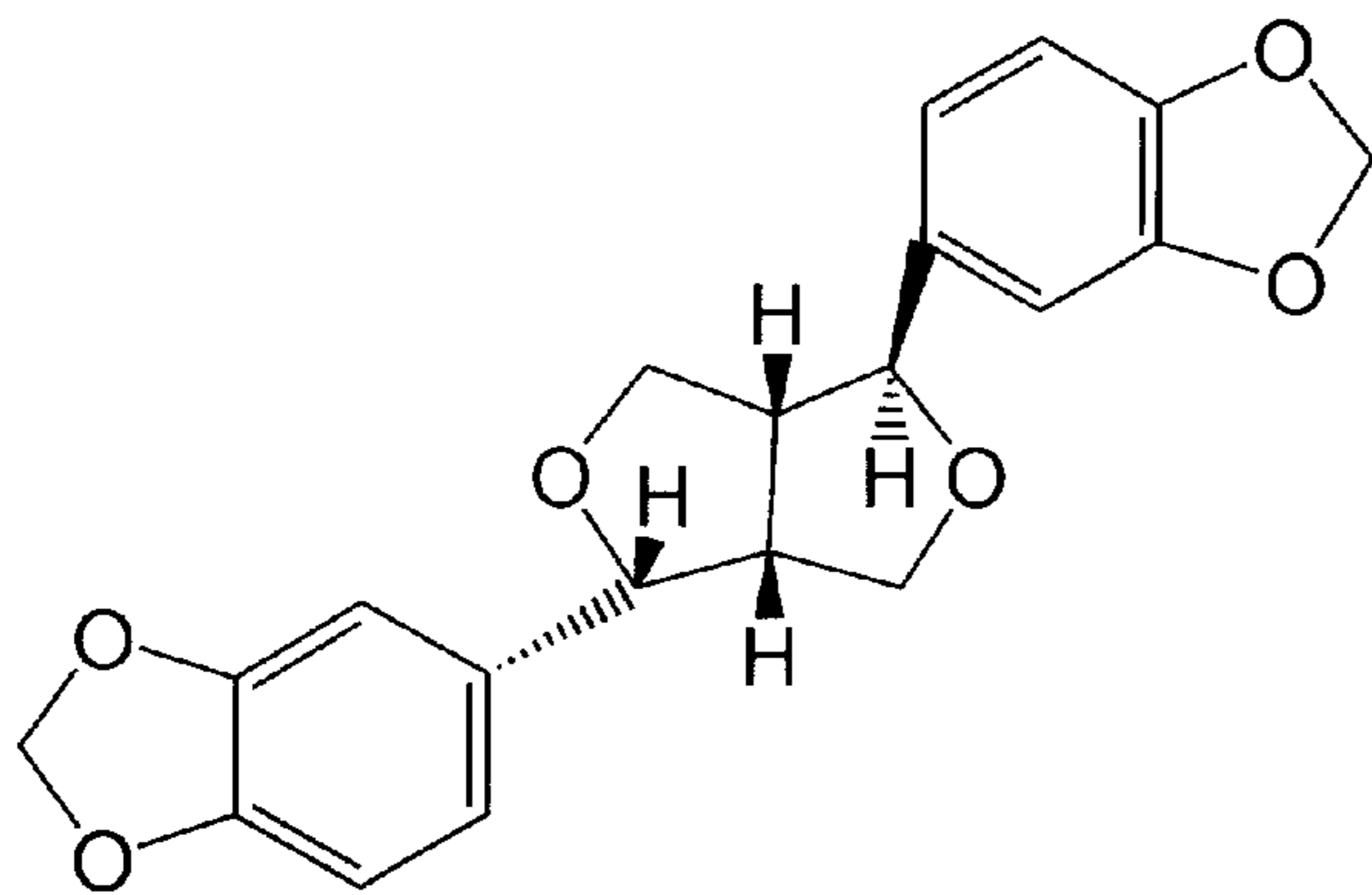
ASARININ
