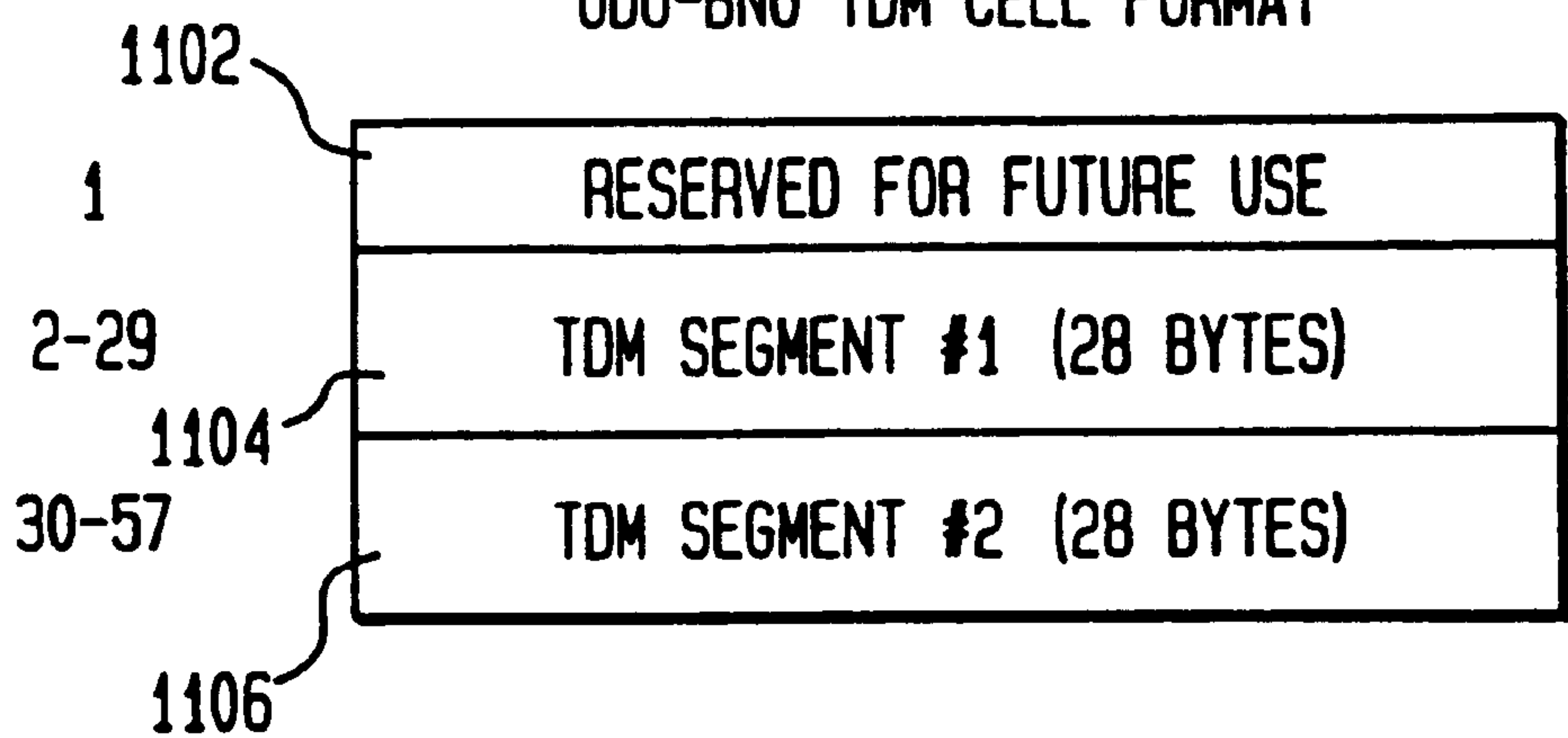
FIG. 14A ODU-BNU TDM CELL FORMAT
