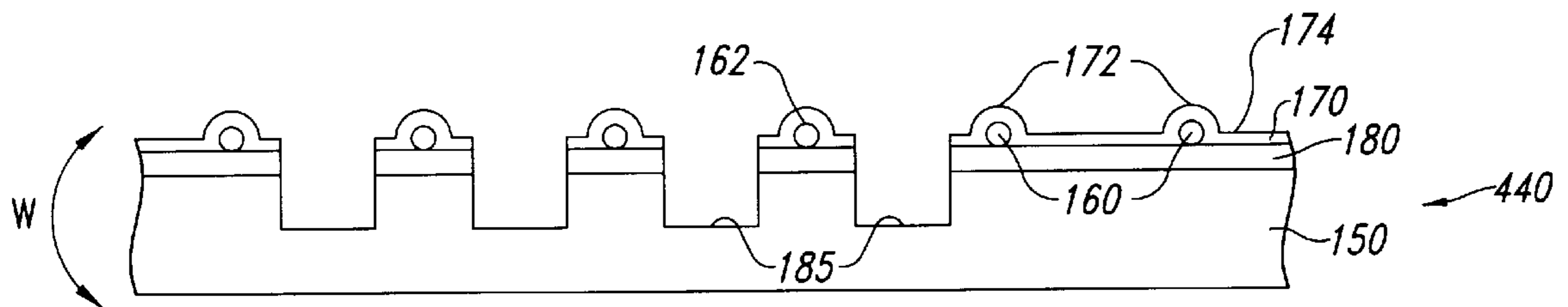
Fig. 8
