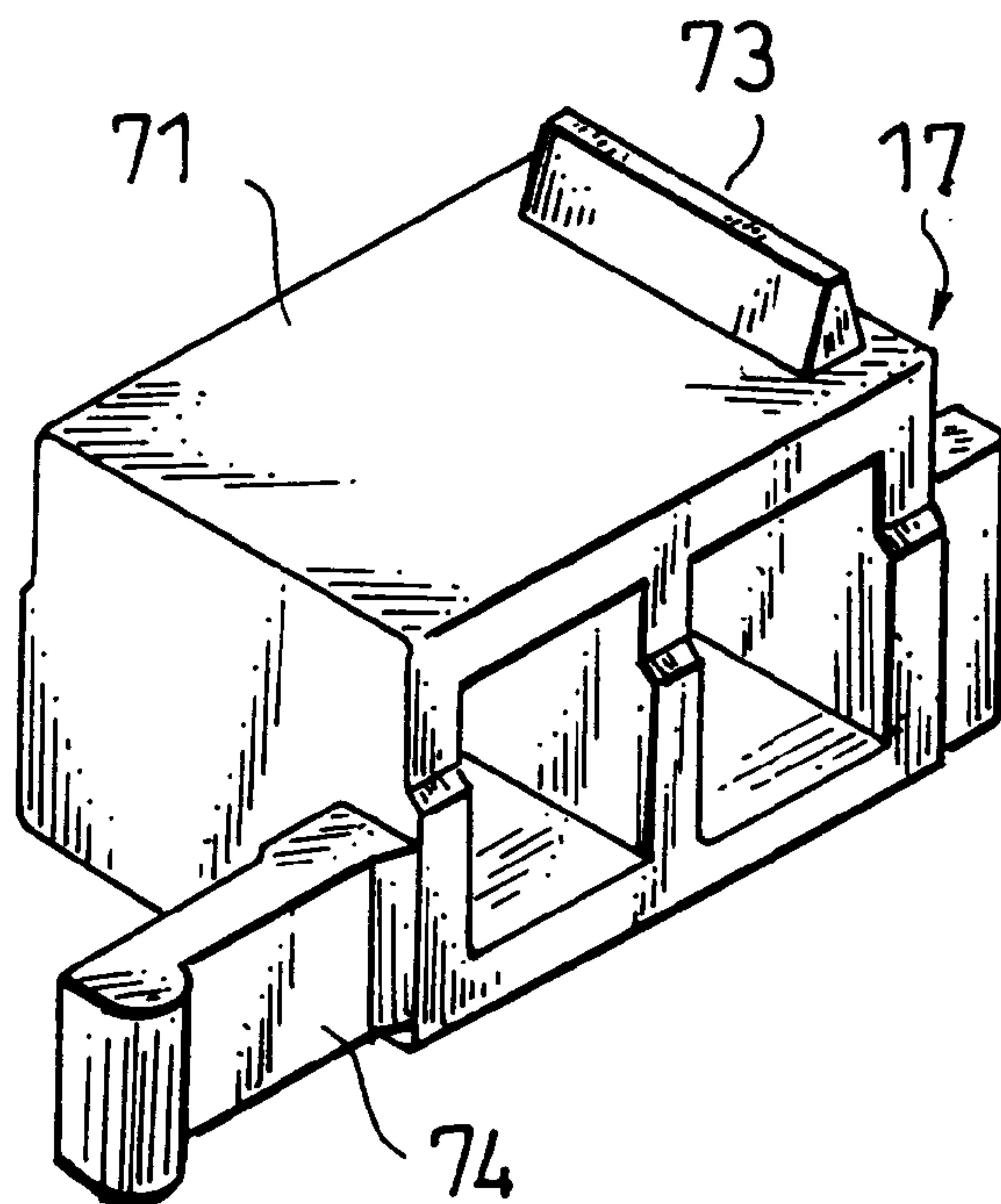
FIG. 4B
