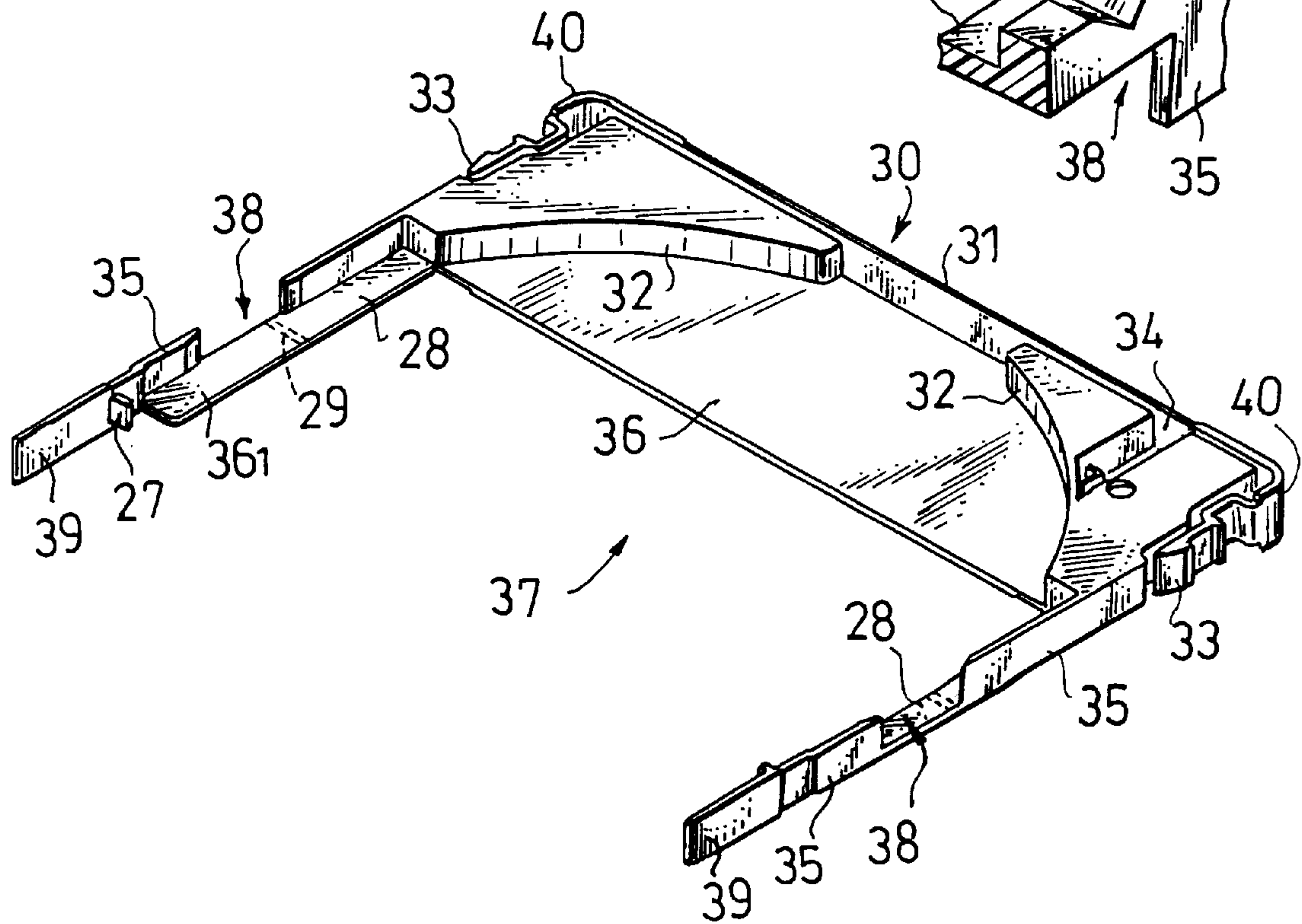
FIG. 9C
