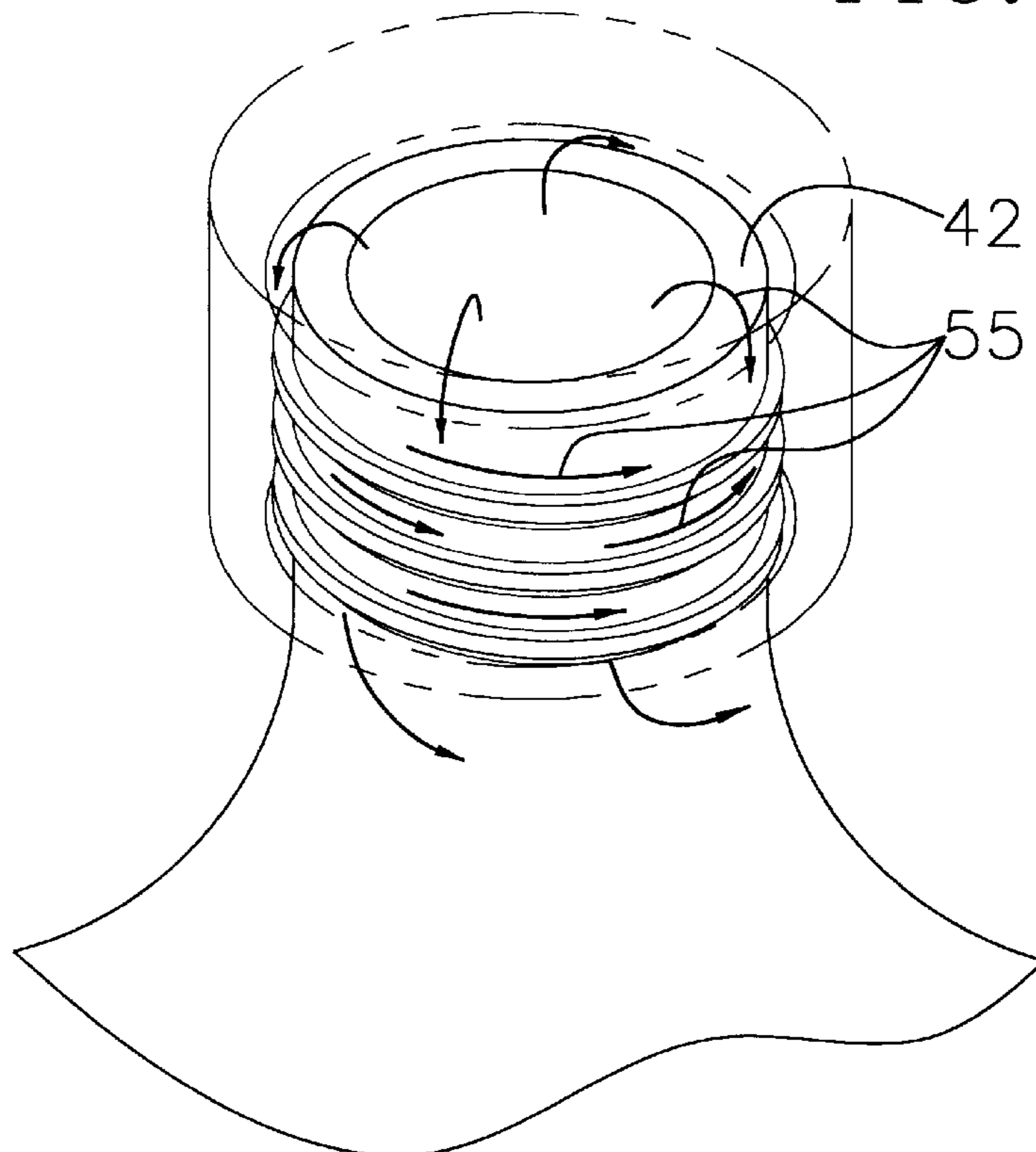
FIG. 3B
