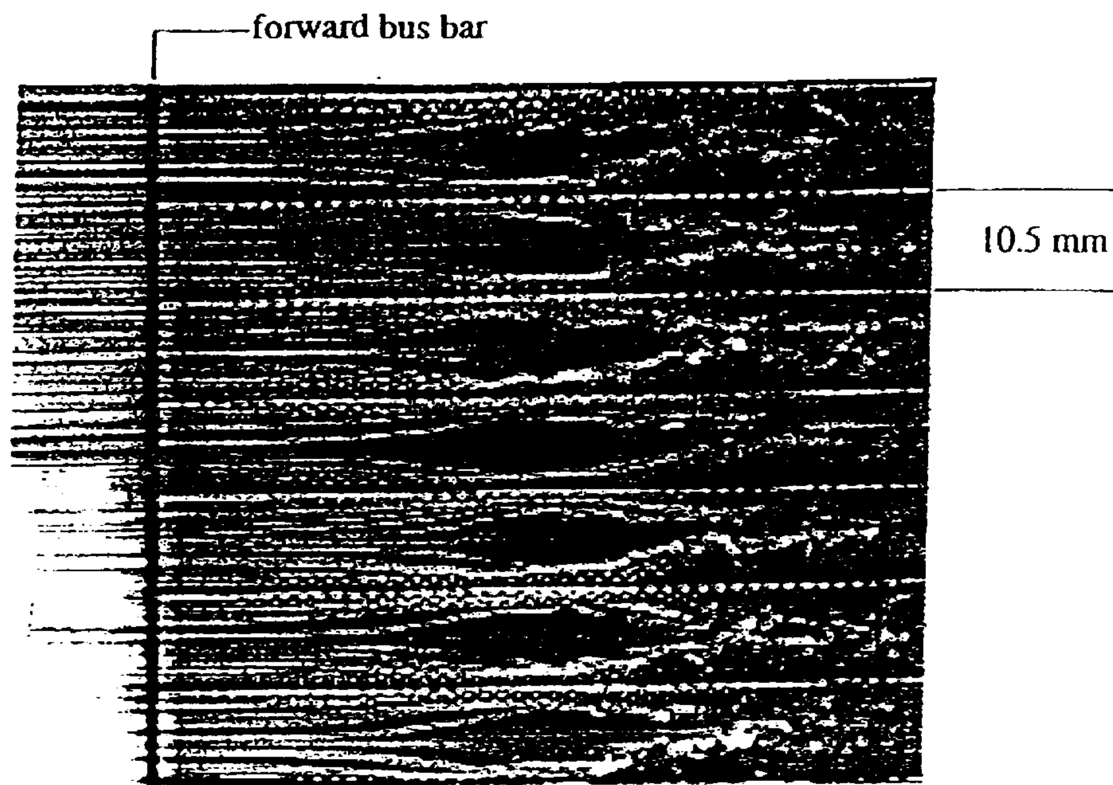
(a) E=3\text{ kV rms} , F=3\text{ kHz}
