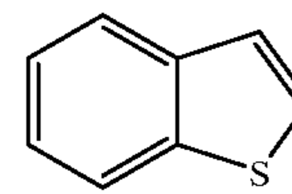
VII
