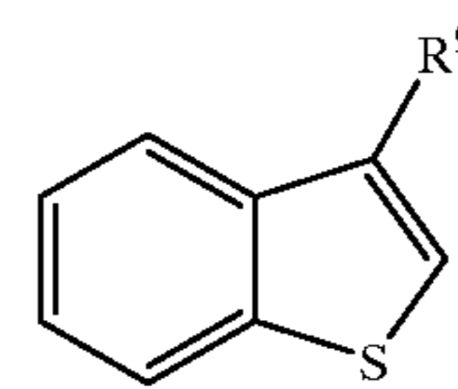
VIII
