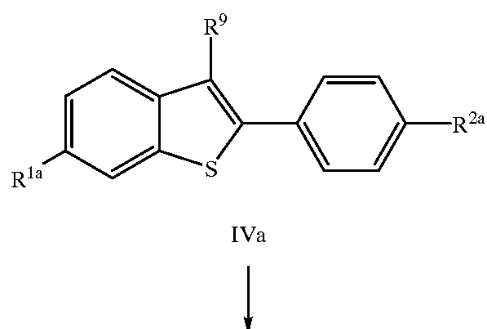
Scheme VI
