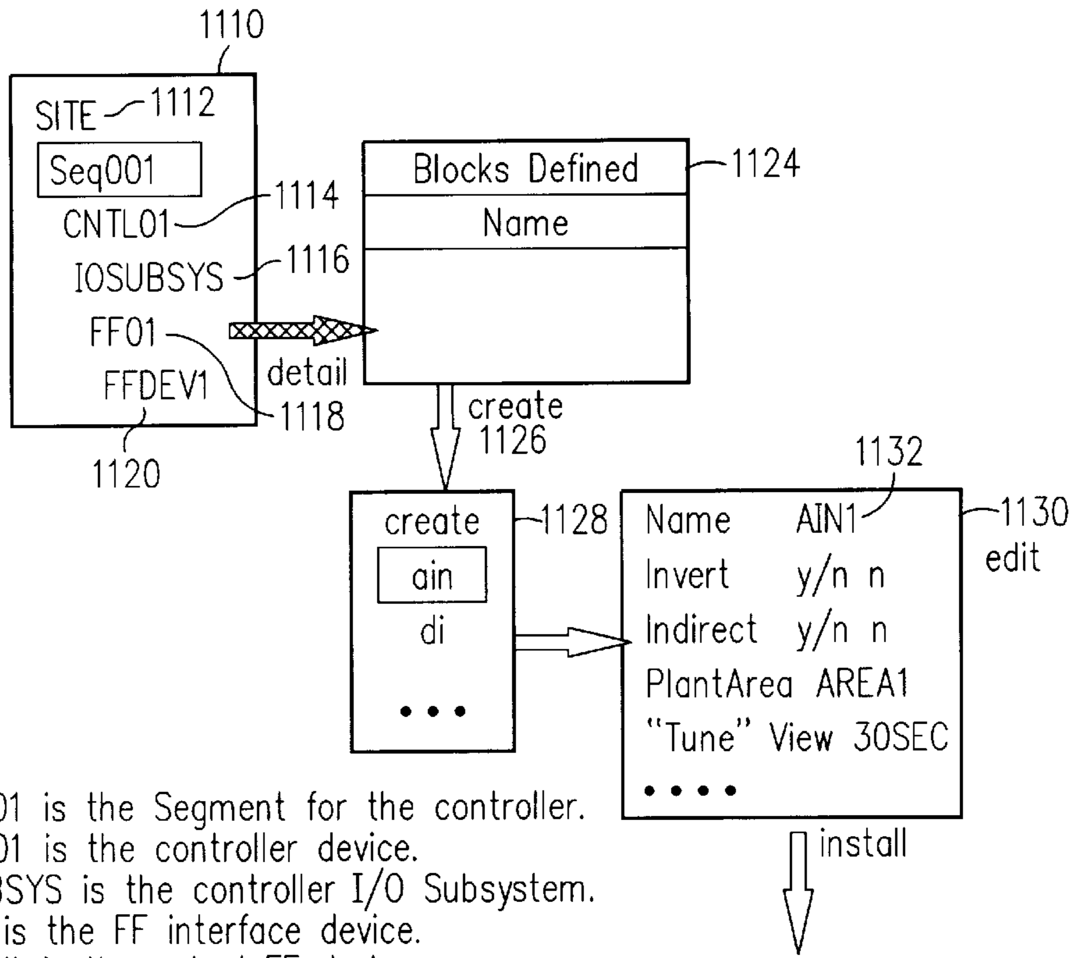
FIG. 12
