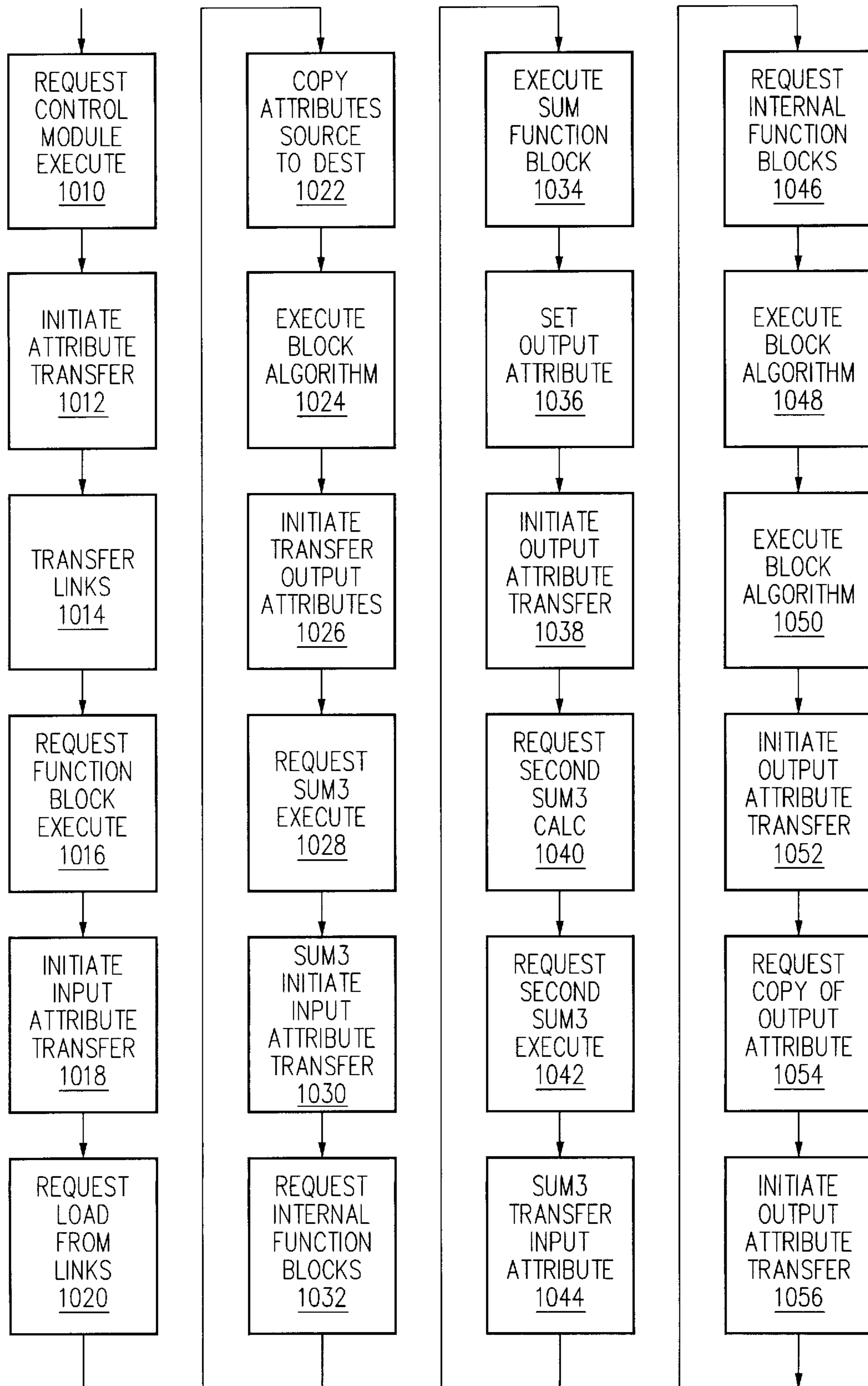
FIG. 10
