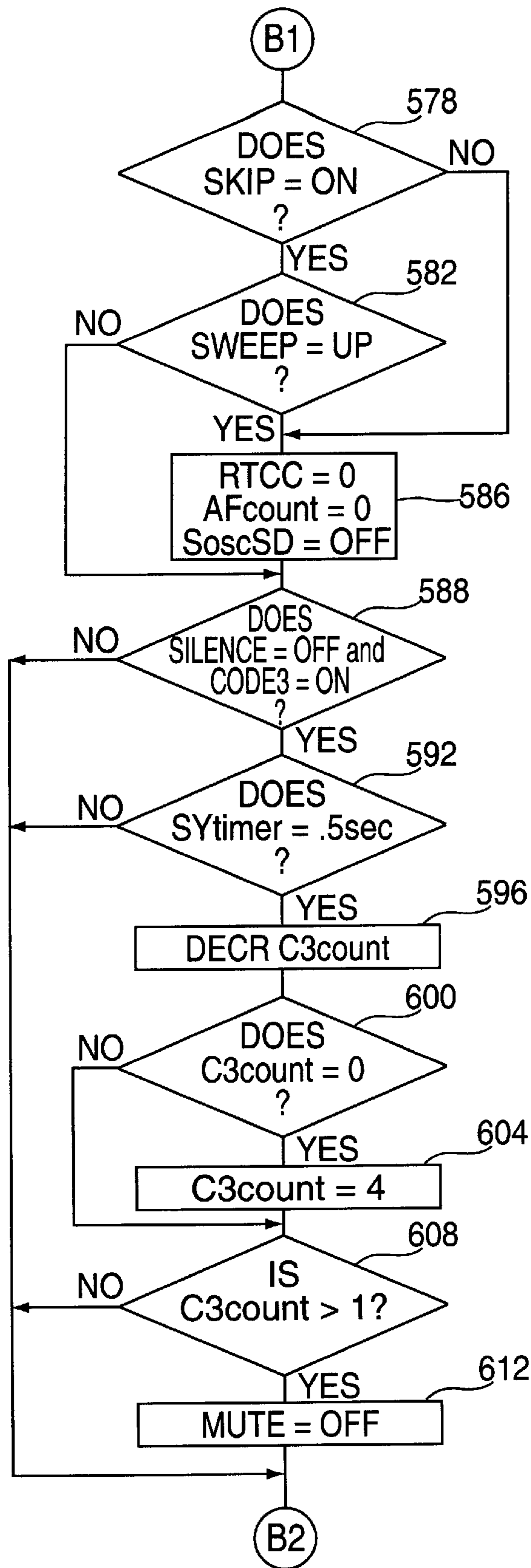
FIG. 4D
