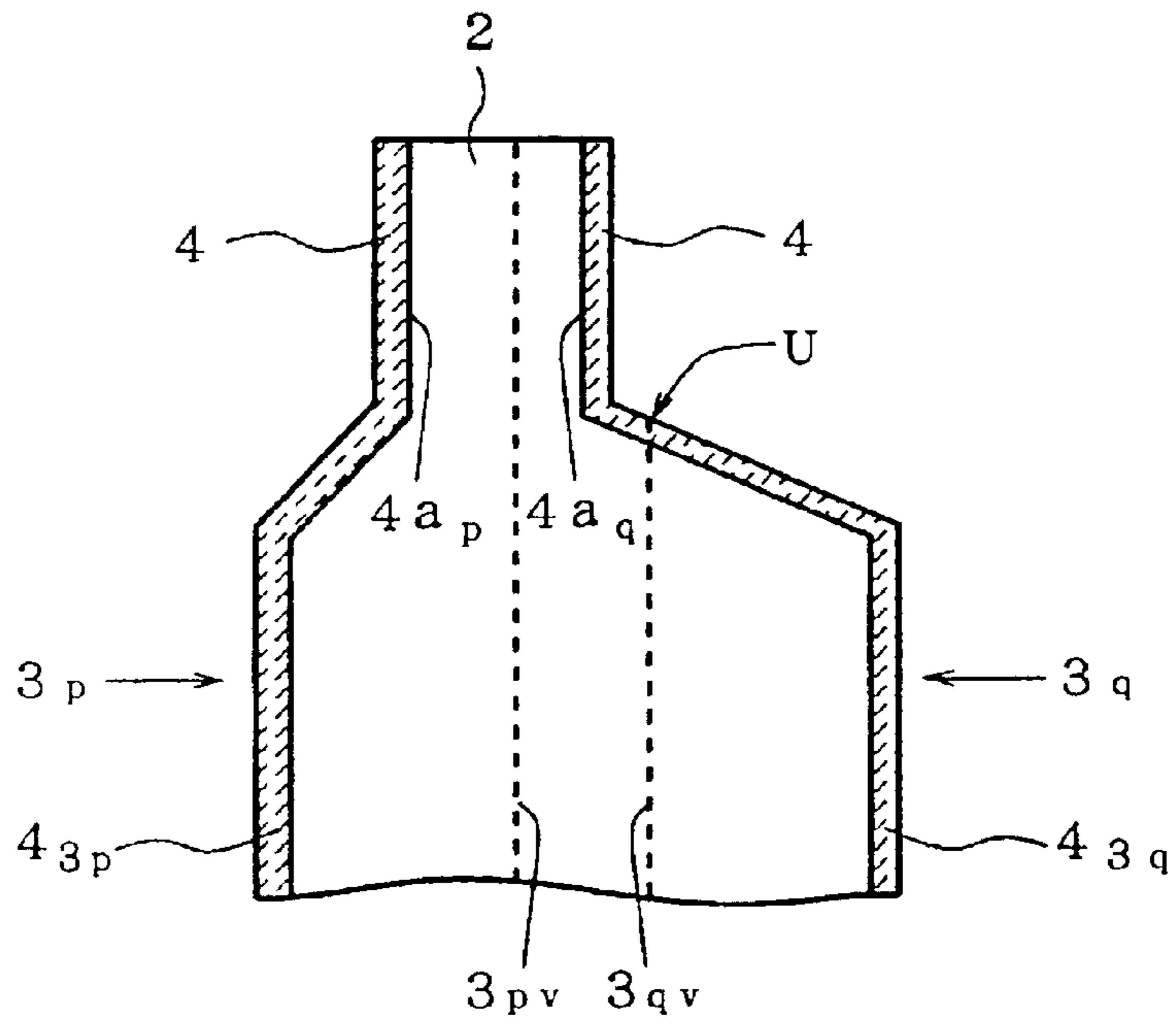
FIG. 8A
