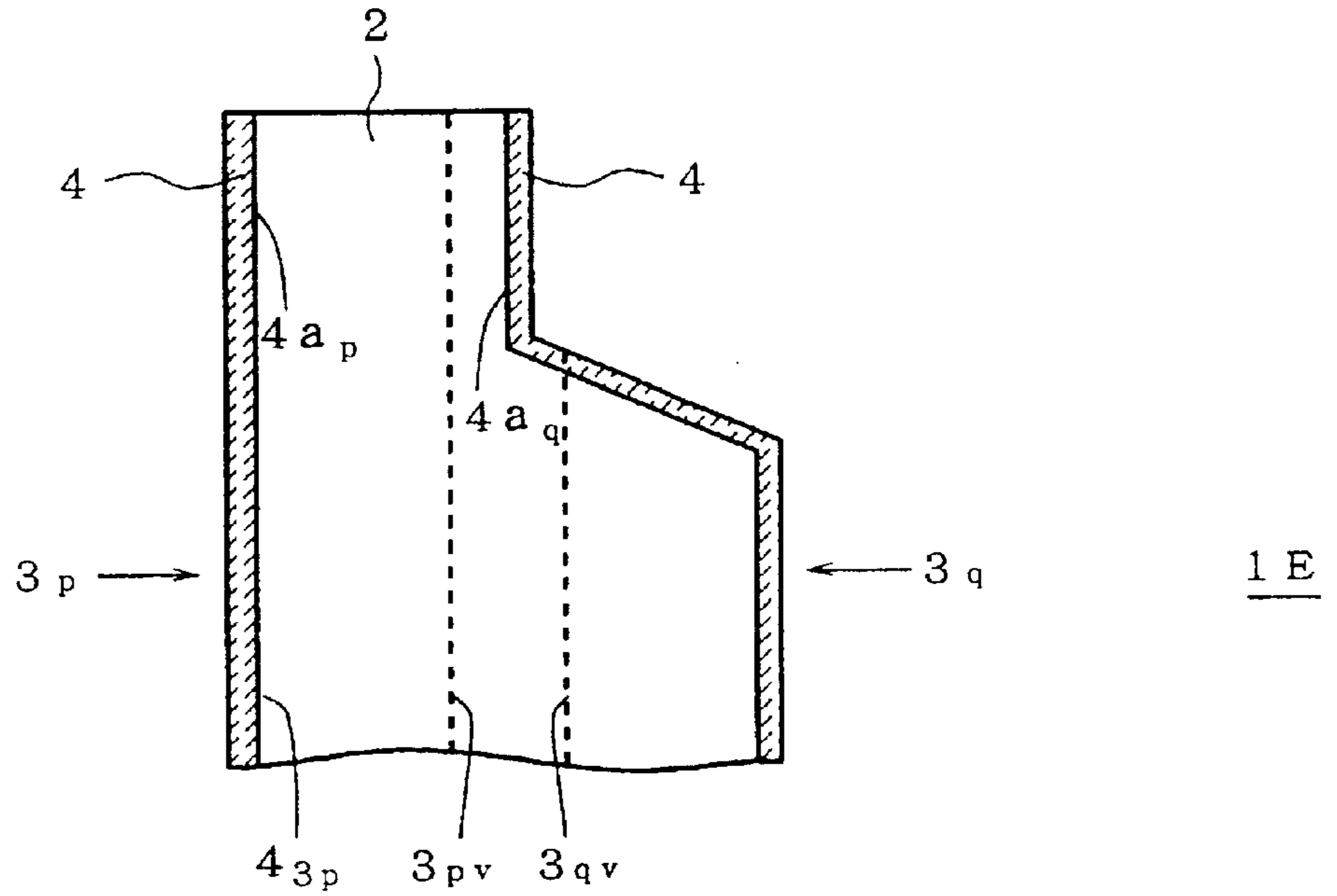
FIG. 11A
