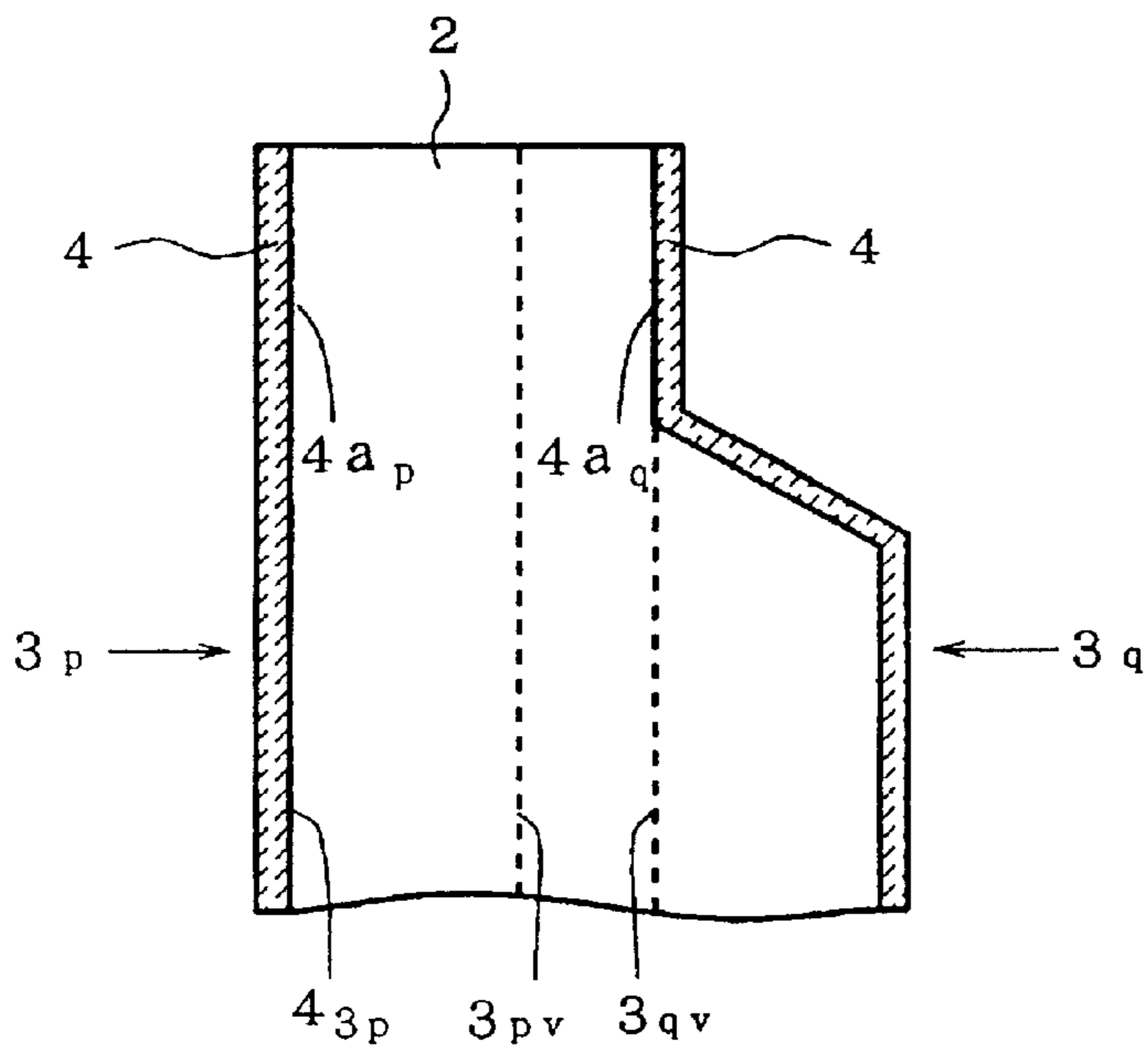
FIG. 12A
