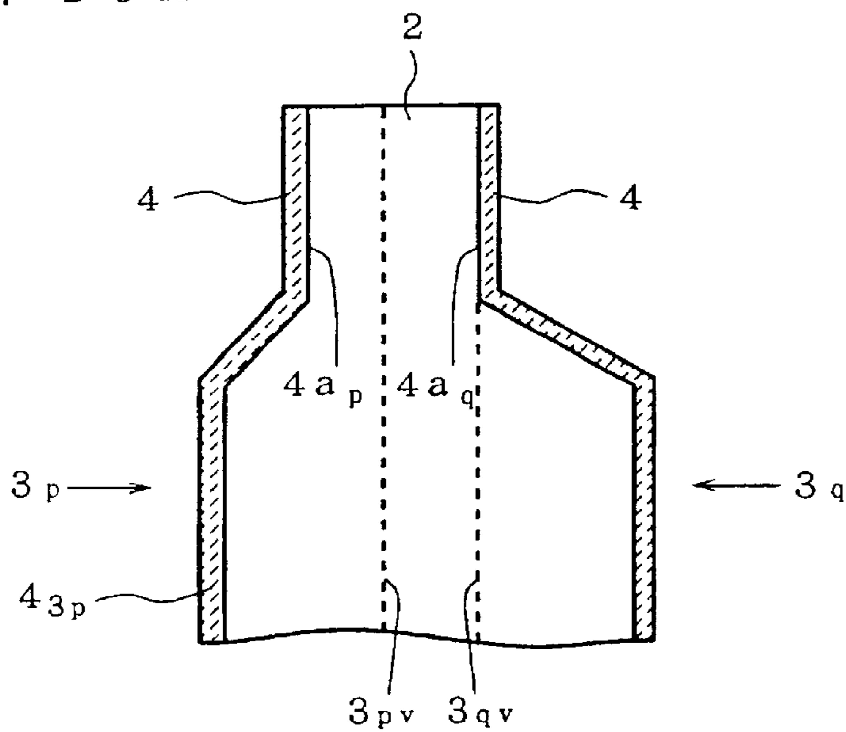
FIG. 10A
