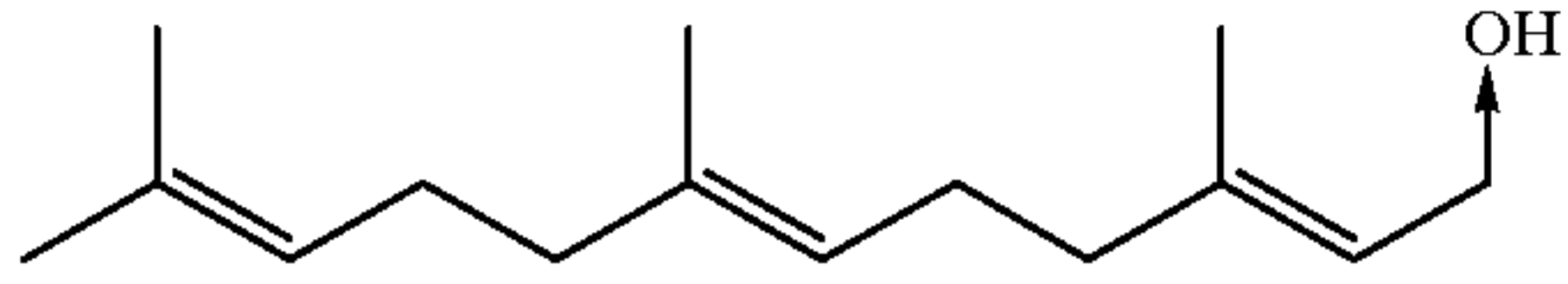
farnesol
