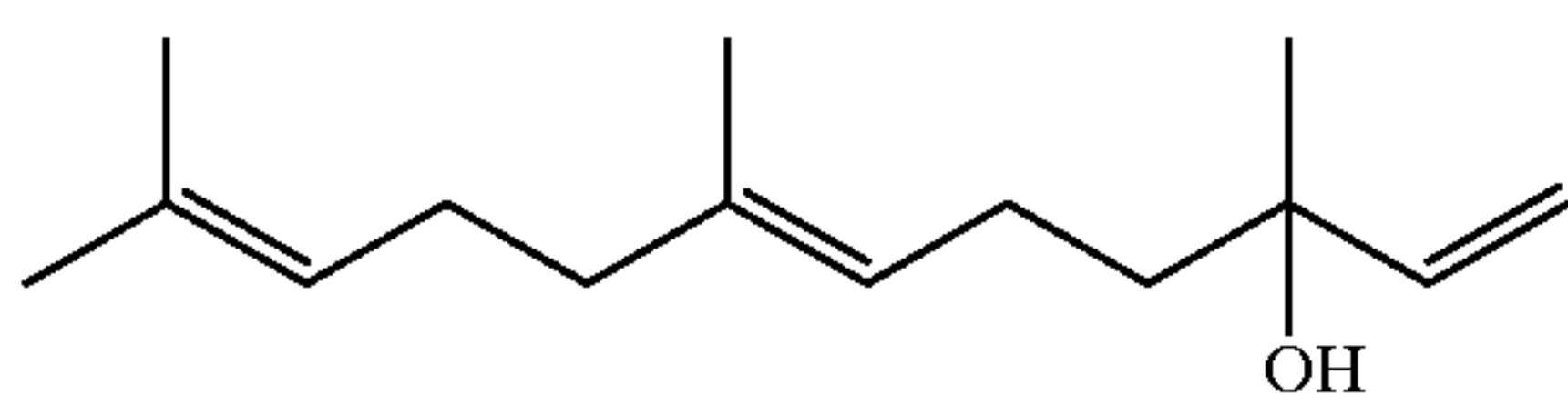
geranylgeraniol
