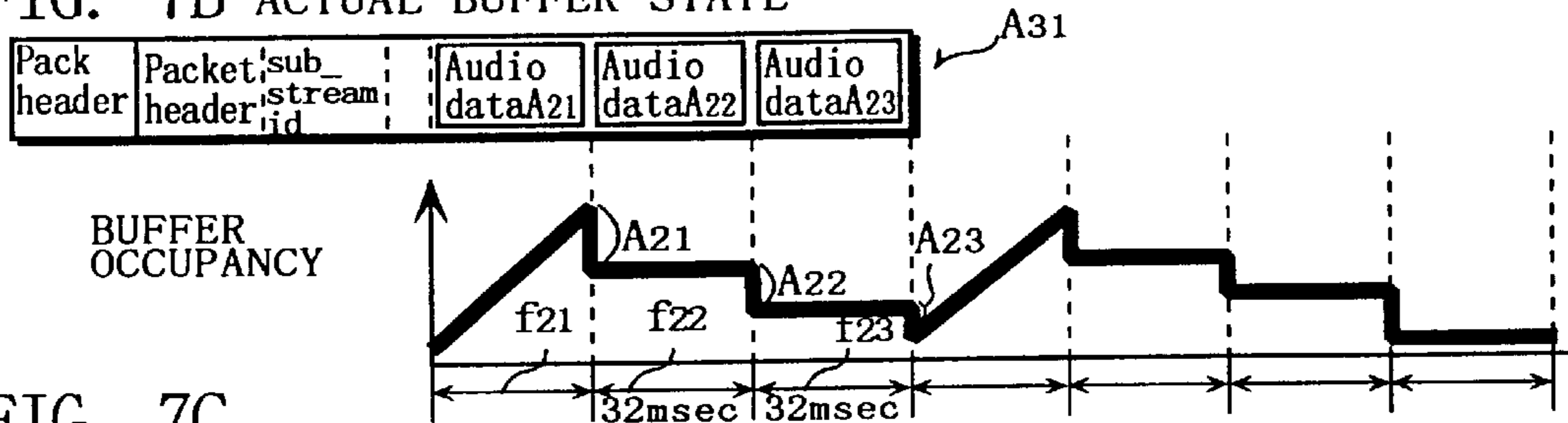
FIG. 7B ACTUAL BUFFER STATE
