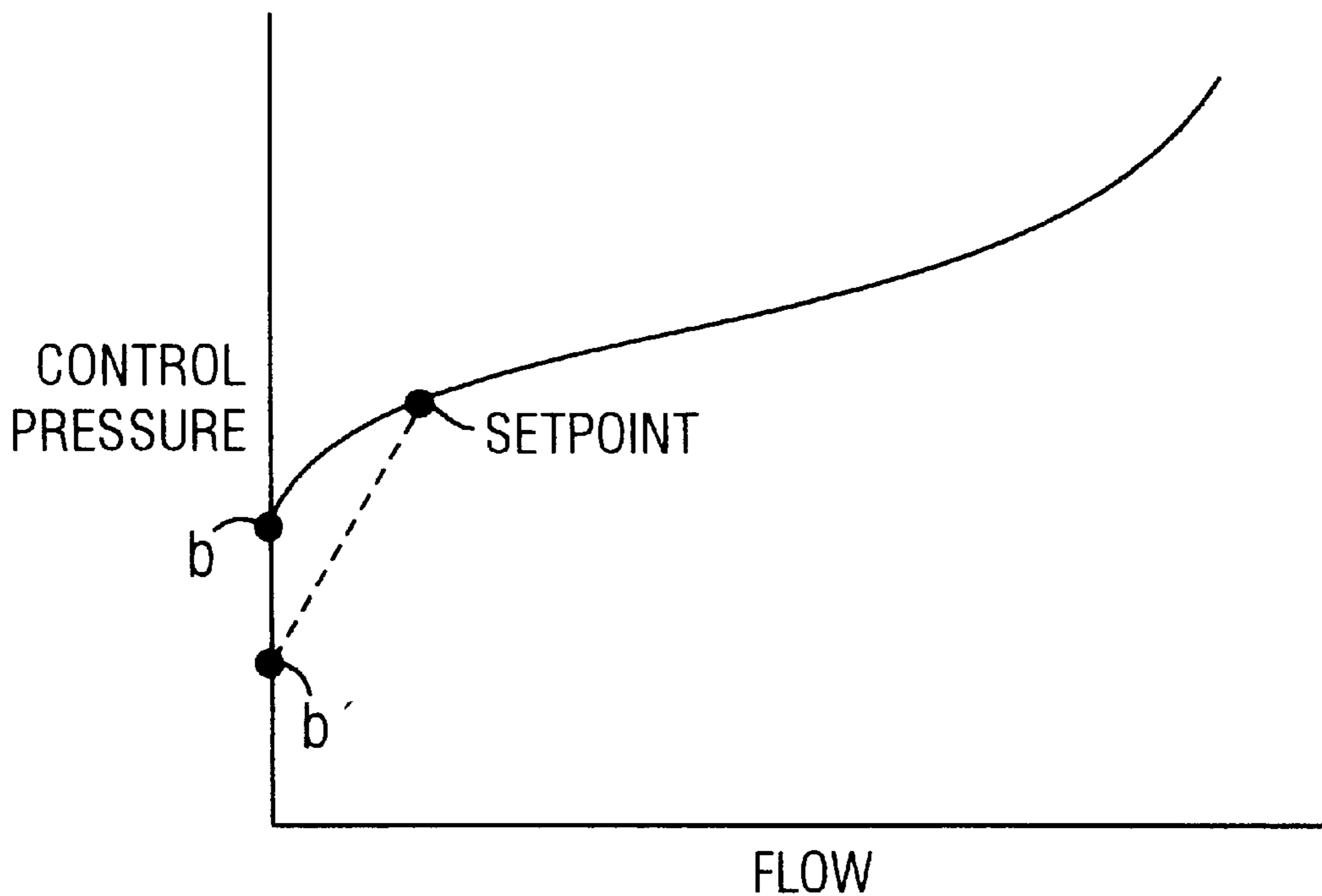
FIG. 11B
