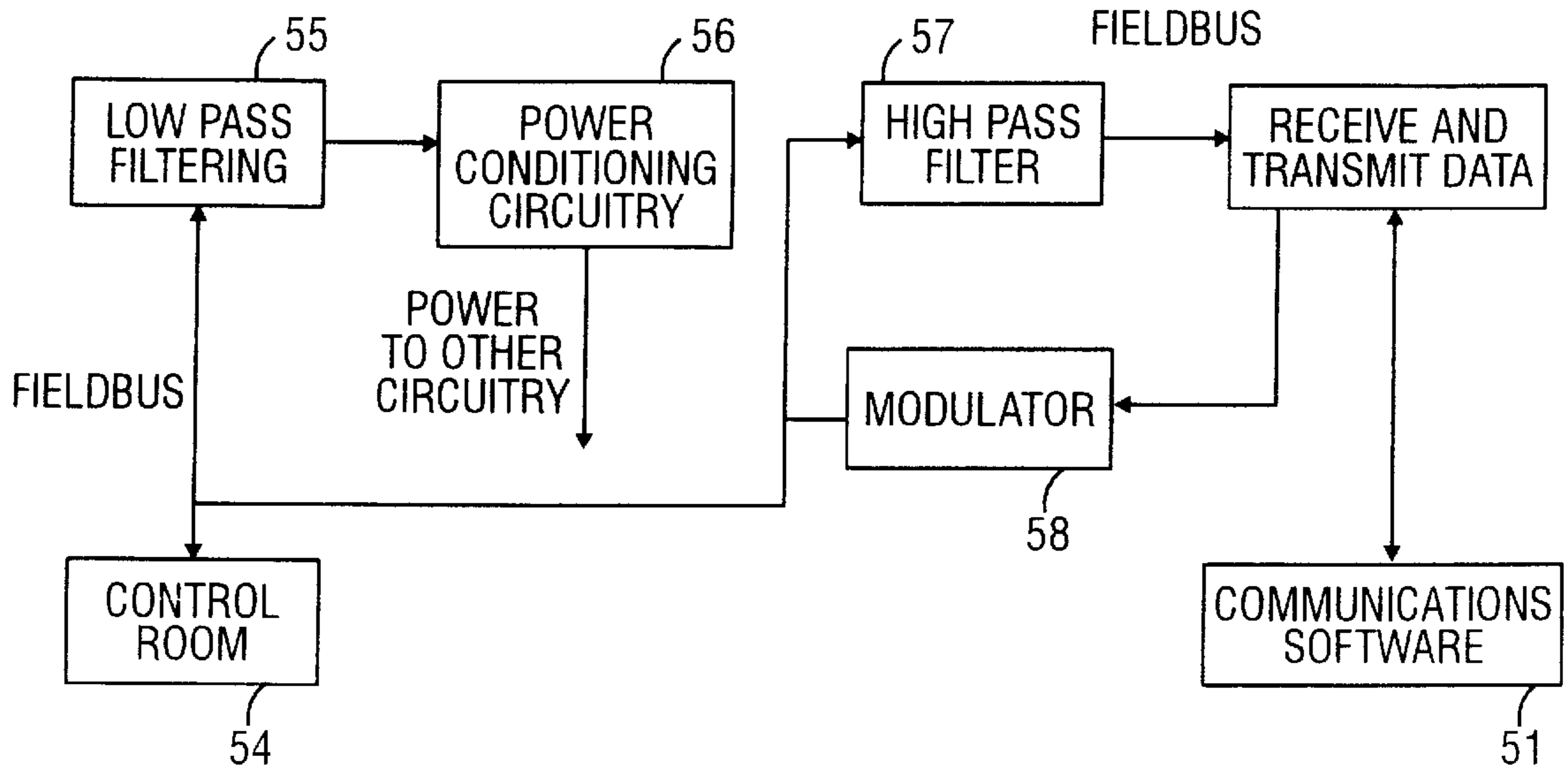
FIG. 12
