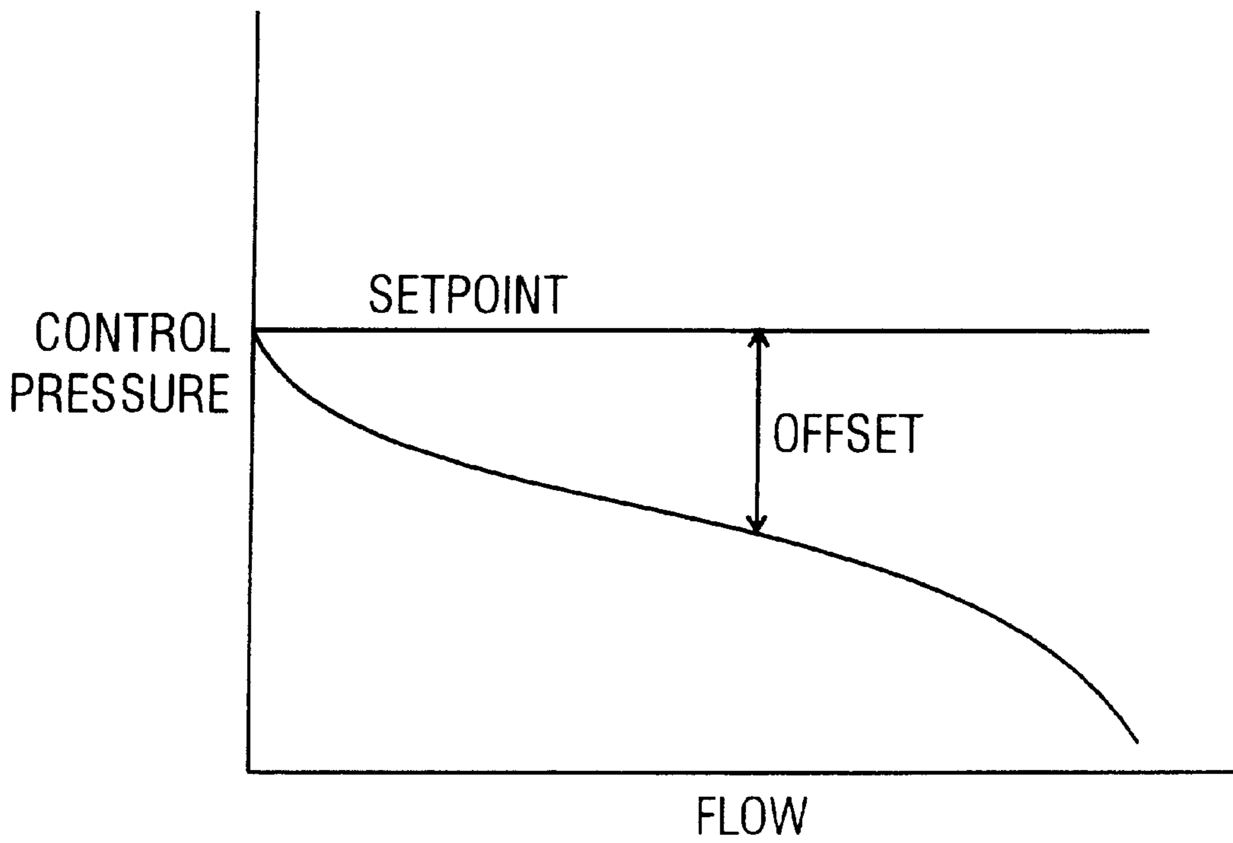
FIG. 8A
