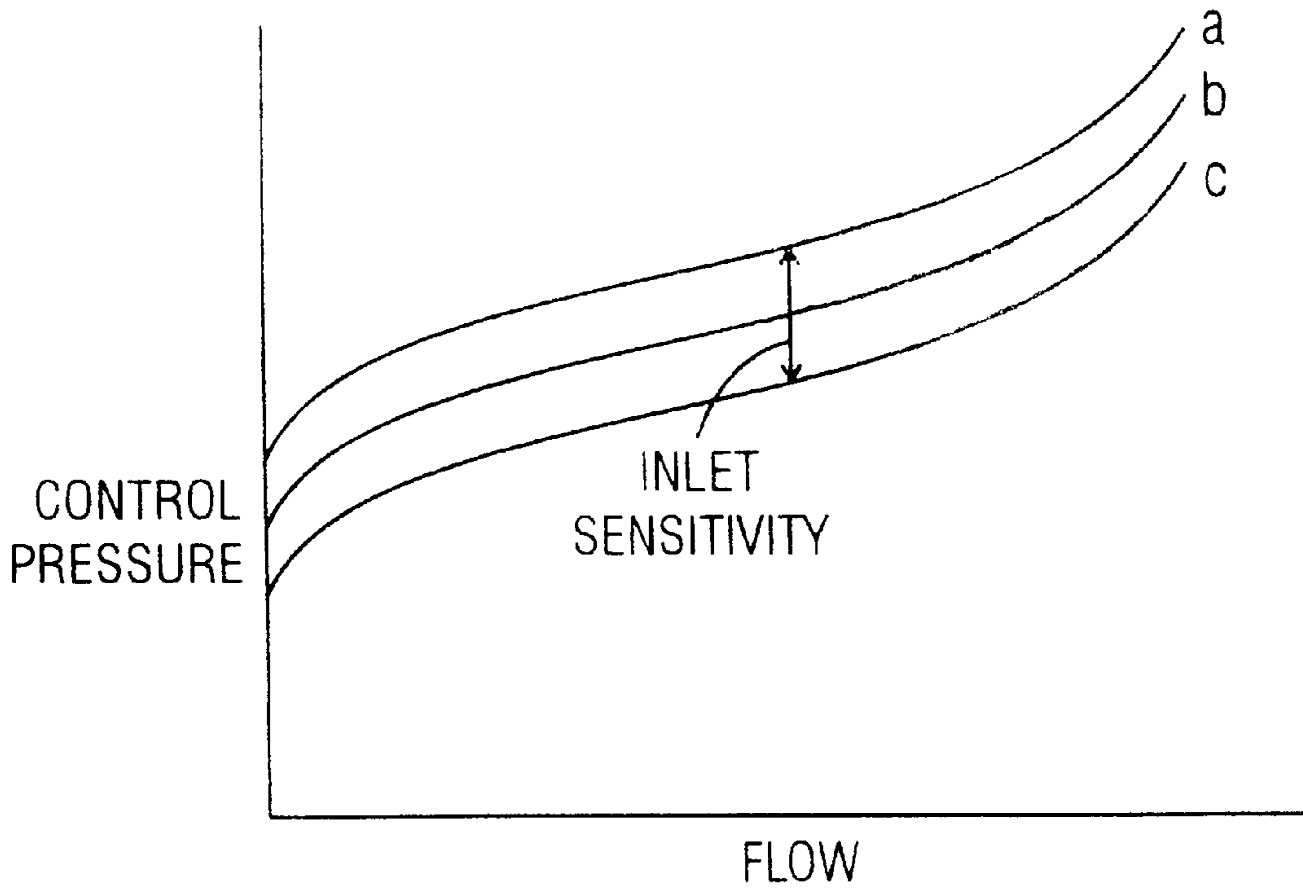
FIG. 9B
