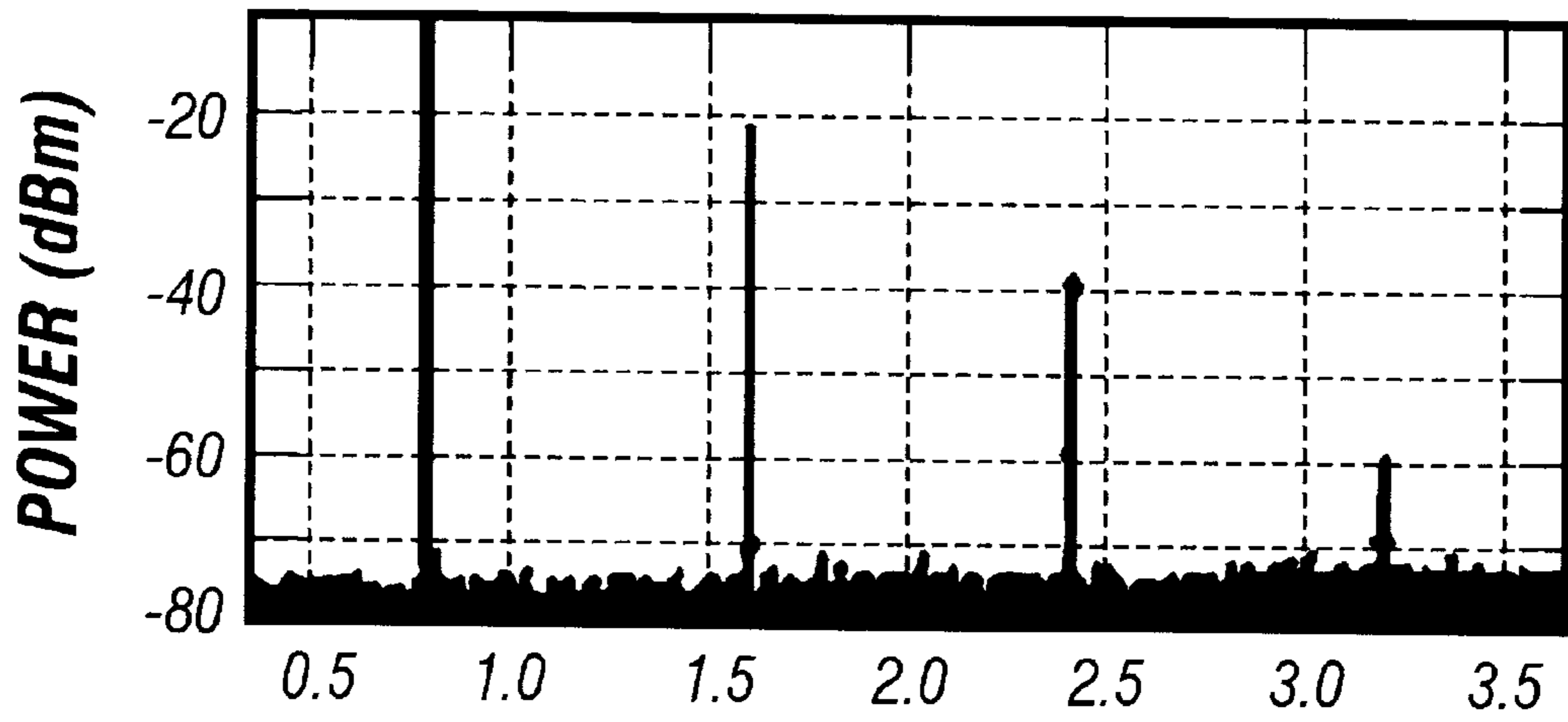
FREQUENCY (GHz) FIG. 9E
