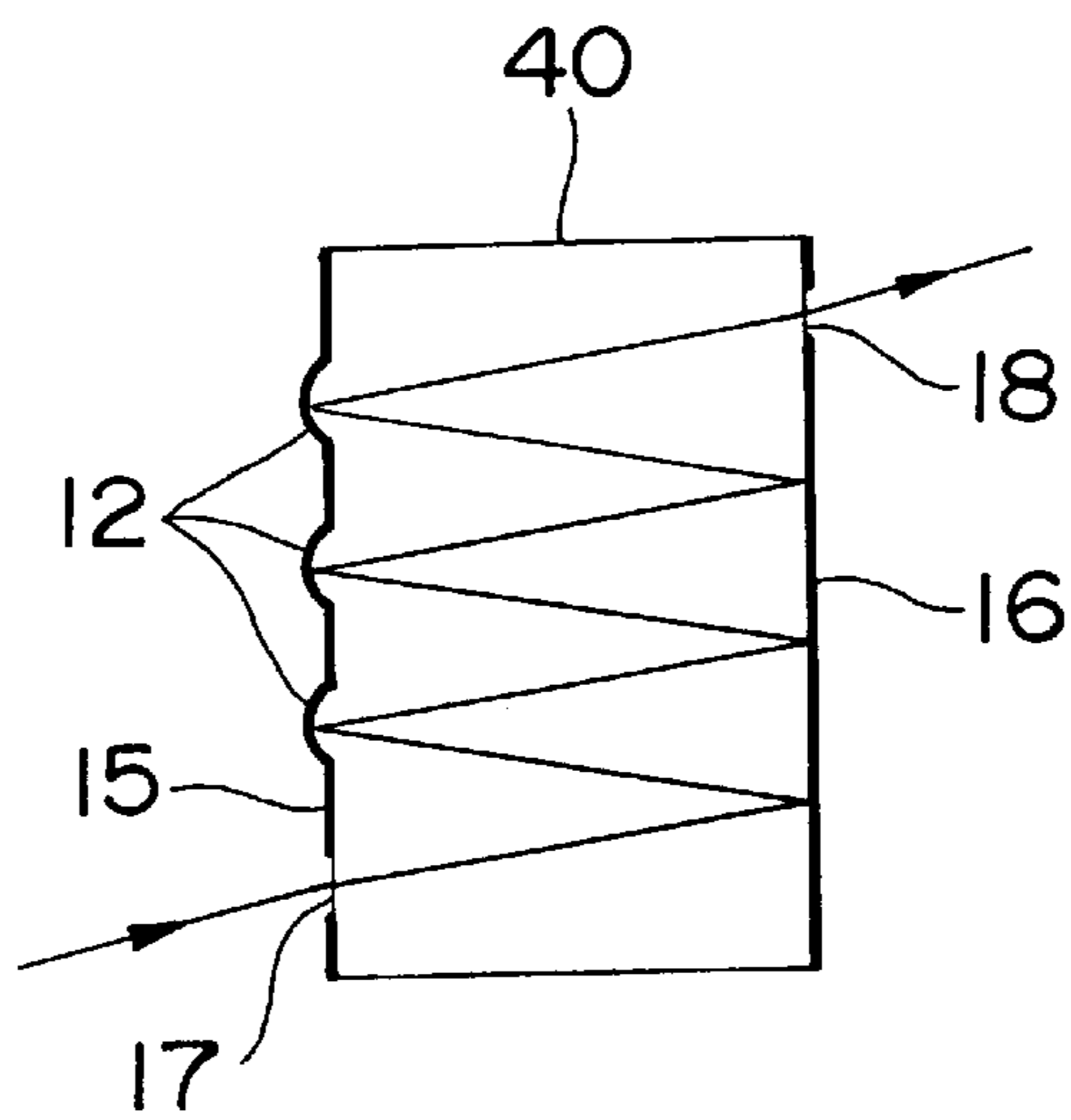
FIG.20
