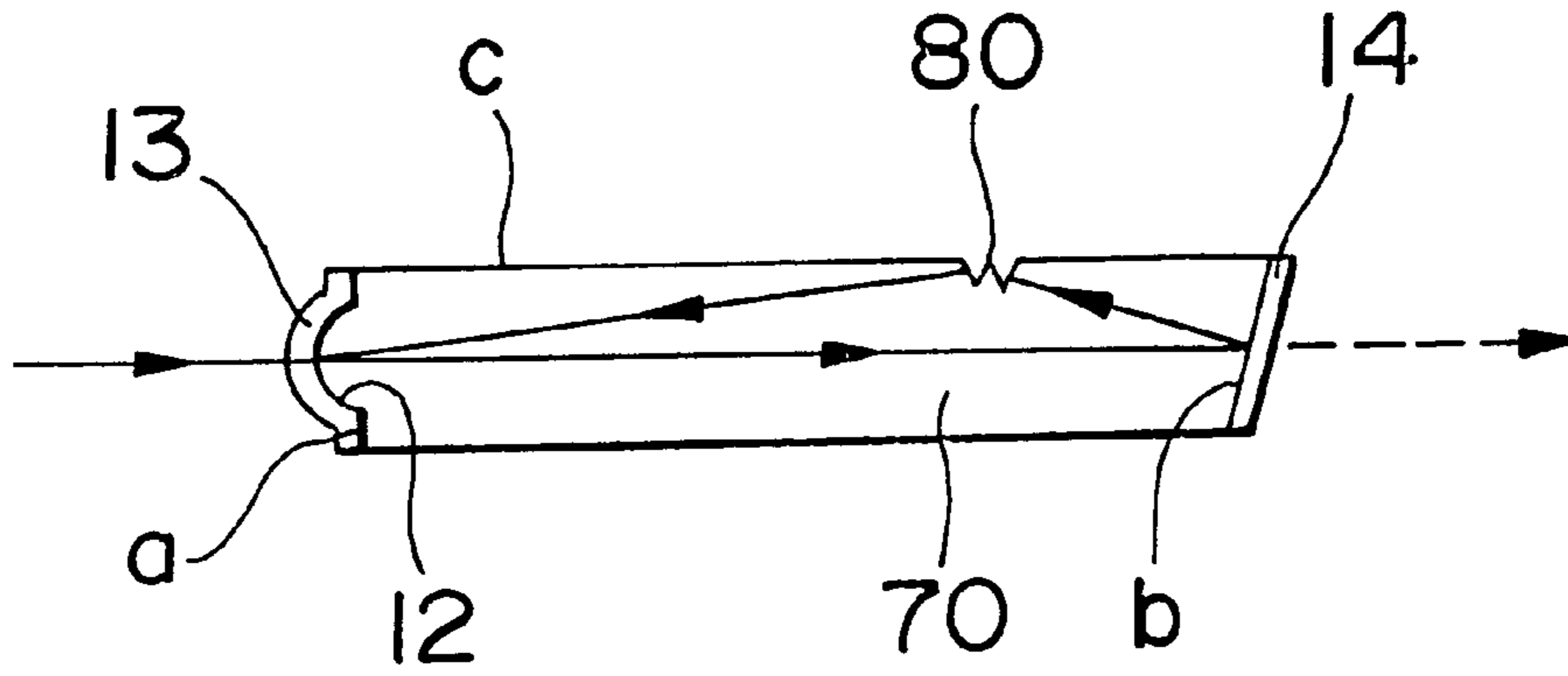
FIG.17
