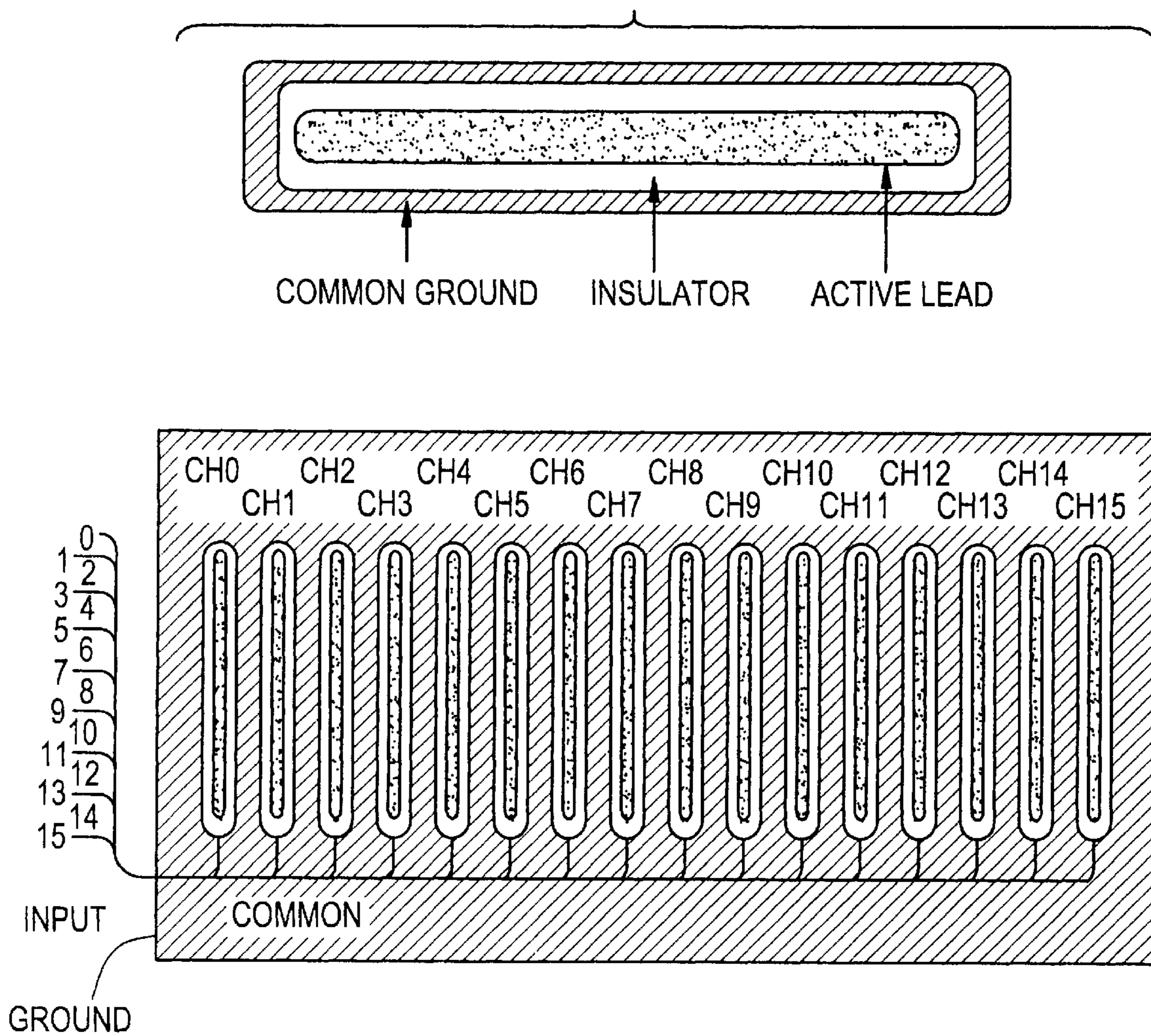
FIG. 7 ANALOG PROBE
