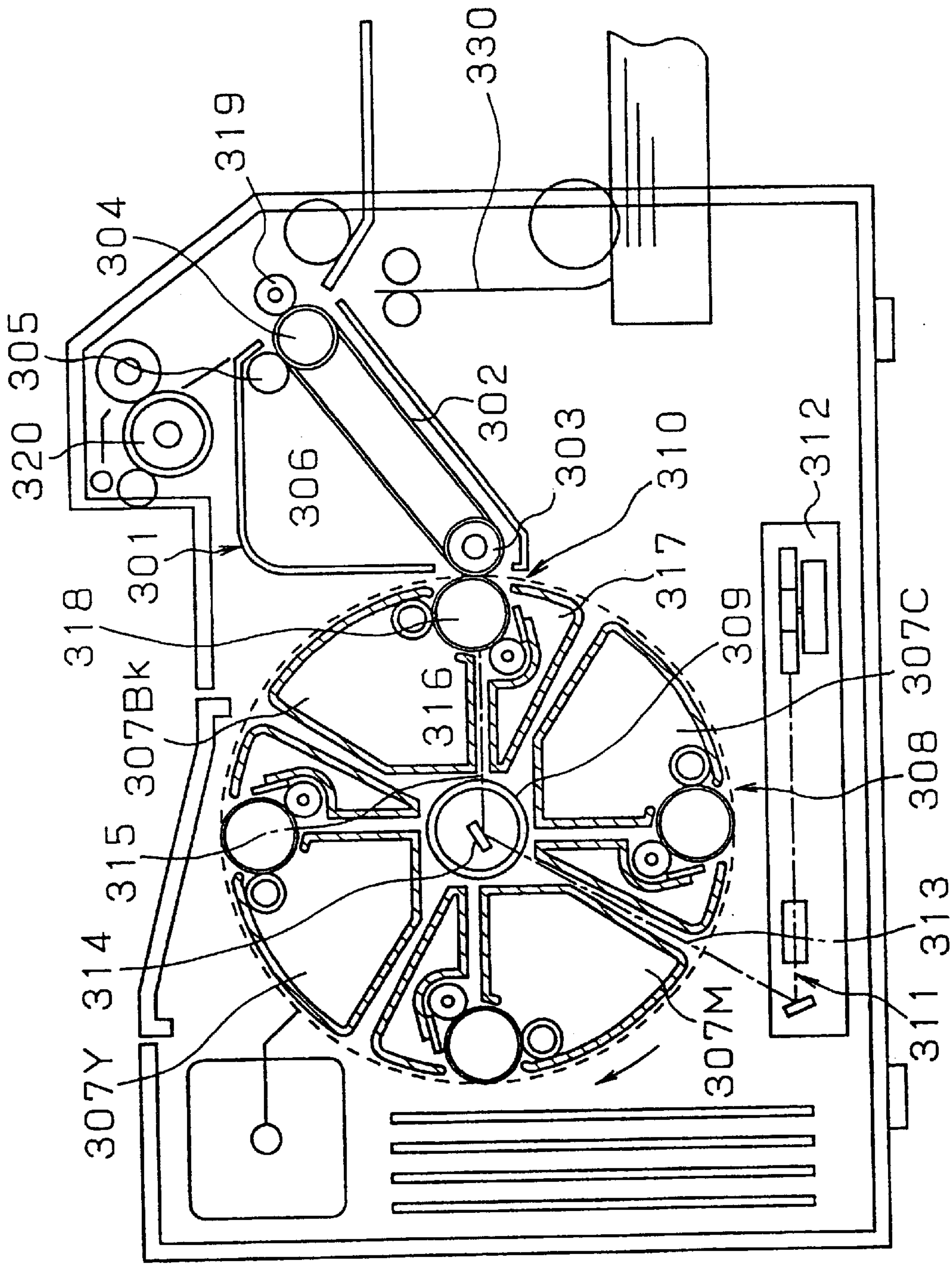
FIG. 20(PRIOR ART)
