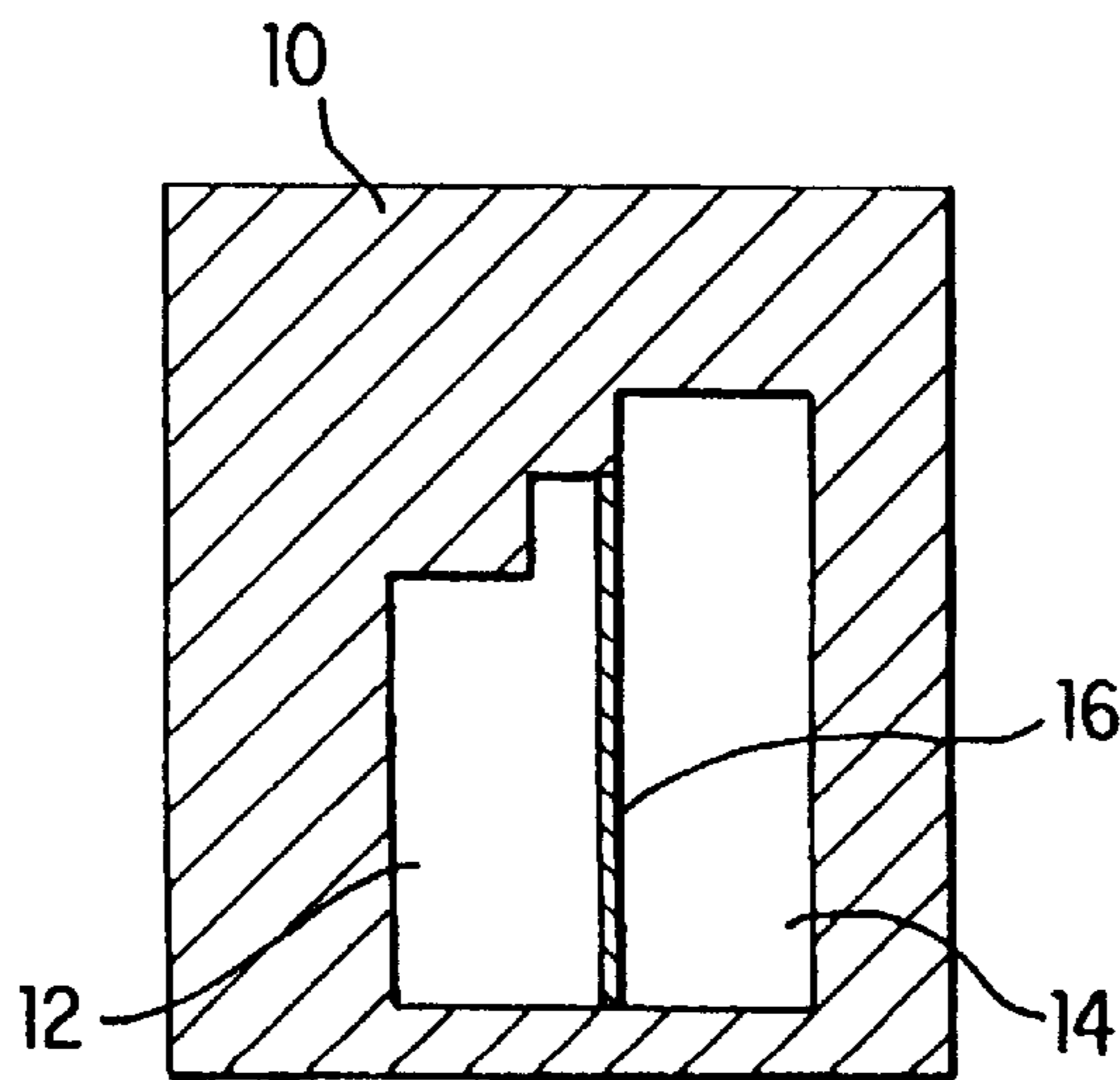
FIG. 2 --PRIOR ART--
