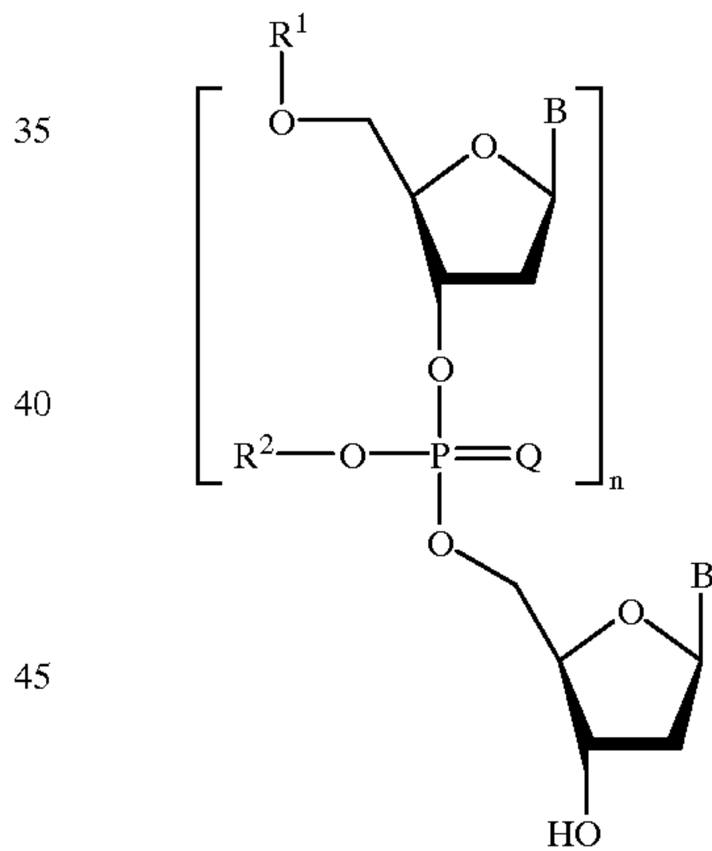
XVIIIa
