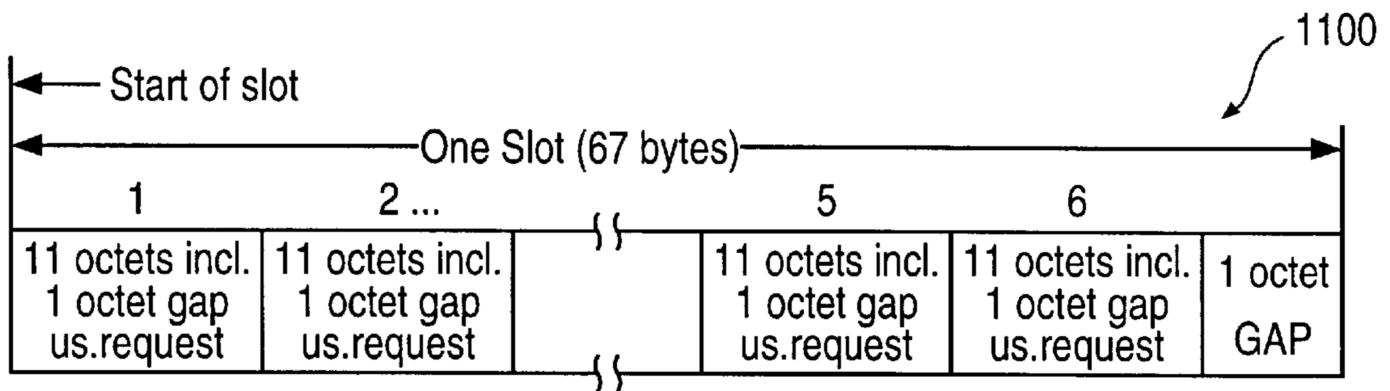
FIG. 11
