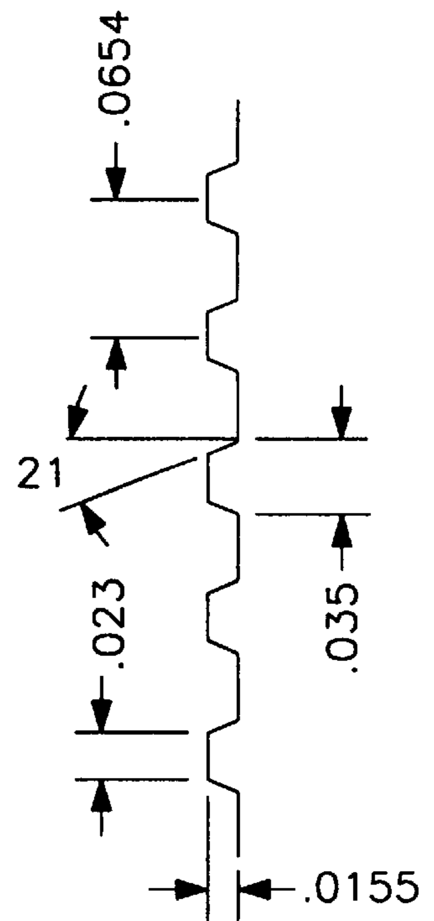
FIG. 4A-3
