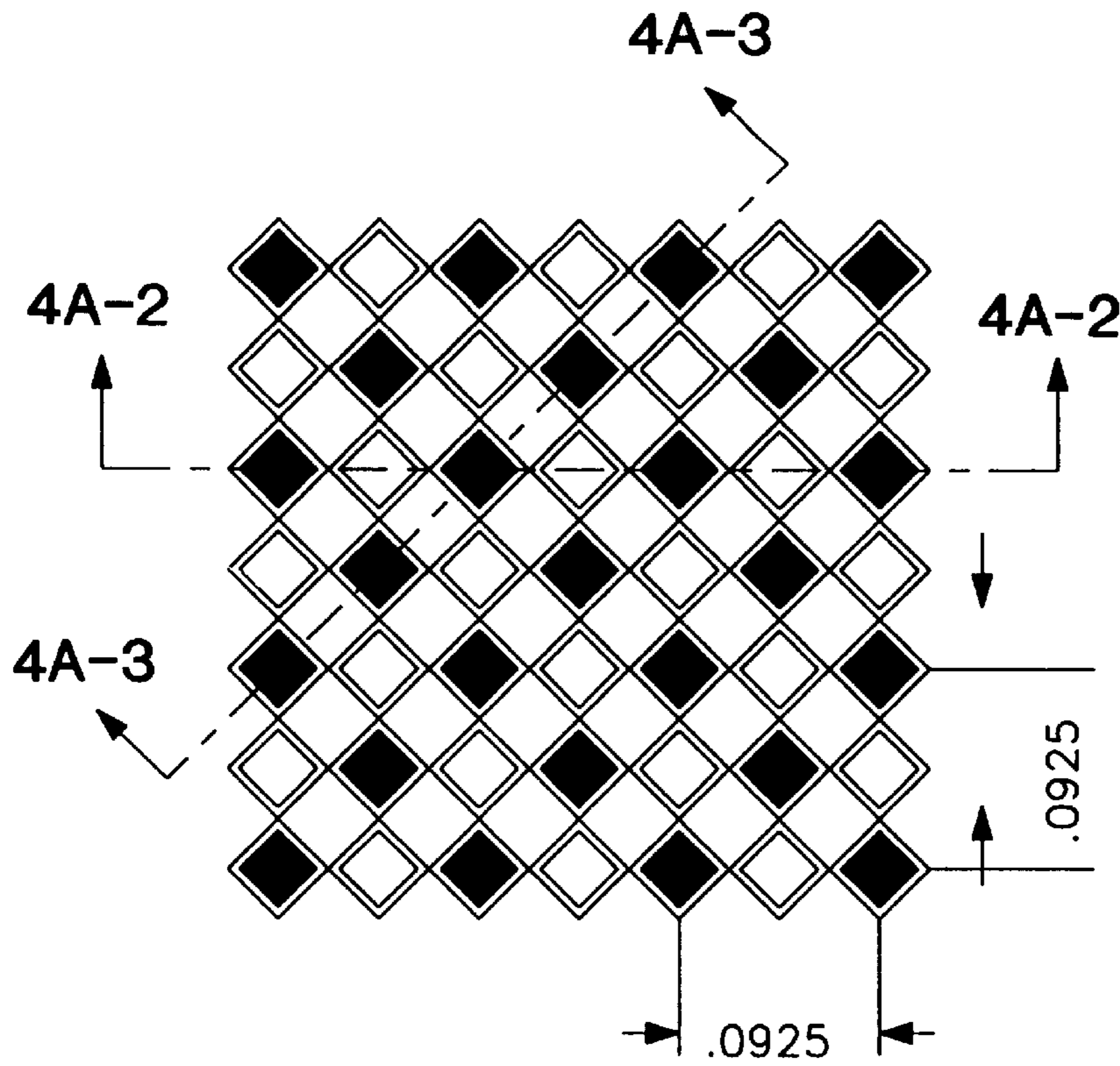
FIG. 4A-1
