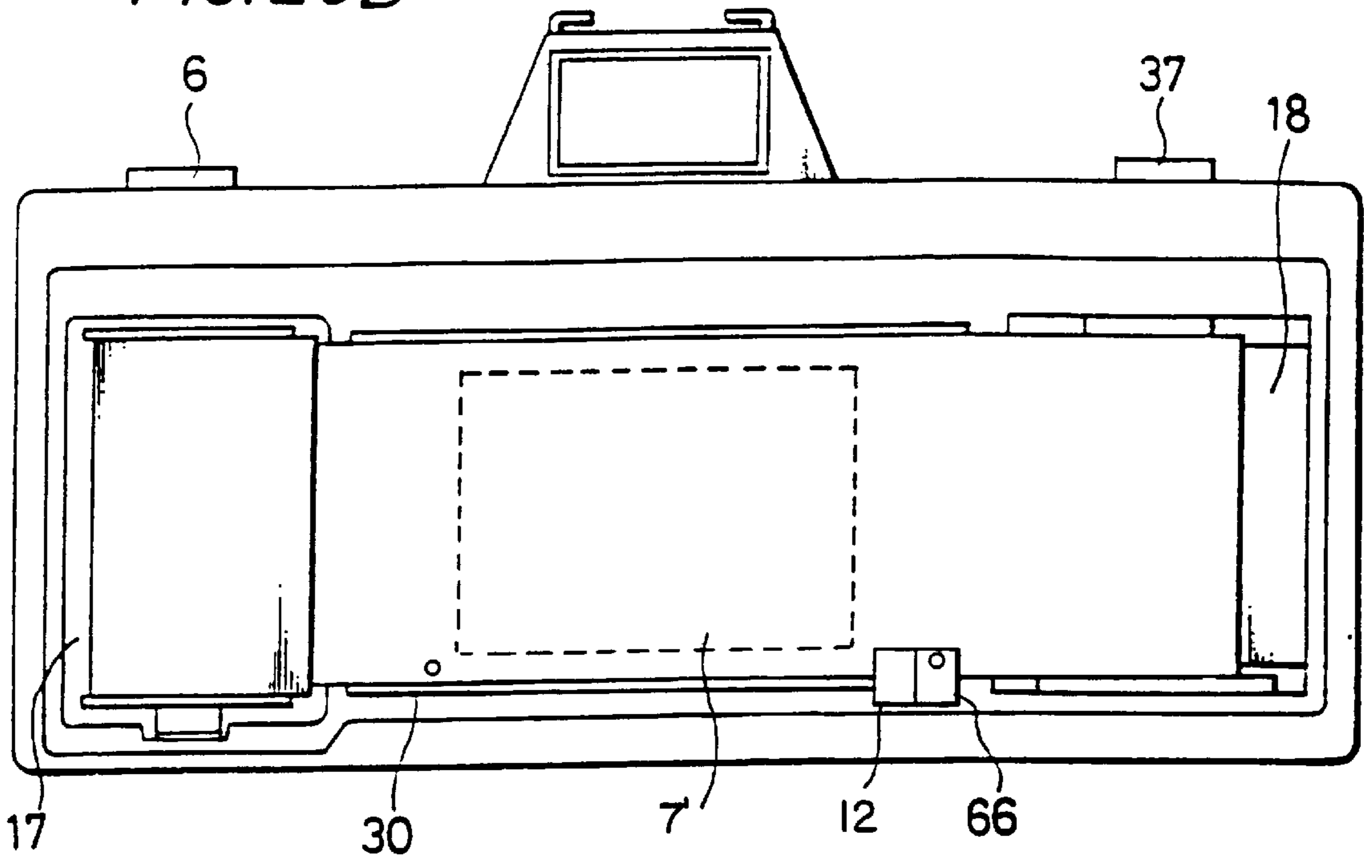
FIG. 20B
