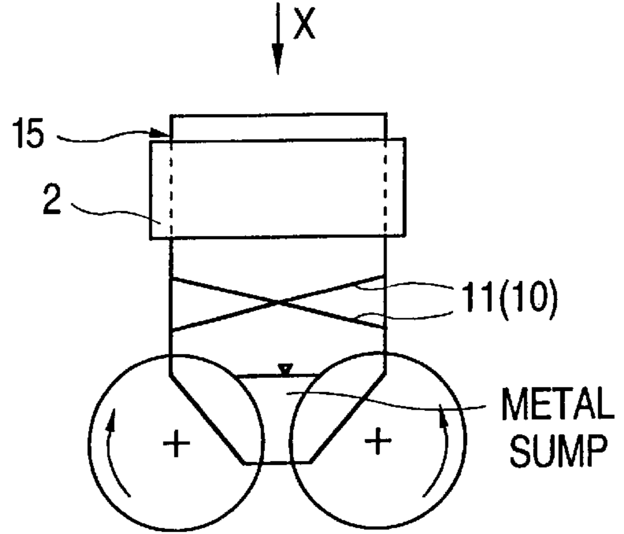
FIG. 4b
