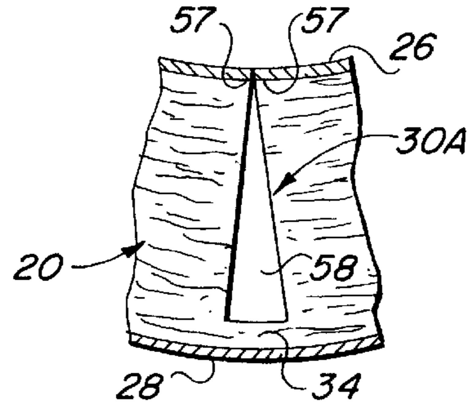
FIG. 6A
