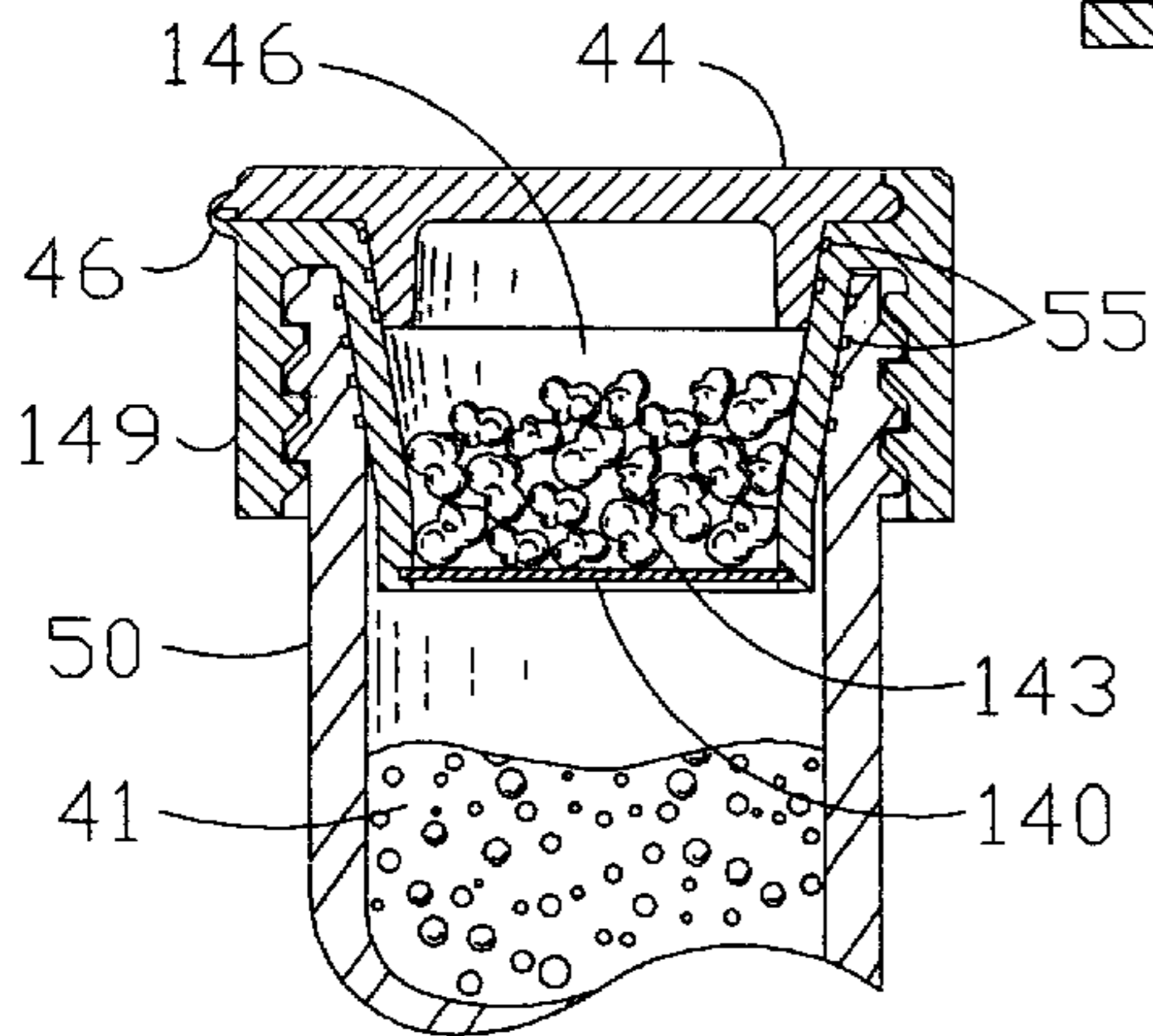
FIG. 20A
