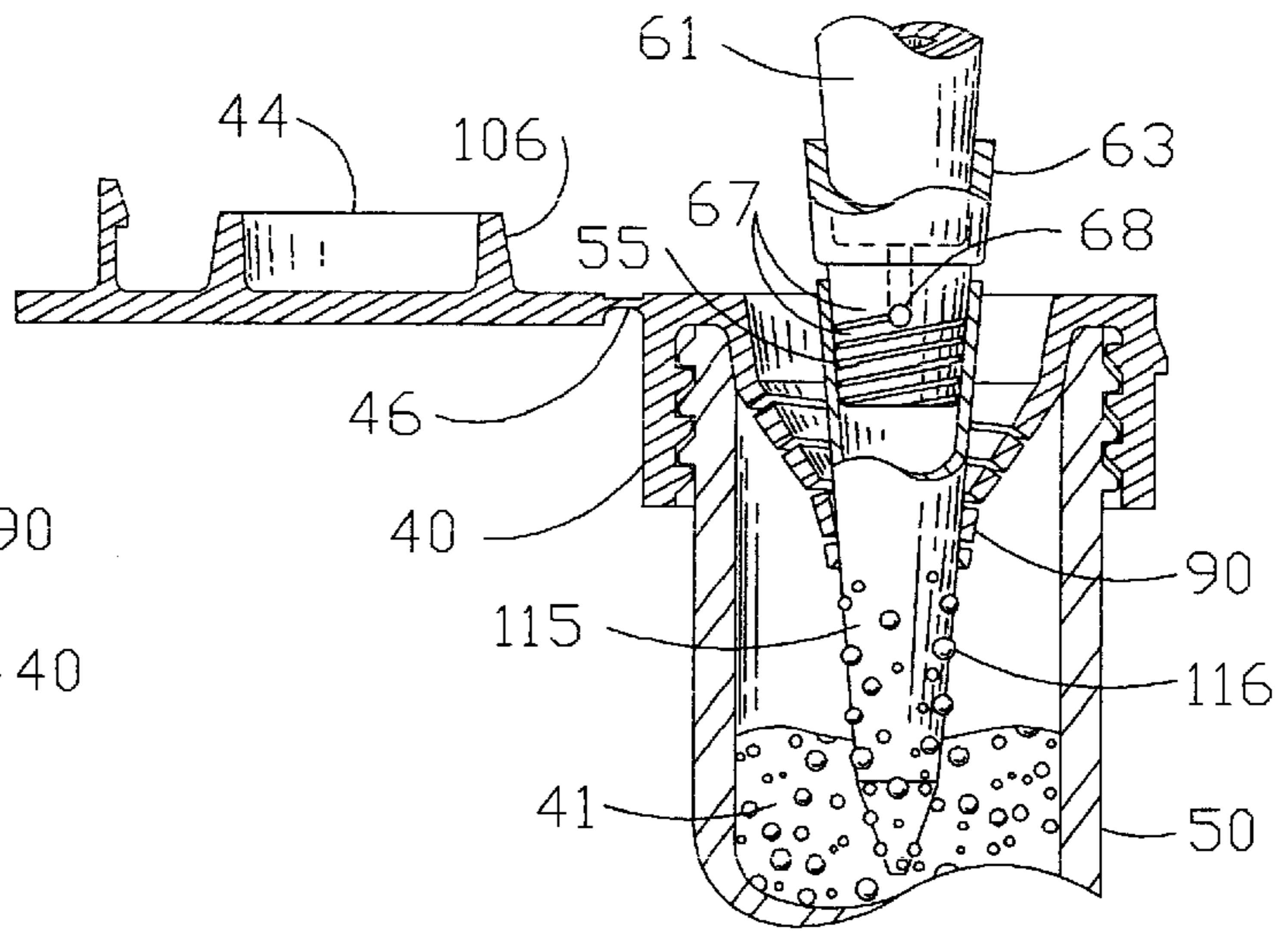
FIG. 16
