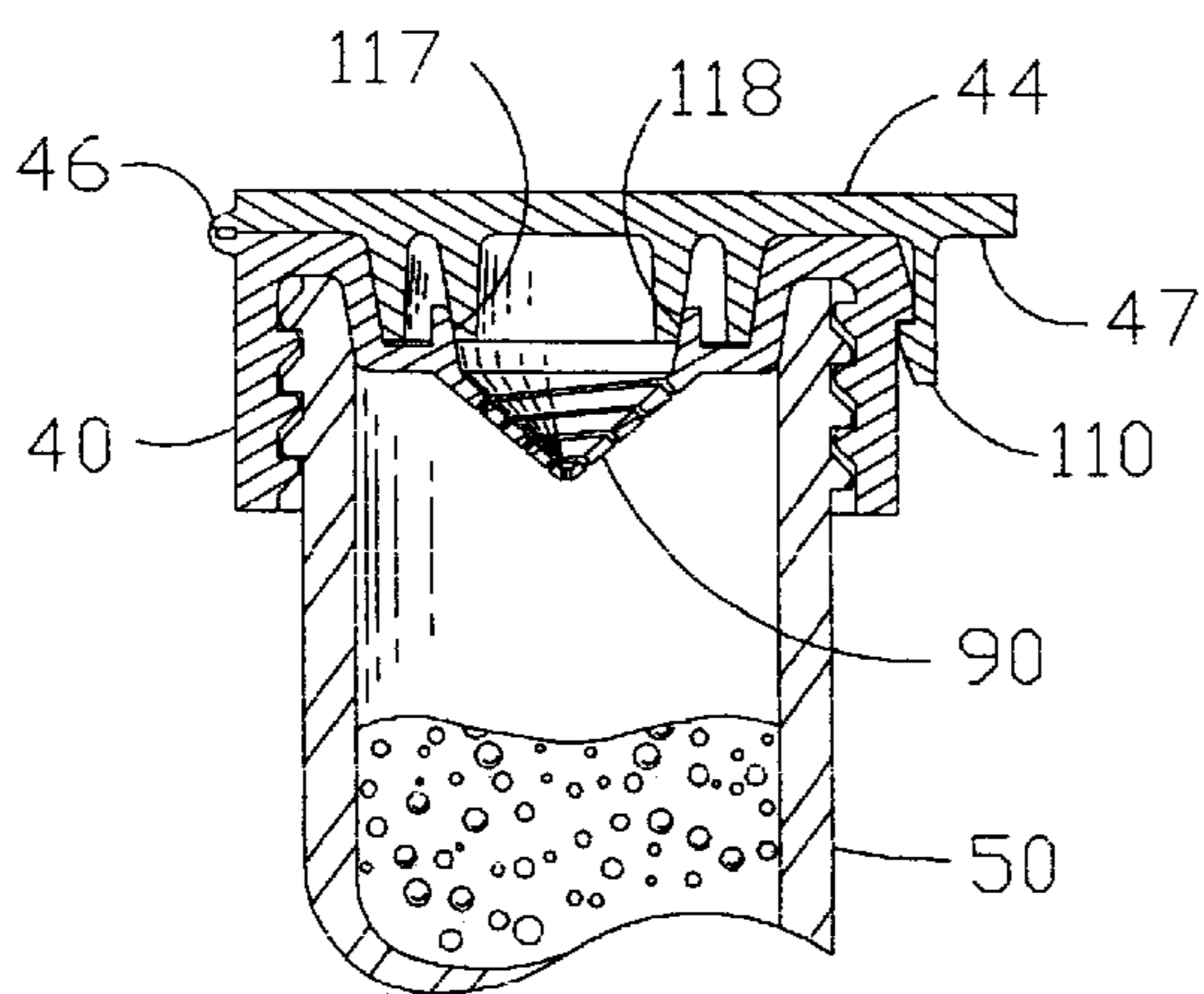
FIG. 18
