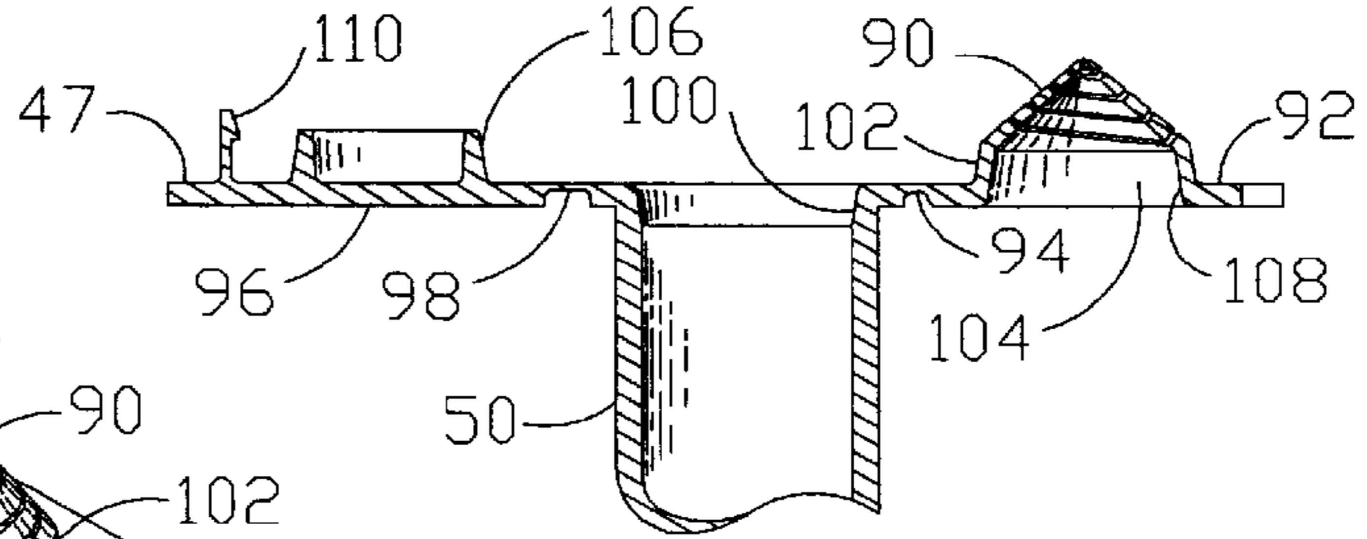
FIG. 12A
