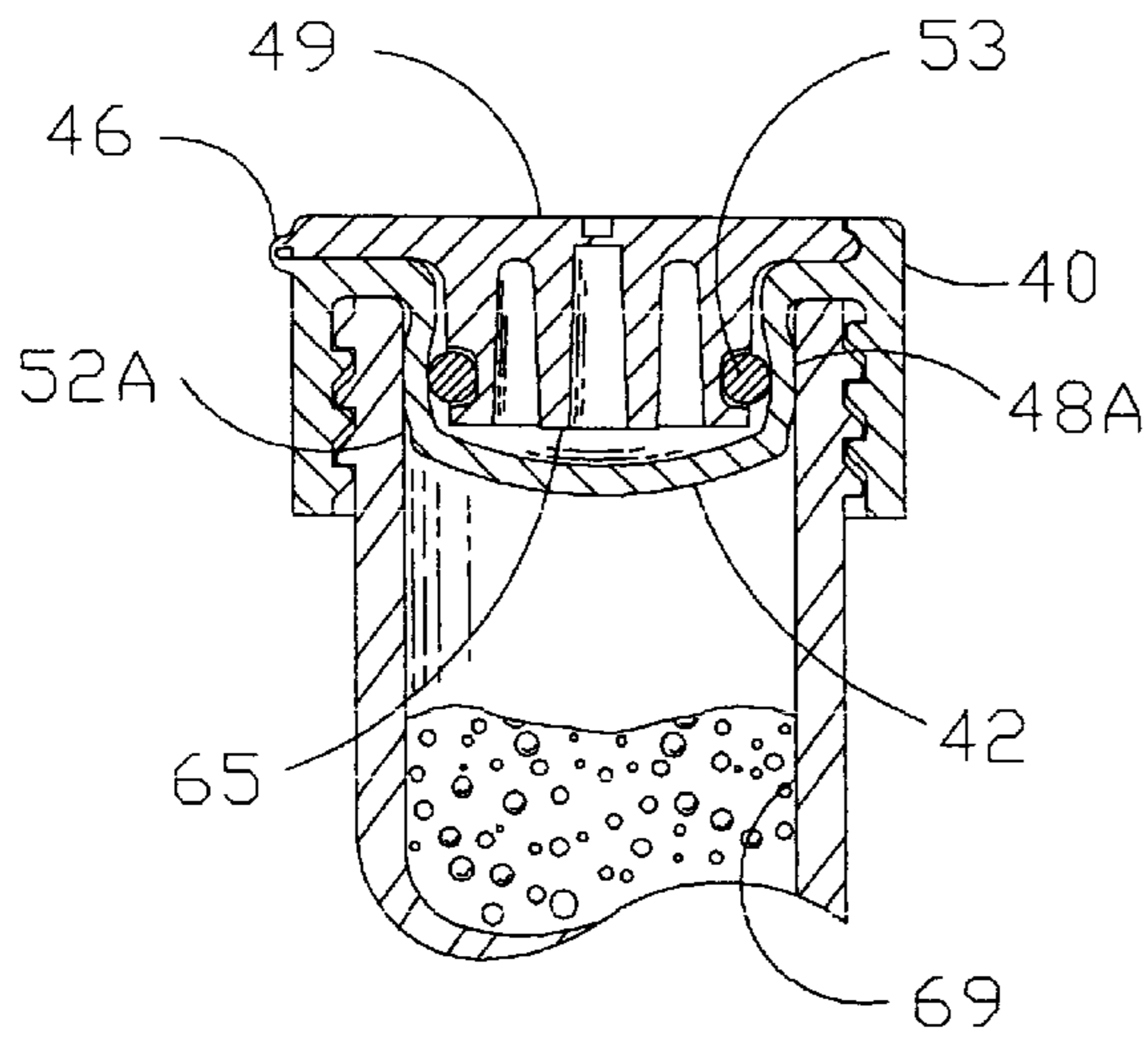
FIG 4B
