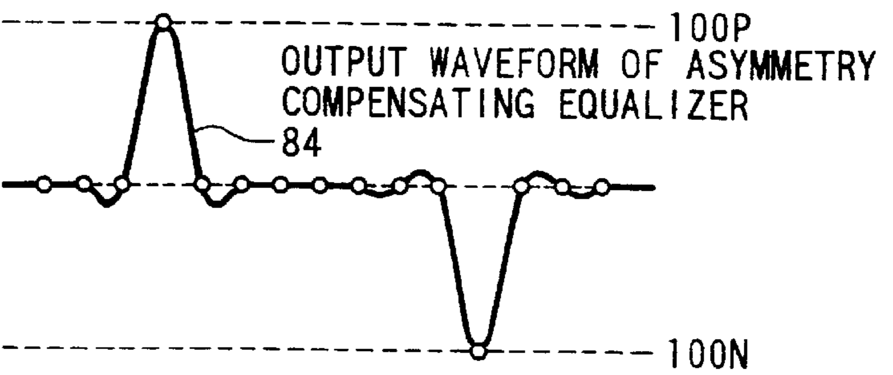
FIG. 14(D)
