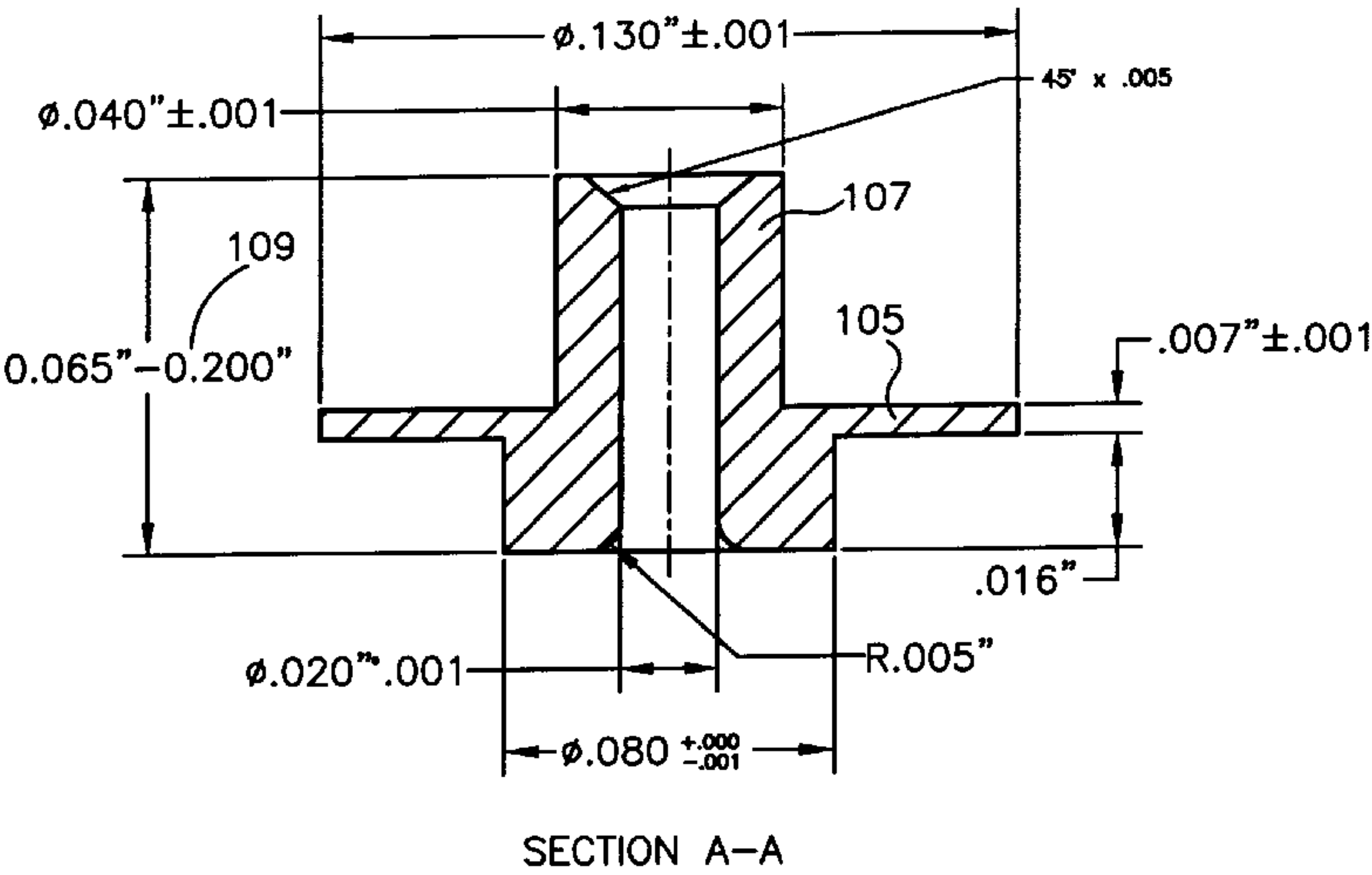
SECTION A-A FIG. 28(c)
