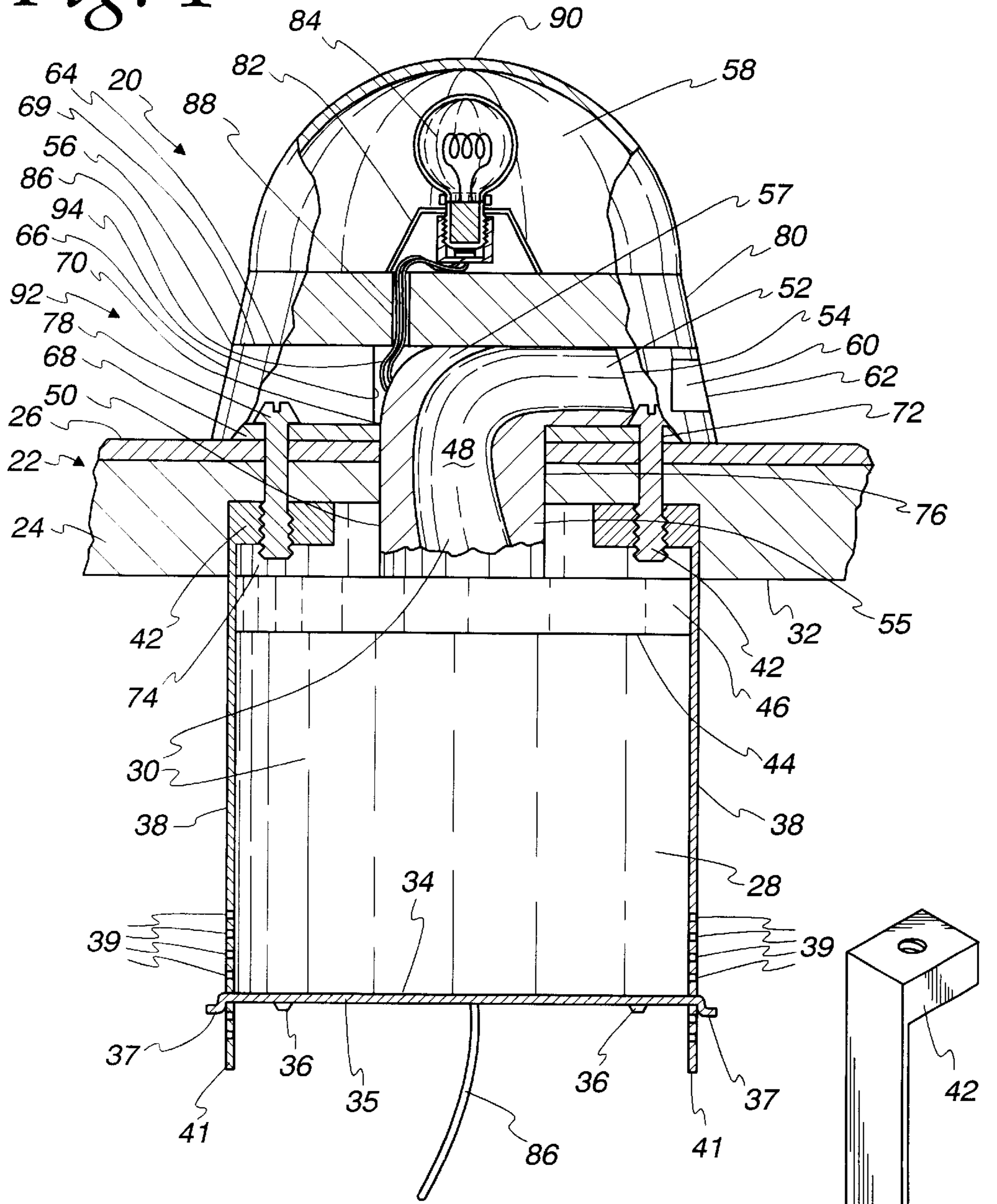
Fig. 1a
