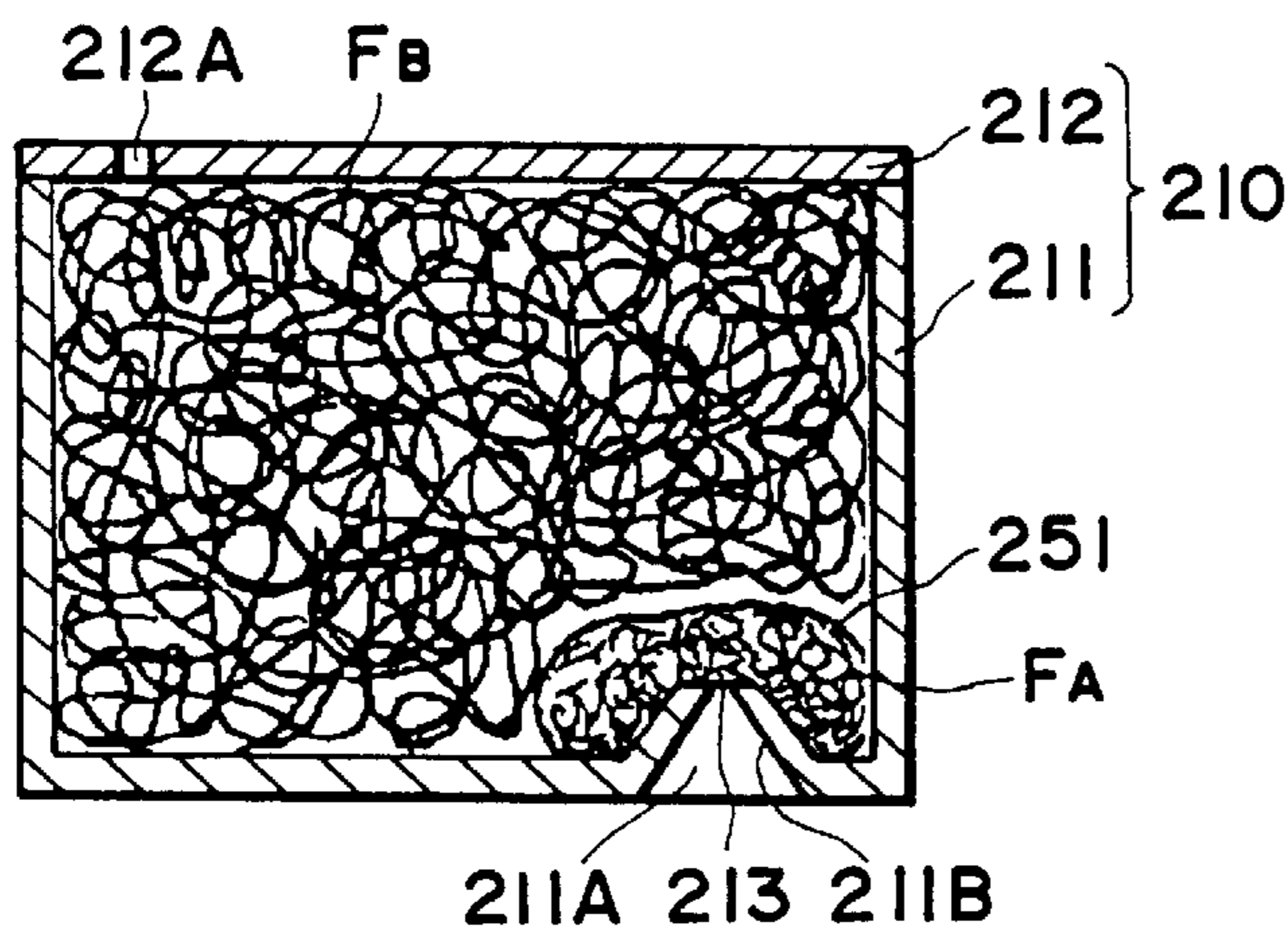
FIG. 21C
