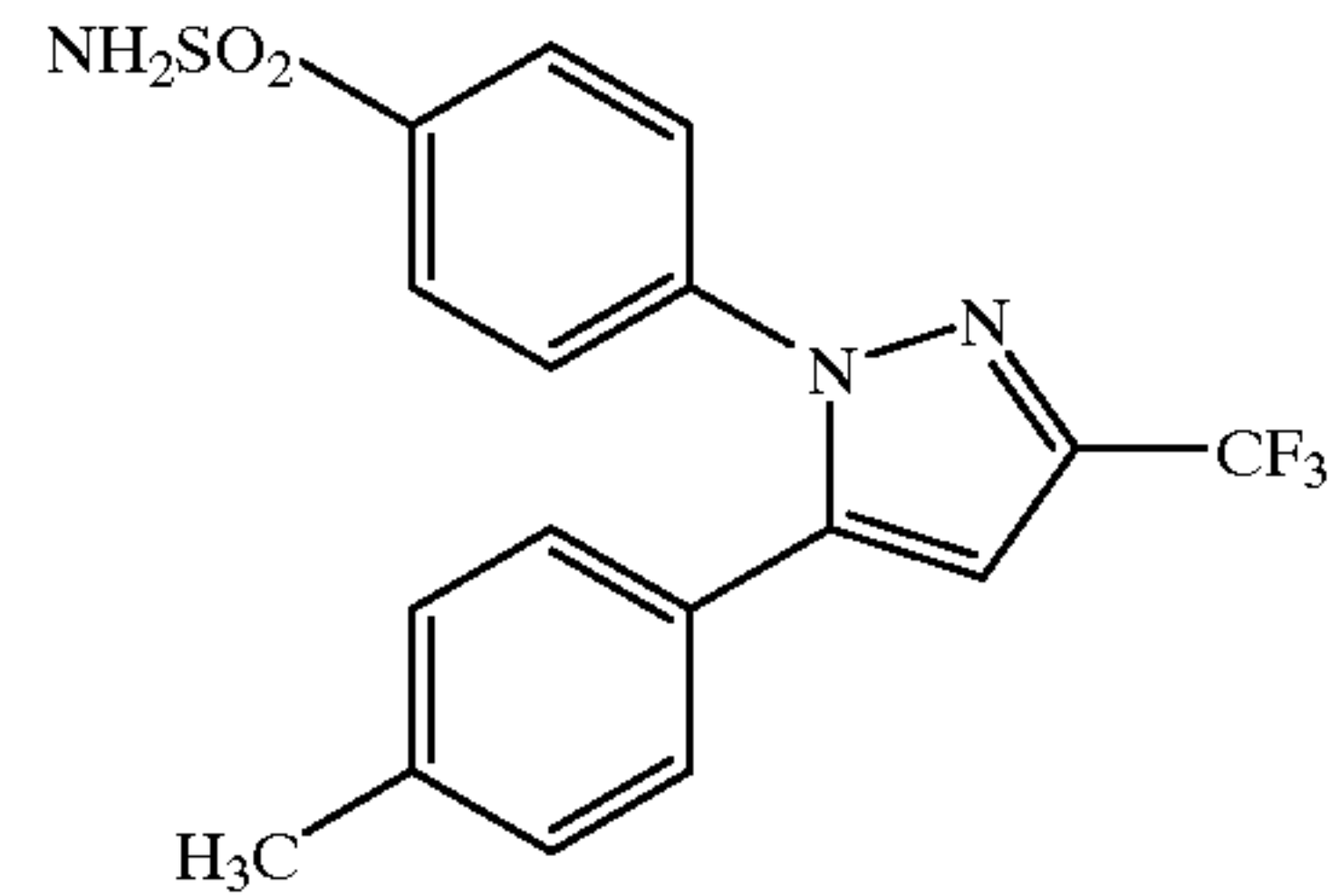
SC-58635
