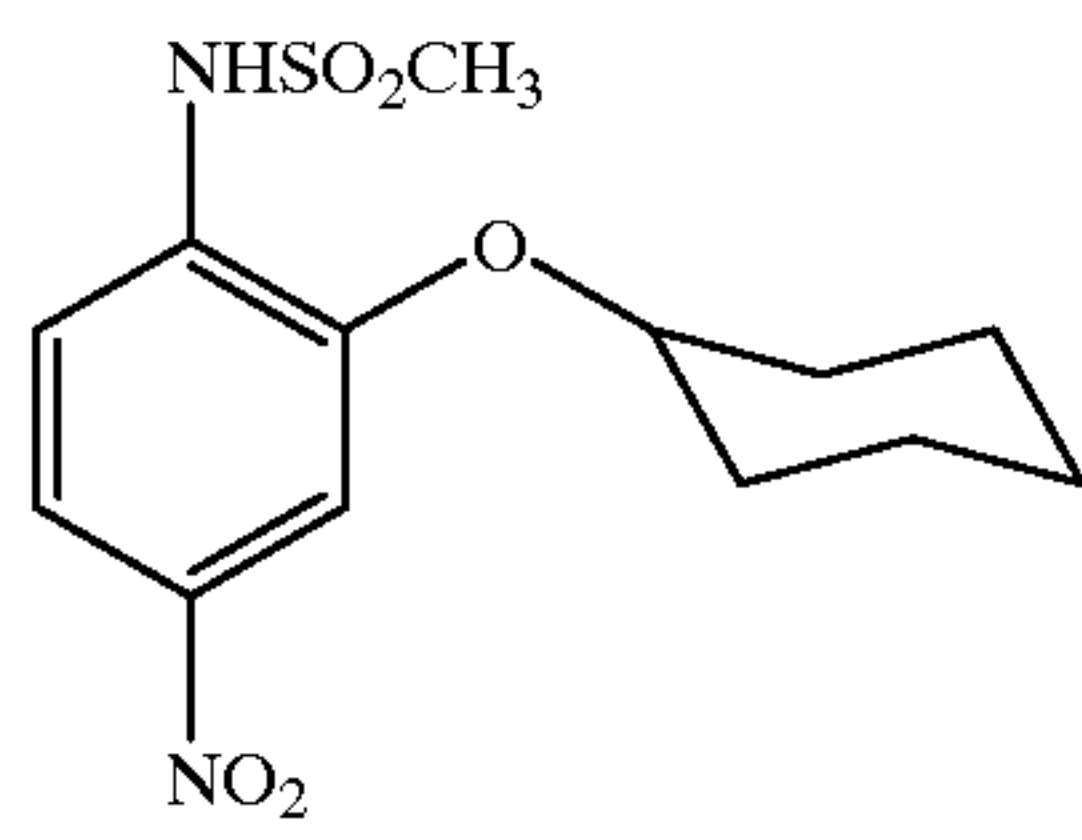
NS-398
