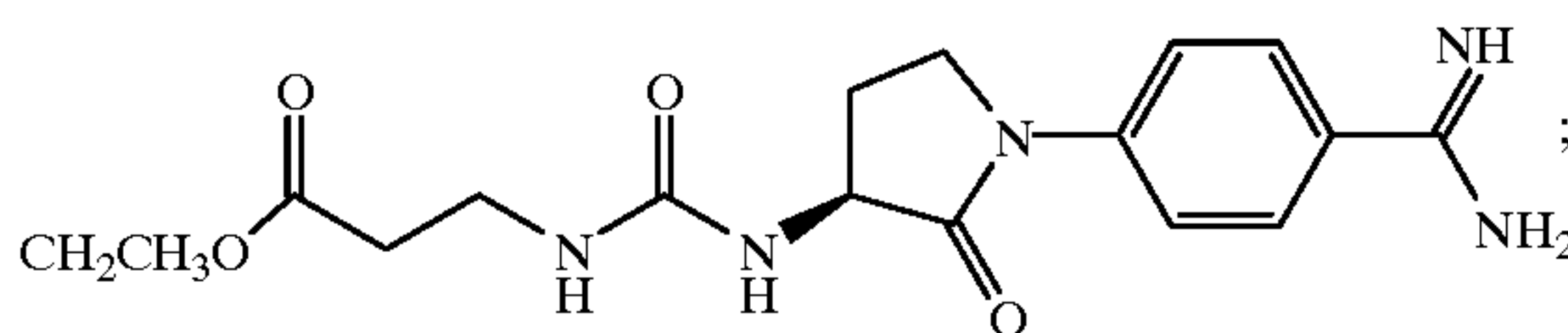
Orbofiban
