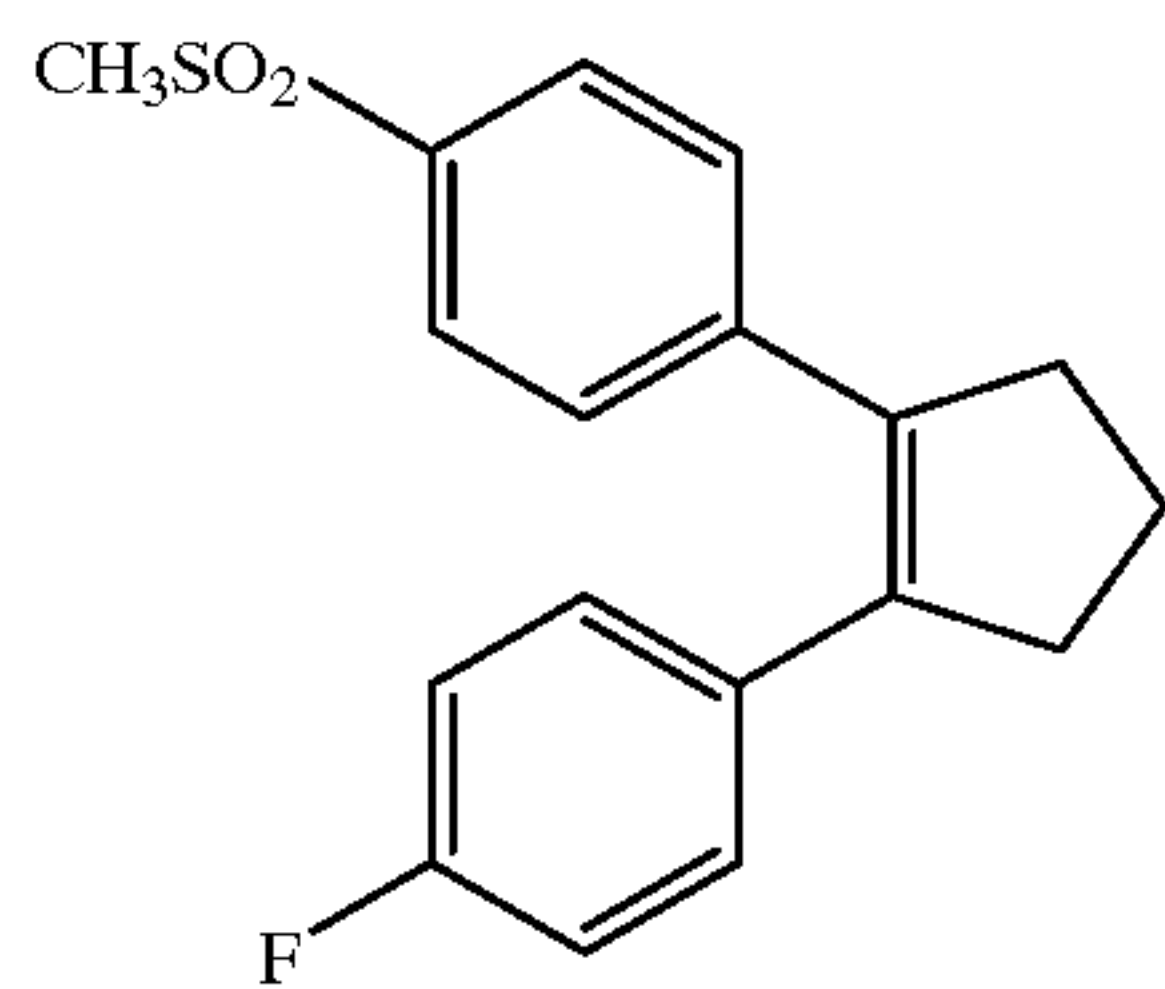
SC-57666
