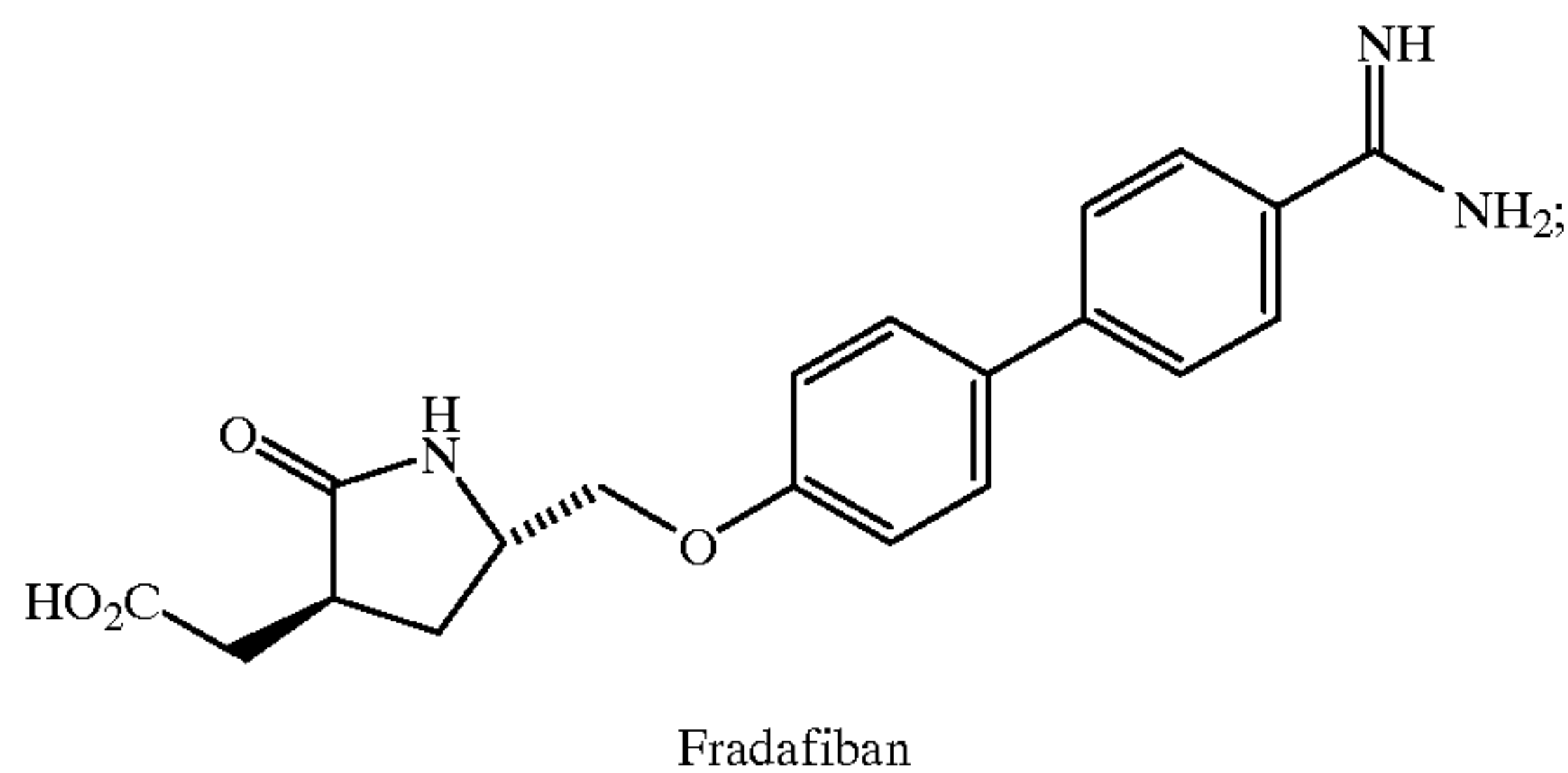
Fradafiban
