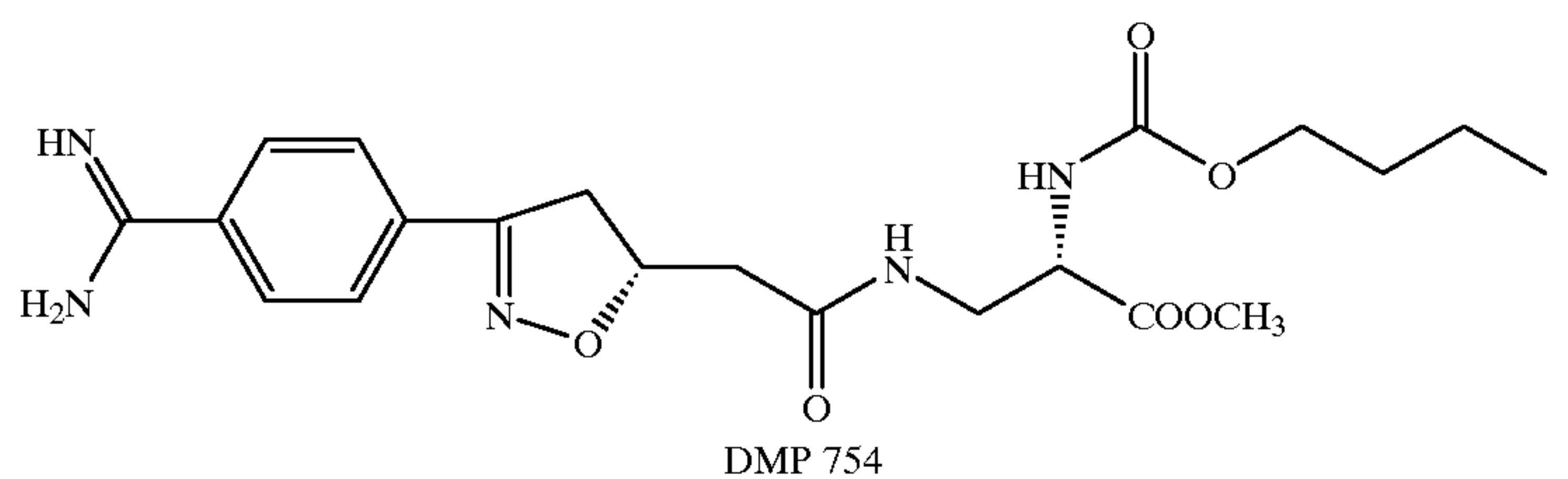
DMP 754
