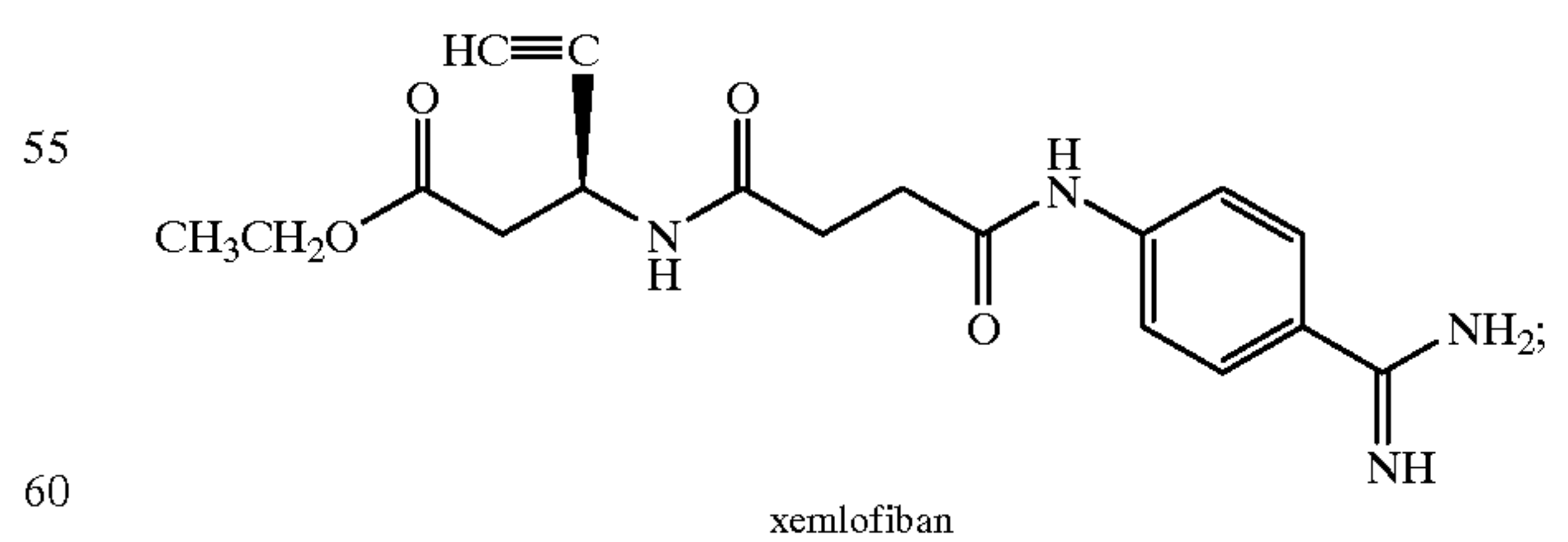
xemlofiban
