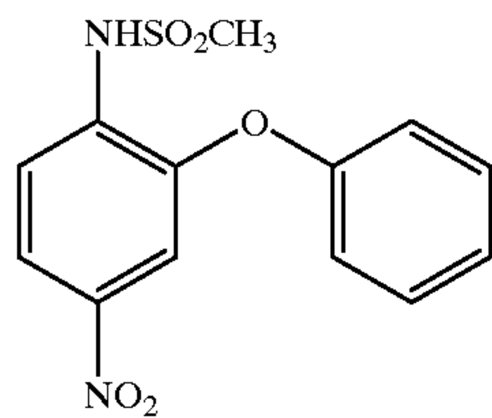
Nimesulide
