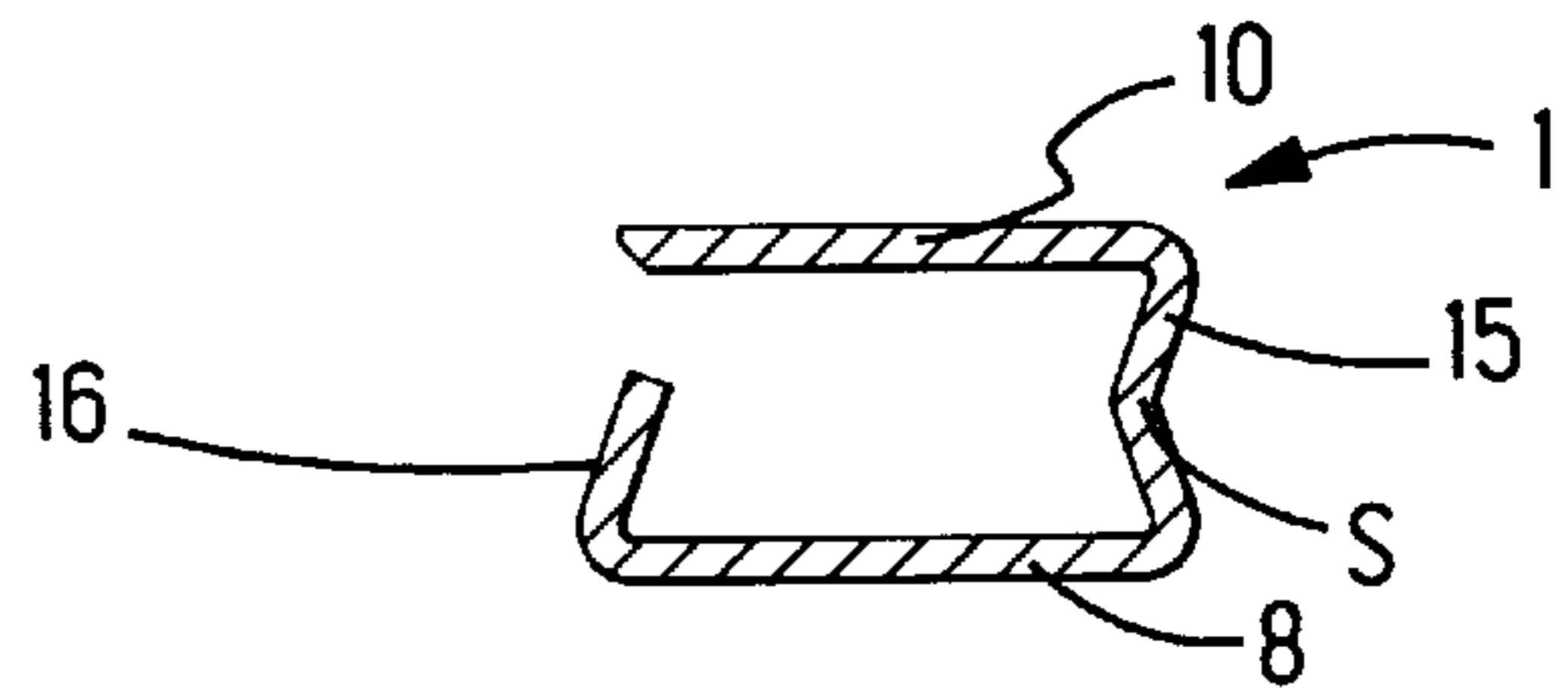
Fig. 7 c-c
