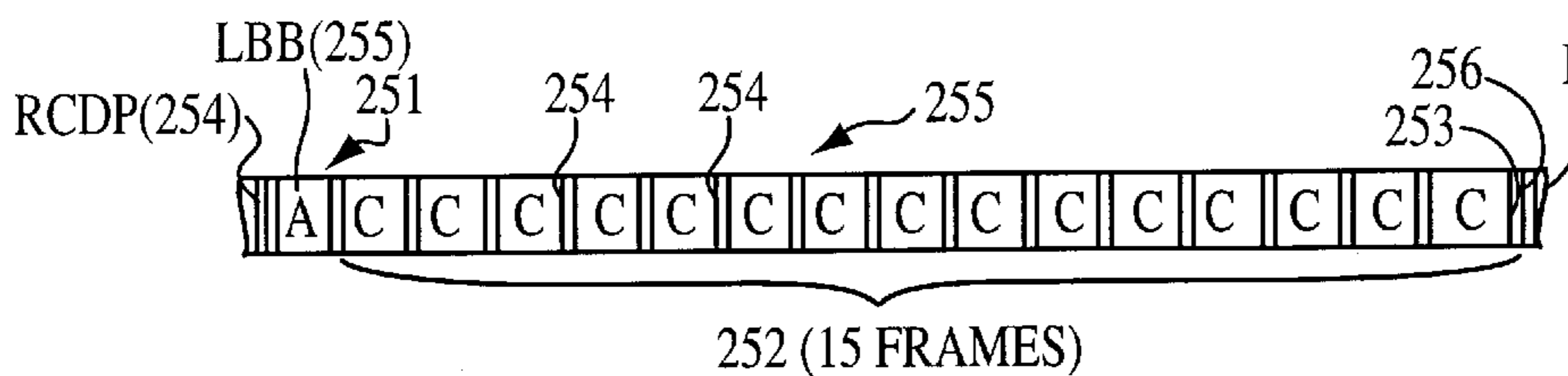
FIG. 6G 2400 BPS
