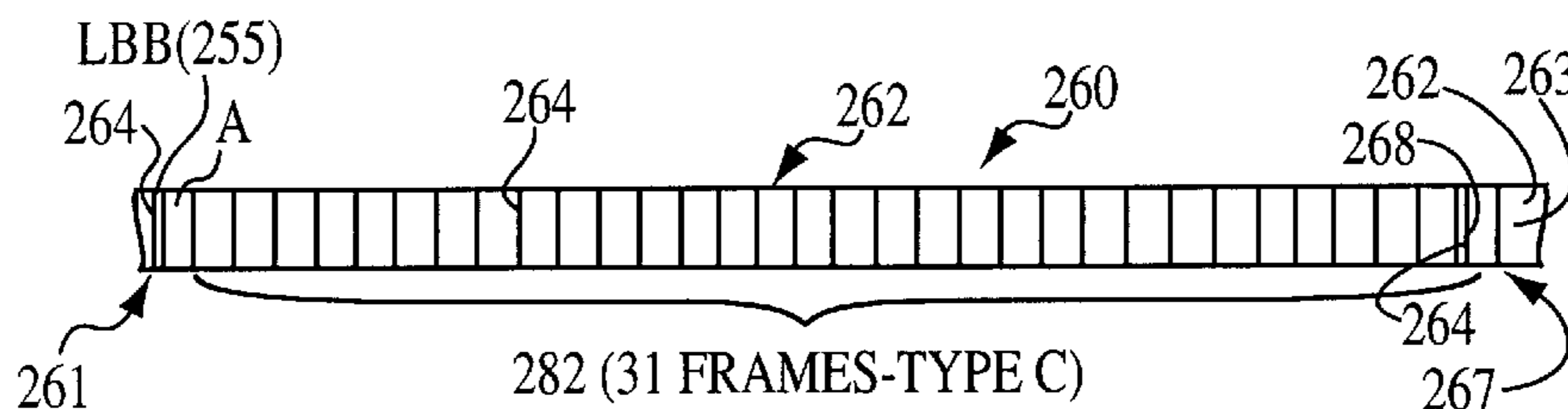
FIG. 6H 4800 BPS
