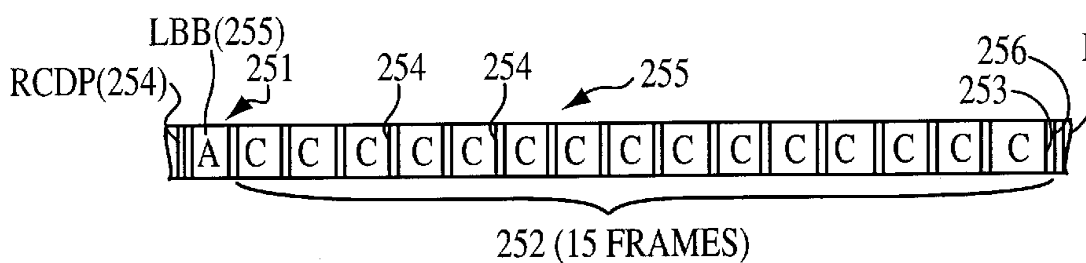
FIG. 6G 2400 BPS
