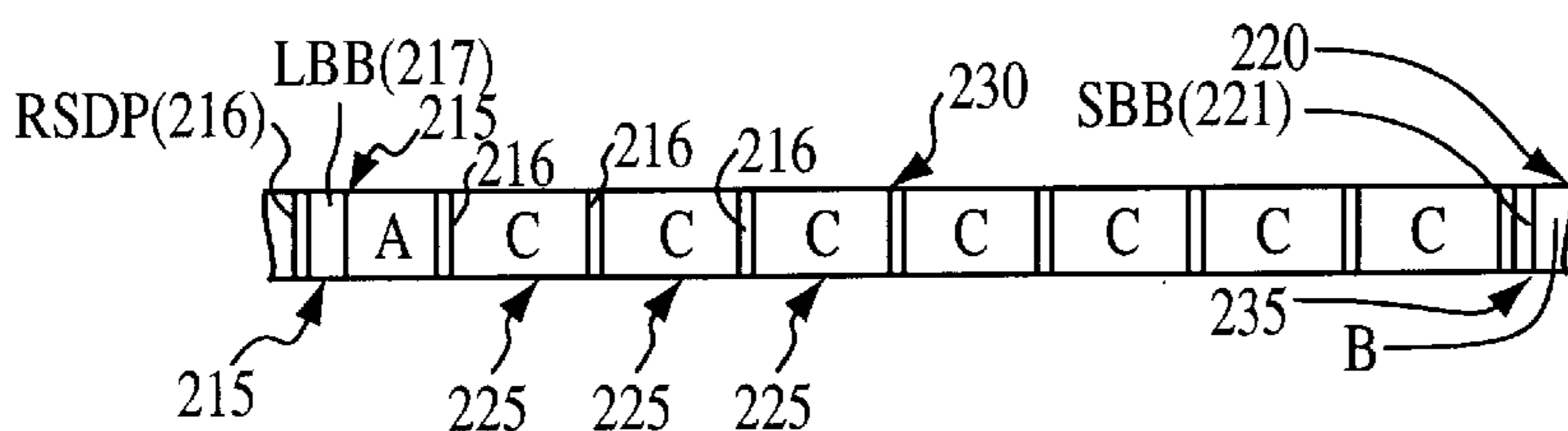
FIG. 6E 600 BPS
