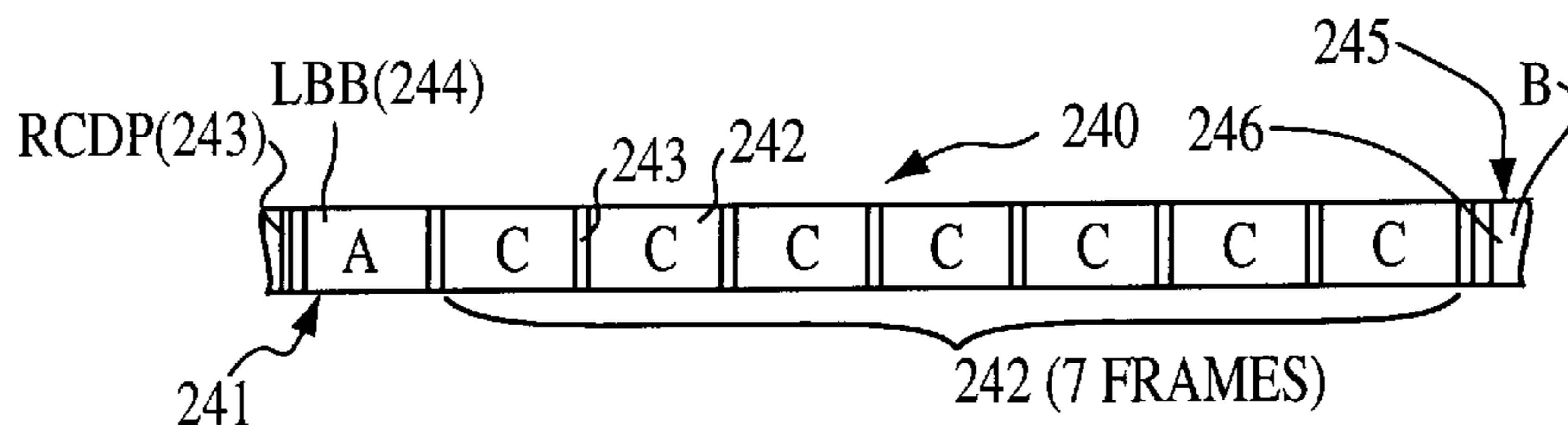
FIG. 6F 1200 BPS
