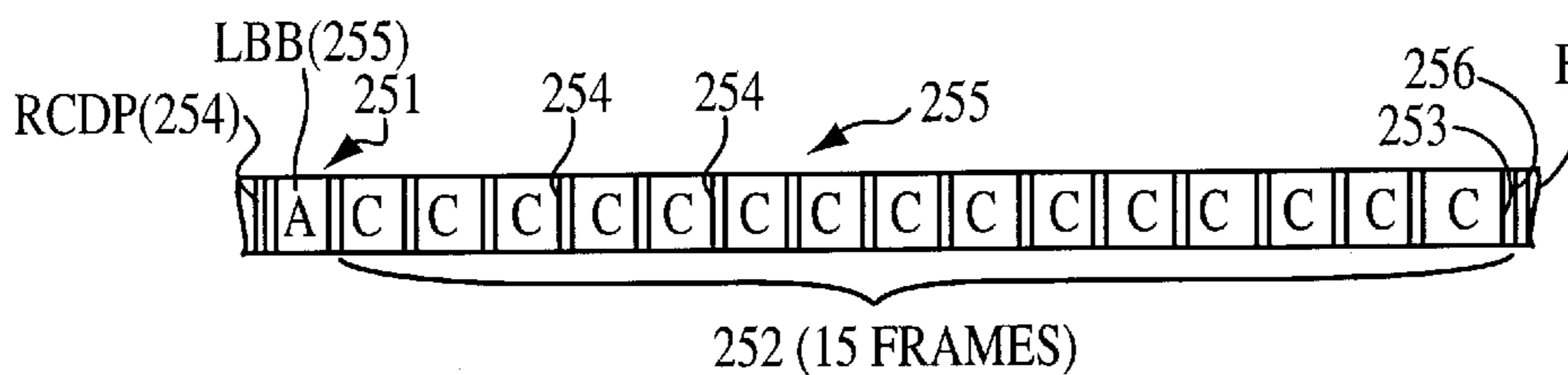
FIG. 6G 2400BPS
