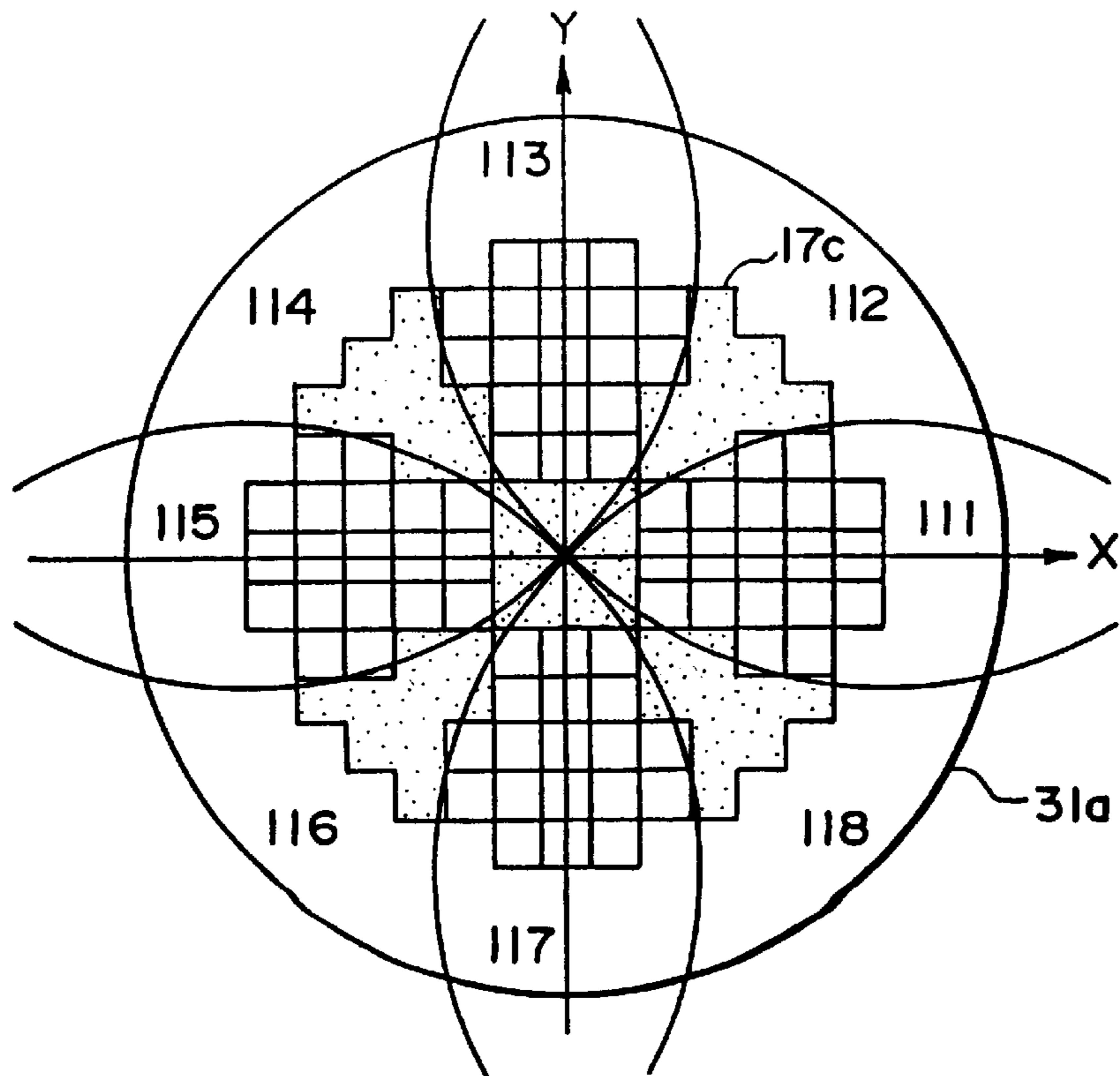
FIG. 15B
