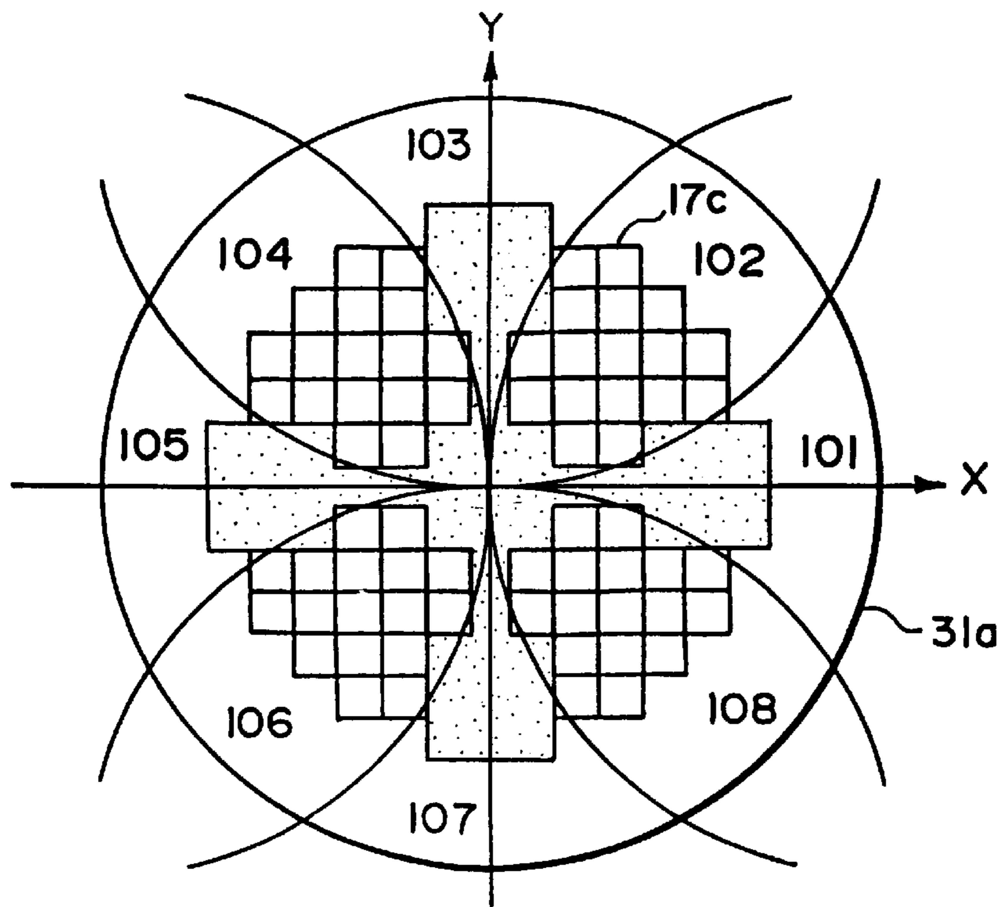
FIG. 15A
