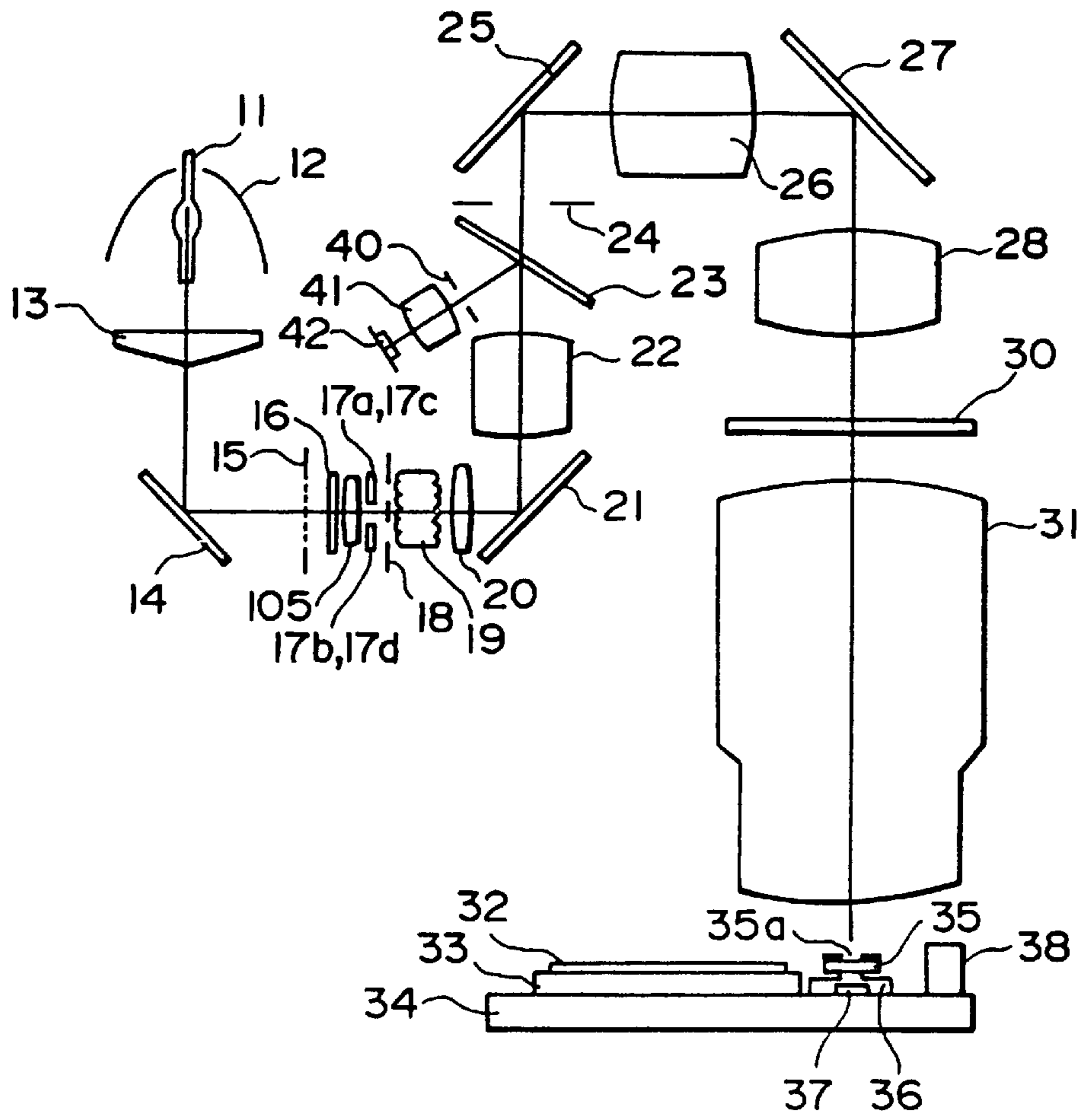
FIG. 6A
